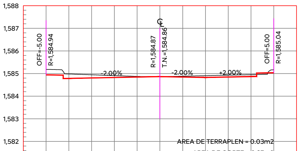
ESTACION 0+280.00 ESCALA HORIZONTAL 1:100 ESCALA VERTICAL 1:100
