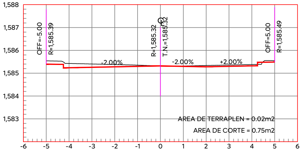
ESTACION 0+240.00 ESCALA HORIZONTAL 1:100 ESCALA VERTICAL 1:100
