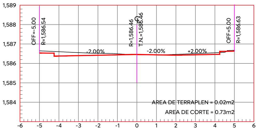
ESTACION 0+200.00 ESCALA HORIZONTAL 1:100 ESCALA VERTICAL 1:100
