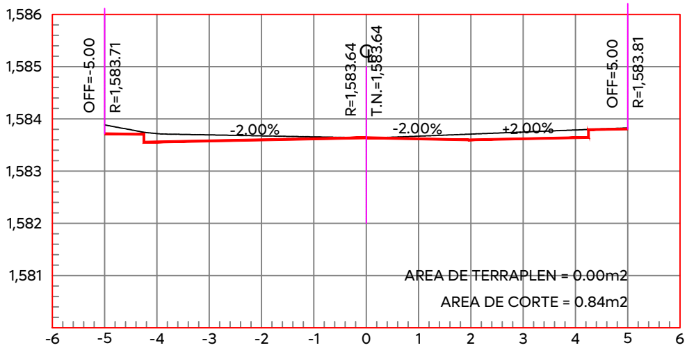
ESTACION 0+360.00 ESCALA HORIZONTAL 1:100 ESCALA VERTICAL 1:100
