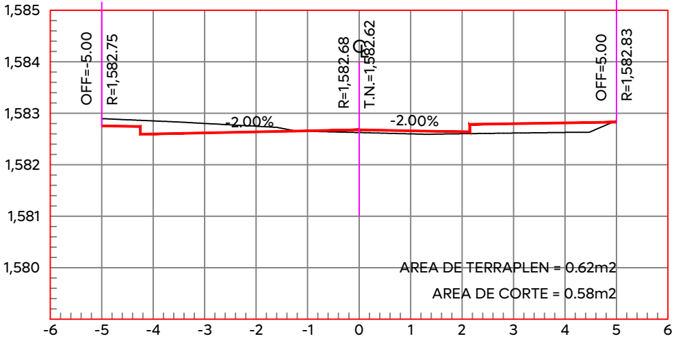
ESTACION 0+420.00 ESCALA HORIZONTAL 1:100 ESCALA VERTICAL 1:100
