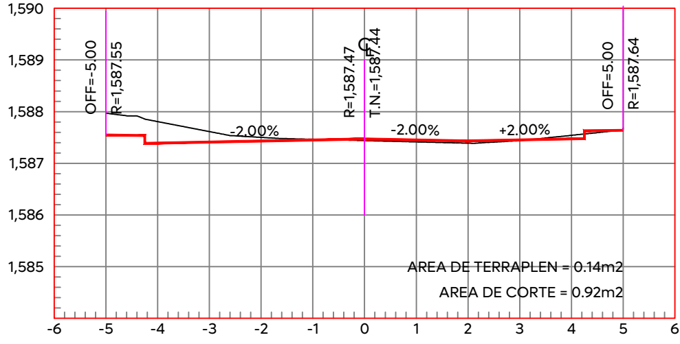
ESTACION 0+140.00 ESCALA HORIZONTAL 1:100 ESCALA VERTICAL 1:100
