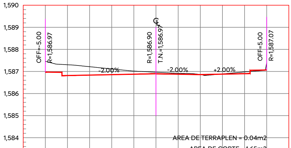
ESTACION 0+180.00 ESCALA HORIZONTAL 1:100 ESCALA VERTICAL 1:100
