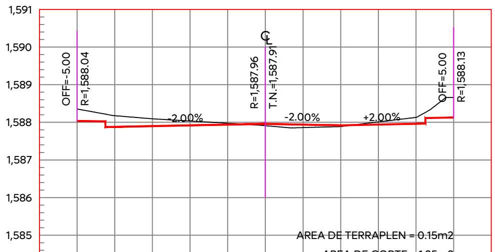
ESTACION 0+100.00 ESCALA HORIZONTAL 1:100 ESCALA VERTICAL 1:100
