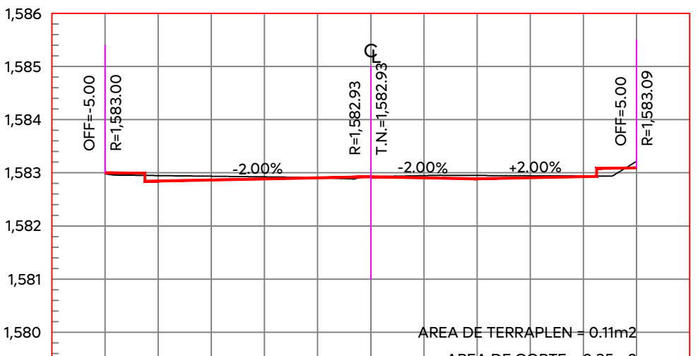
ESTACION 0+400.00 ESCALA HORIZONTAL 1:100 ESCALA VERTICAL 1:100
