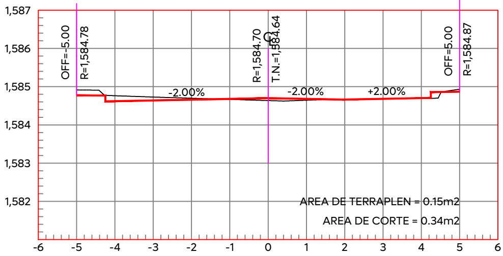
ESTACION 0+300.00 ESCALA HORIZONTAL 1:100 ESCALA VERTICAL 1:100
