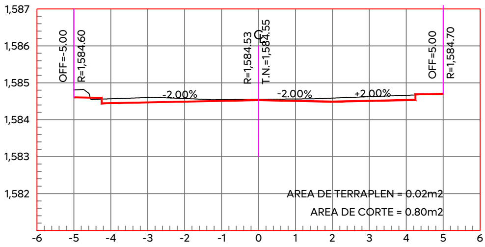
ESTACION 0+320.00 ESCALA HORIZONTAL 1:100 ESCALA VERTICAL 1:100
