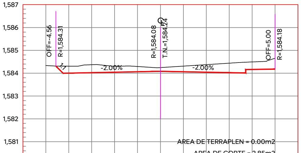
ESTACION 0+340.00 ESCALA HORIZONTAL 1:100 ESCALA VERTICAL 1:100
