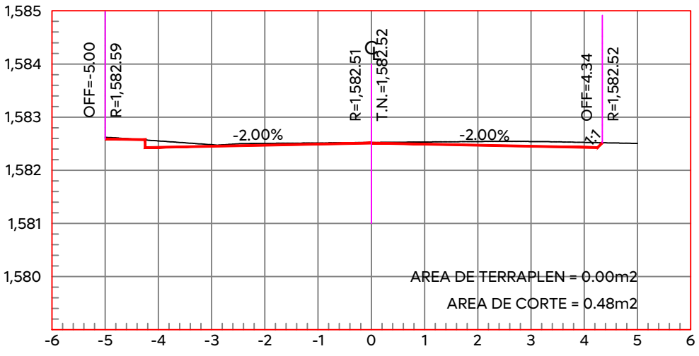
ESTACION 0+433.48 ESCALA HORIZONTAL 1:100 ESCALA VERTICAL 1:100
