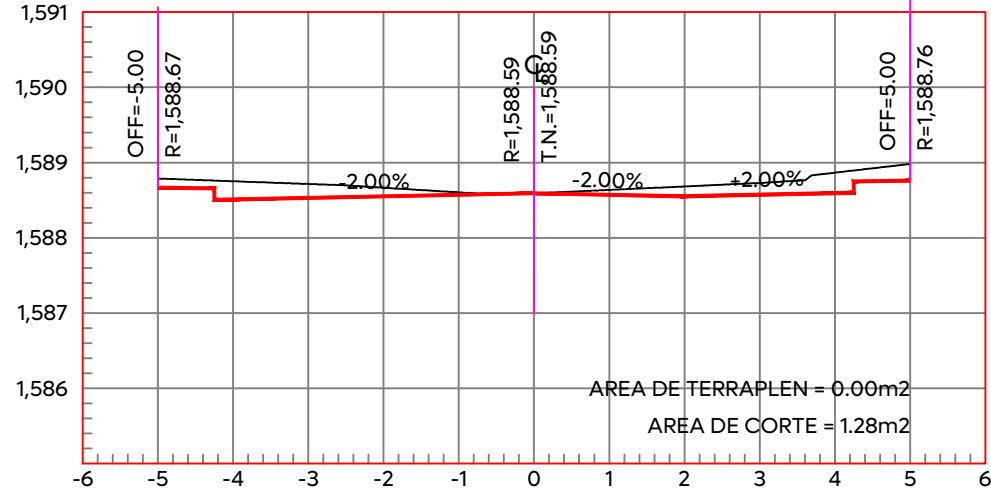
ESTACION 0+040.00 ESCALA HORIZONTAL 1:100 ESCALA VERTICAL 1:100
