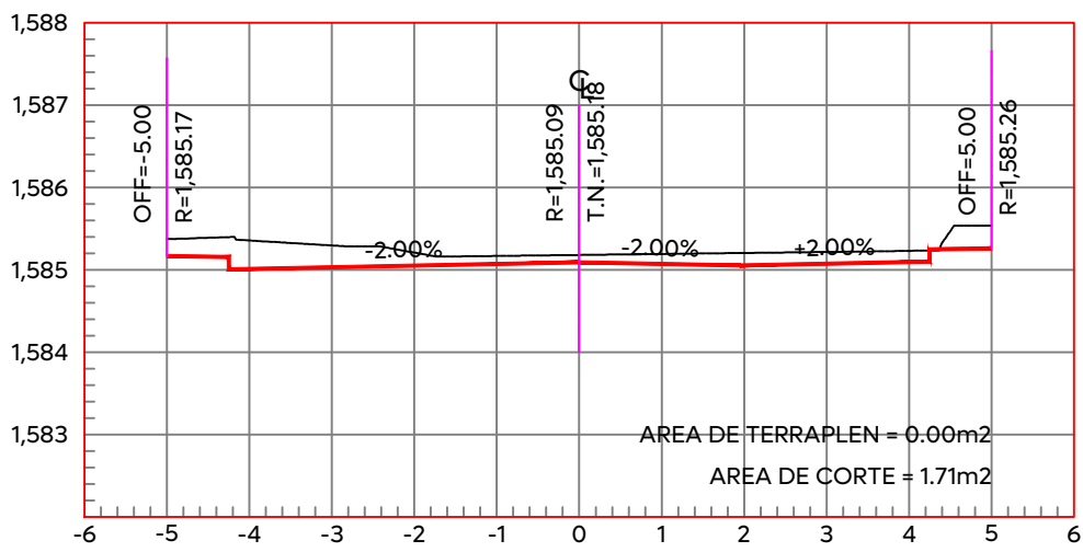
ESTACION 0+260.00 ESCALA HORIZONTAL 1:100 ESCALA VERTICAL 1:100
