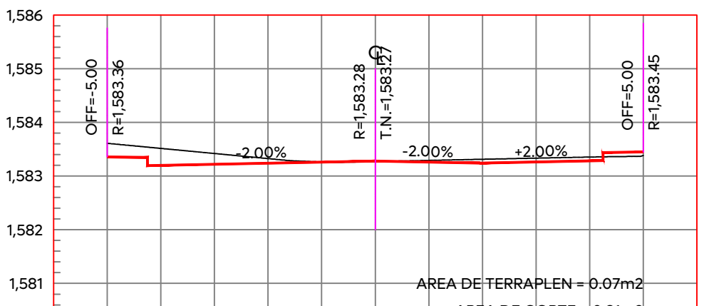
ESTACION 0+380.00 ESCALA HORIZONTAL 1:100 ESCALA VERTICAL 1:100
