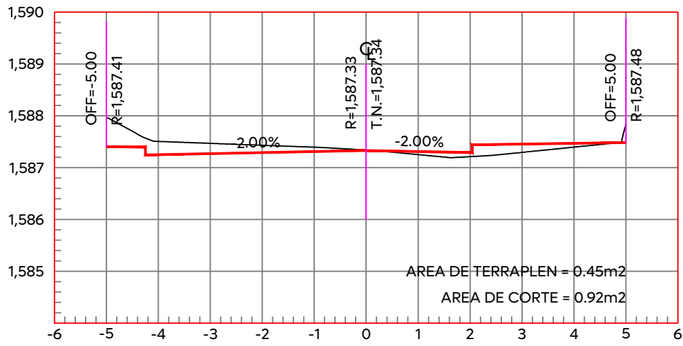
ESTACION 0+160.00 ESCALA HORIZONTAL 1:100 ESCALA VERTICAL 1:100
