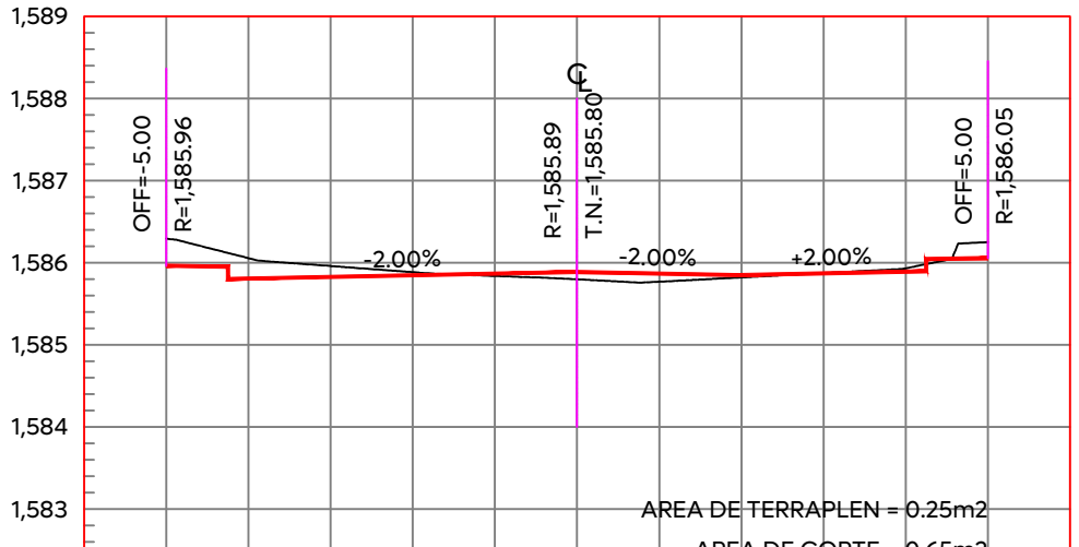
ESTACION 0+220.00 ESCALA HORIZONTAL 1:100 ESCALA VERTICAL 1:100
