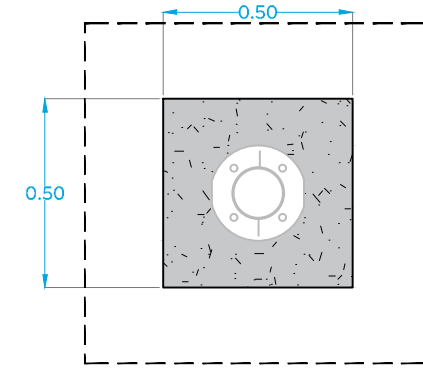
Planta ESC. 1:20
