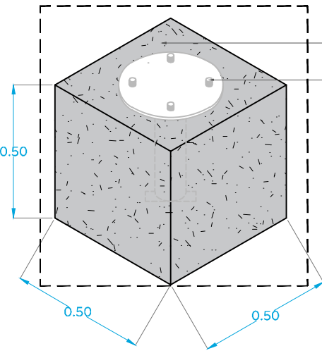
Isométrico ESC. 1:20
