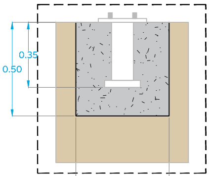
Sección ESC. 1:20
