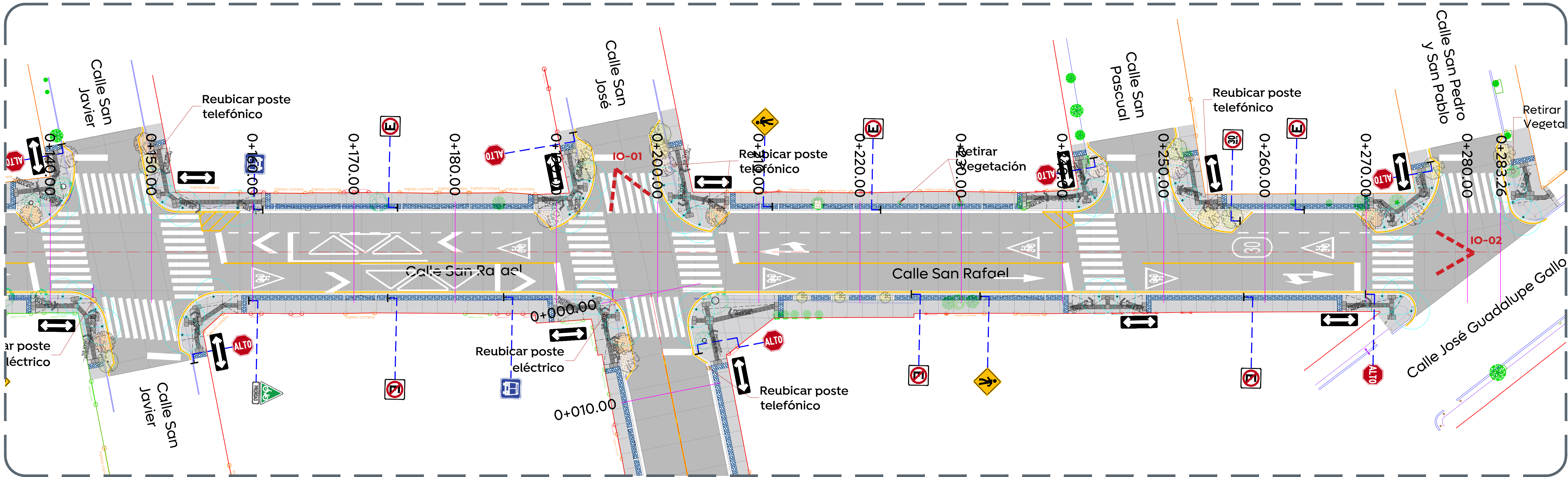
02 Planta arquitectónica Calle San Rafael
