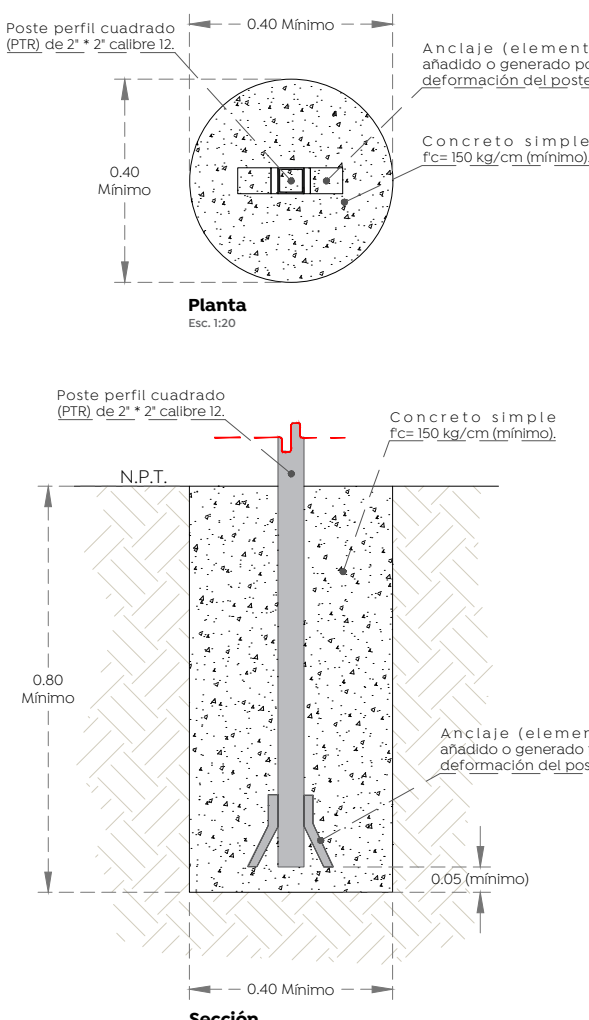
Distancia lateral y Altura de las Señales Verticales en Zona Urbana Escala 1:30
