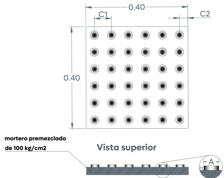
Figura No. 2.1.b. Indicador de advertencia.
