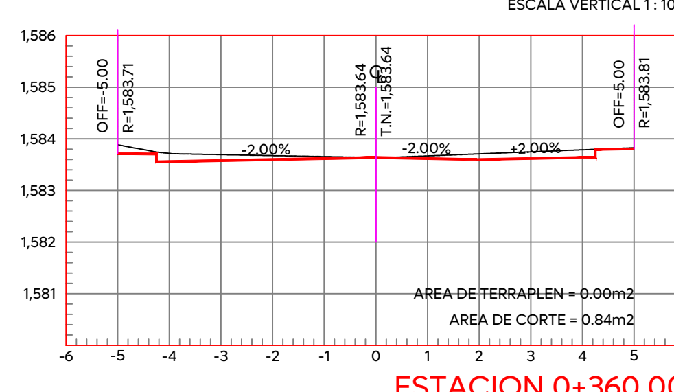
ESTACION 0+360.00 ESCALA HORIZONTAL 1:100 ESCALA VERTICAL 1:100
