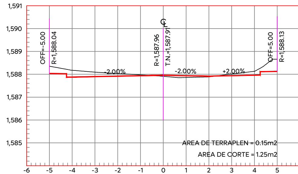
ESTACION 0+100.00 ESCALA HORIZONTAL 1:100 ESCALA VERTICAL 1:100
