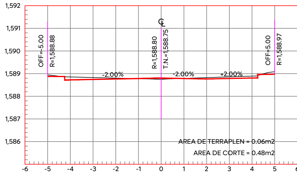
ESTACION 0+020.00 ESCALA HORIZONTAL 1:100 ESCALA VERTICAL 1:100
