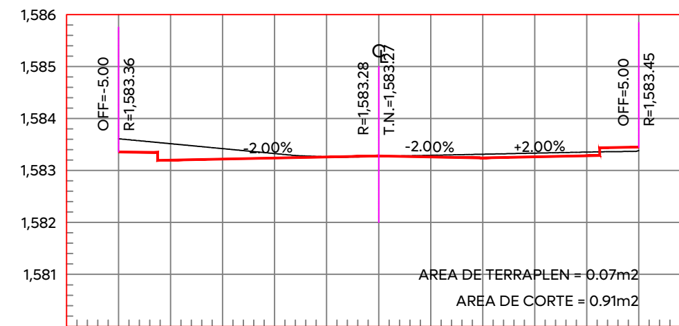
ESTACION 0+380.00 ESCALA HORIZONTAL 1:100 ESCALA VERTICAL 1:100
