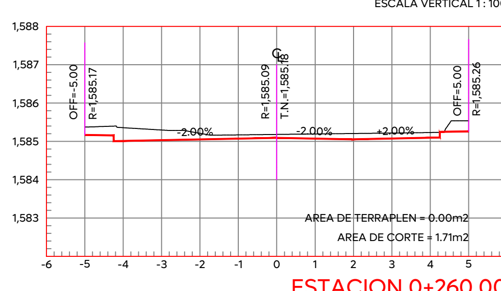
ESTACION 0+260.00 ESCALA HORIZONTAL 1:100 ESCALA VERTICAL 1:100
