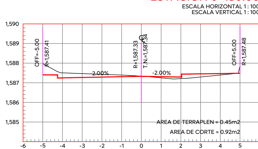
ESTACION 0+160.00 ESCALA HORIZONTAL 1:100 ESCALA VERTICAL 1:100
