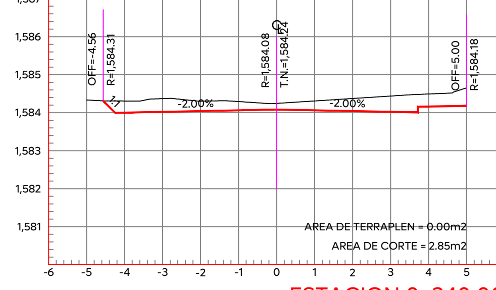
ESTACION 0+340.00 ESCALA HORIZONTAL 1:100 ESCALA VERTICAL 1:100
