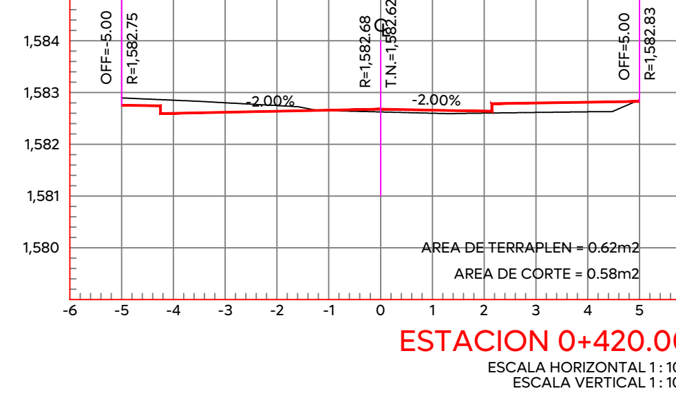
ESTACION 0+420.00 ESCALA HORIZONTAL 1:100 ESCALA VERTICAL 1:100
