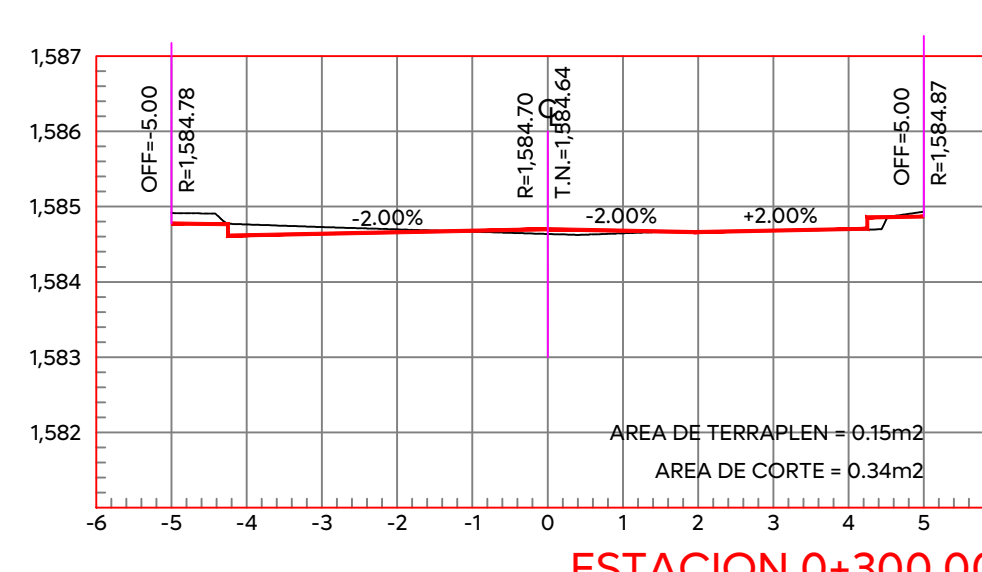
ESTACION 0+300.00 ESCALA HORIZONTAL 1:100 ESCALA VERTICAL 1:100
