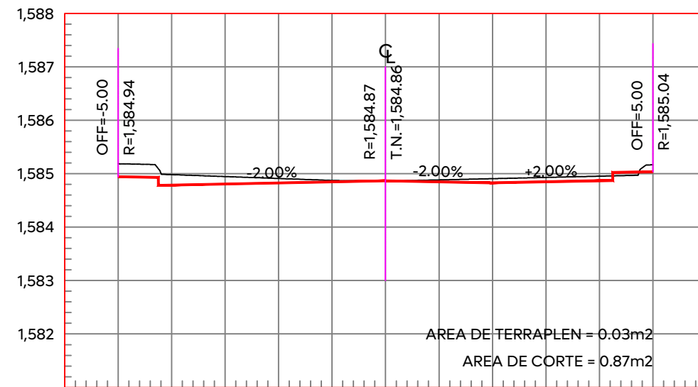
ESTACION 0+280.00 ESCALA HORIZONTAL 1:100 ESCALA VERTICAL 1:100
