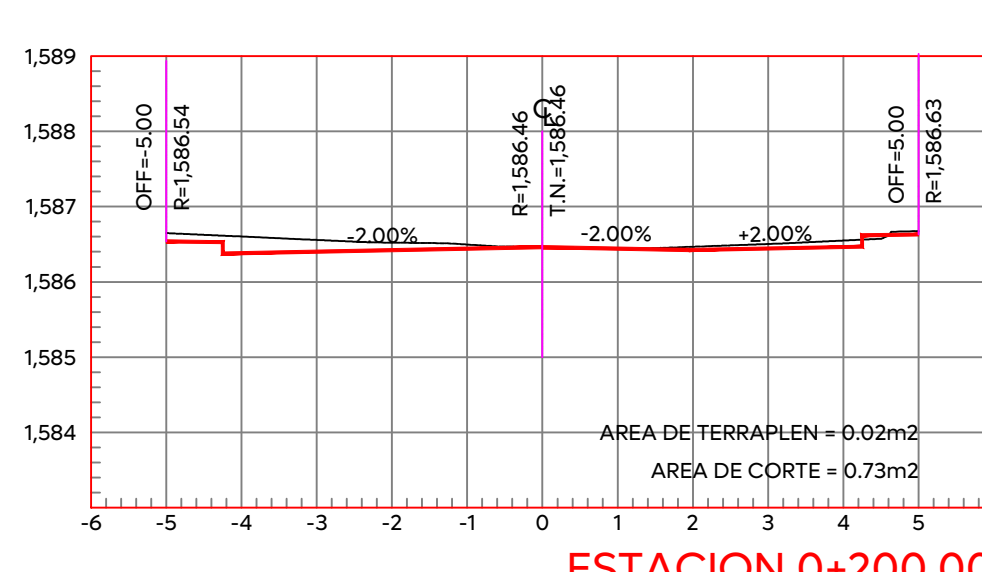
ESTACION 0+200.00 ESCALA HORIZONTAL 1:100 ESCALA VERTICAL 1:100
