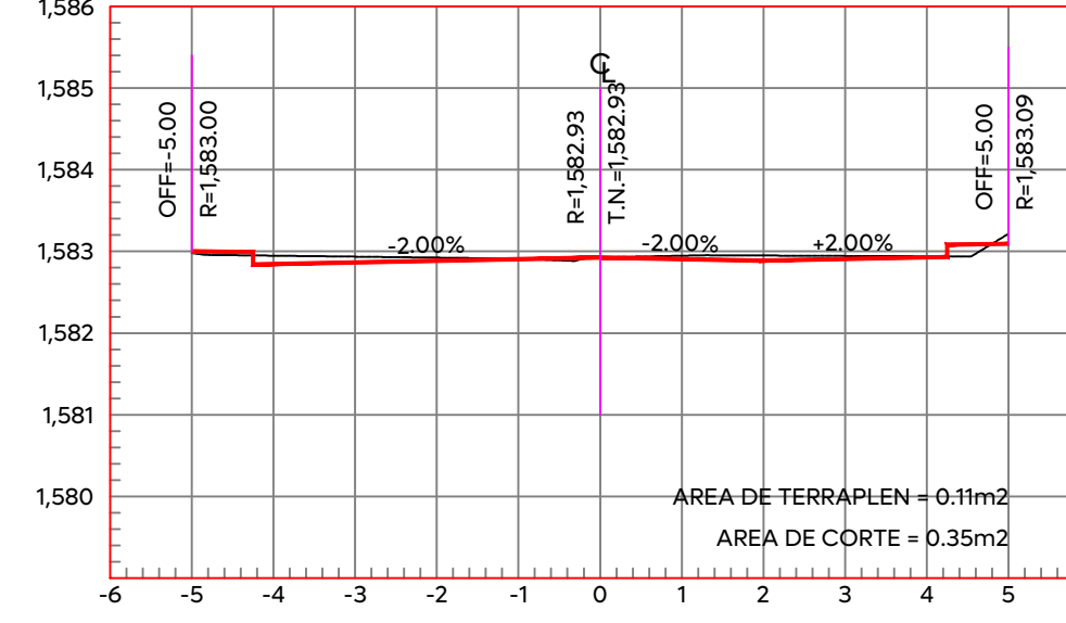
ESTACION 0+400.00 ESCALA HORIZONTAL 1:100 ESCALA VERTICAL 1:100
