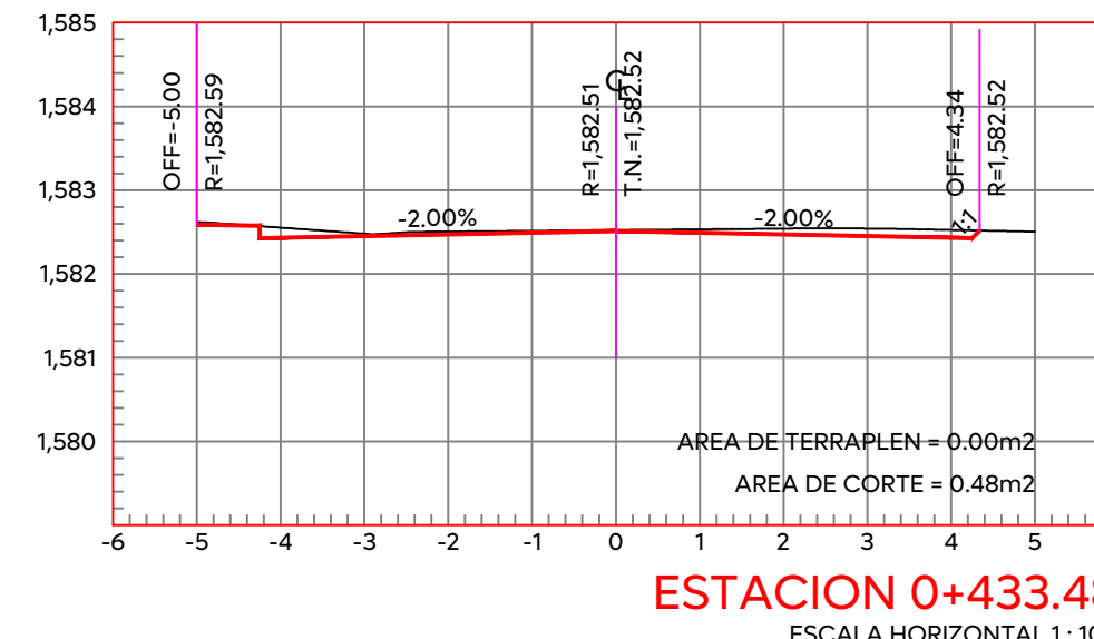
ESTACION 0+433.48 ESCALA HORIZONTAL 1:100 ESCALA VERTICAL 1:100
