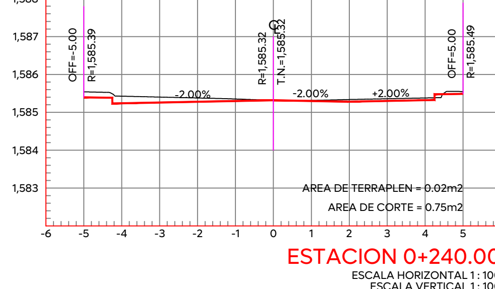
ESTACION 0+240.00 ESCALA HORIZONTAL 1:100 ESCALA VERTICAL 1:100
