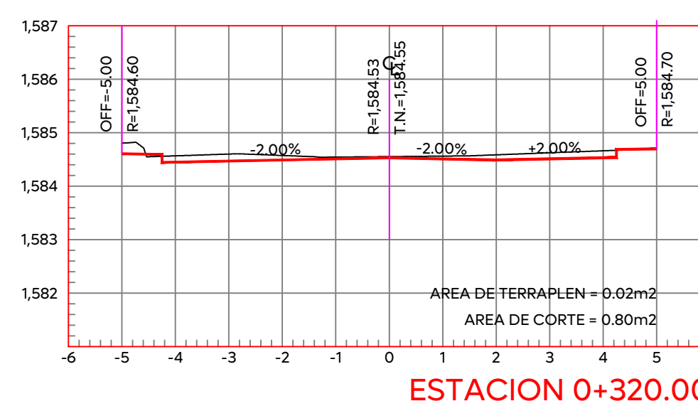
ESTACION 0+320.00 ESCALA HORIZONTAL 1:100 ESCALA VERTICAL 1:100
