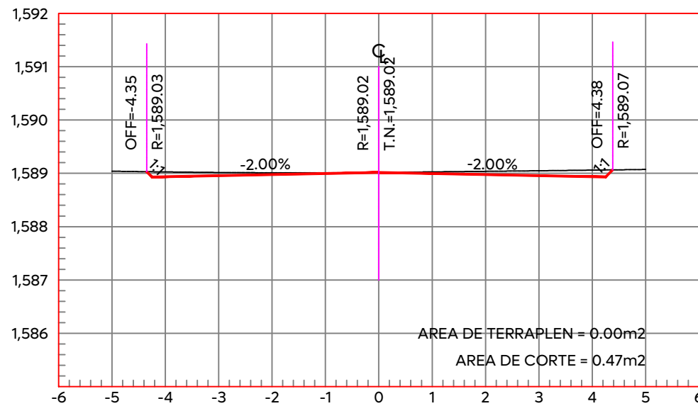
ESTACION 0+000.00 ESCALA HORIZONTAL 1:100 ESCALA VERTICAL 1:100
