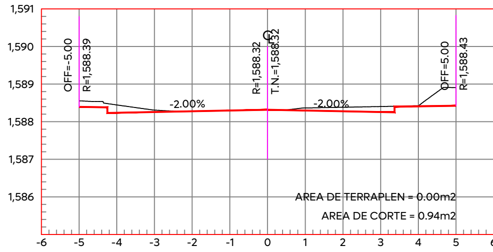
ESTACION 0+080.00 ESCALA HORIZONTAL 1:100 ESCALA VERTICAL 1:100
