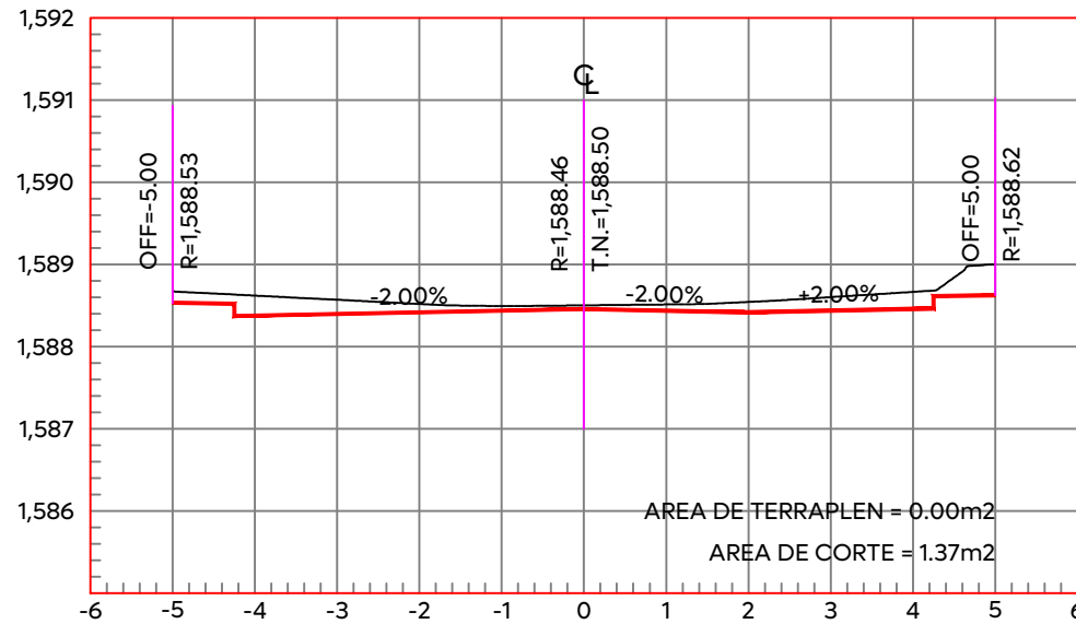
ESTACION 0+060.00 ESCALA HORIZONTAL 1:100 ESCALA VERTICAL 1:100
