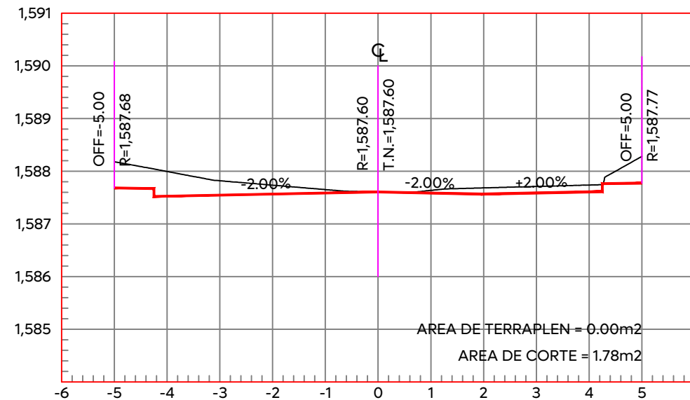
ESTACION 0+120.00 ESCALA HORIZONTAL 1:100 ESCALA VERTICAL 1:100
