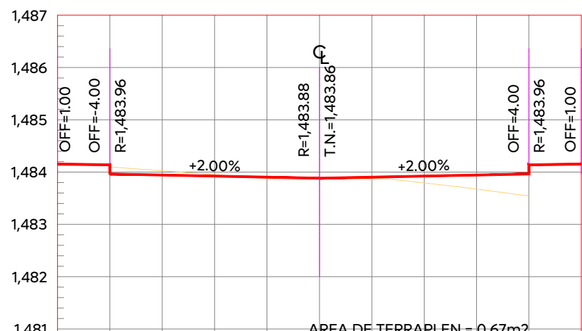
ESTACION 0+168.64 ESCALA HORIZONTAL 1:100 ESCALA VERTICAL 1:100
