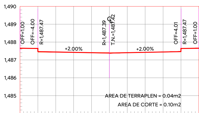
ESTACION 0+040.00 ESCALA HORIZONTAL 1:100 ESCALA VERTICAL 1:100
