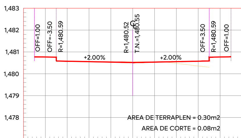
ESTACION 0+120.00 ESCALA HORIZONTAL 1:100 ESCALA VERTICAL 1:100
