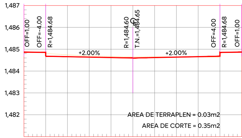
ESTACION 0+180.00 ESCALA HORIZONTAL 1:100 ESCALA VERTICAL 1:100
