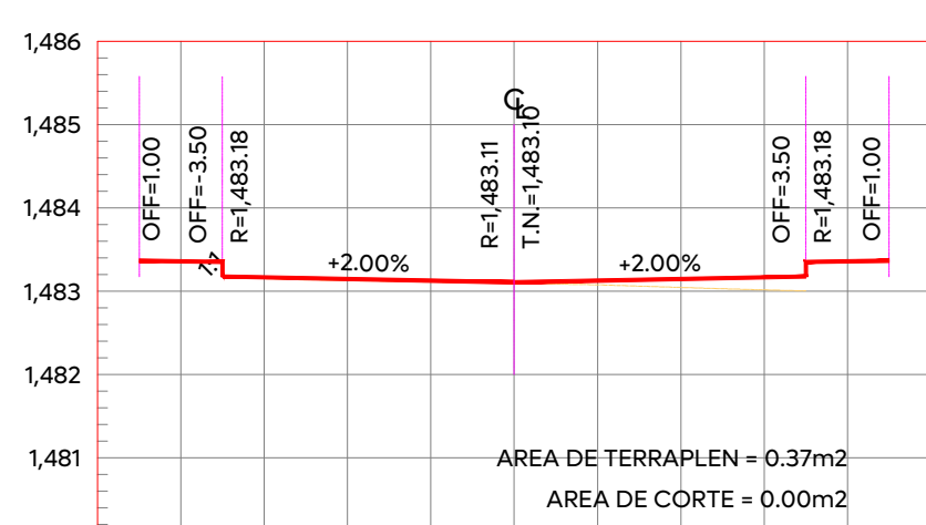
ESTACION 0+160.00 ESCALA HORIZONTAL 1:100 ESCALA VERTICAL 1:100
