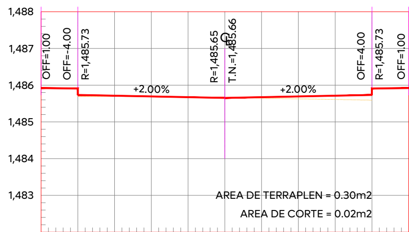
ESTACION 0+054.87 ESCALA HORIZONTAL 1:100 ESCALA VERTICAL 1:100
