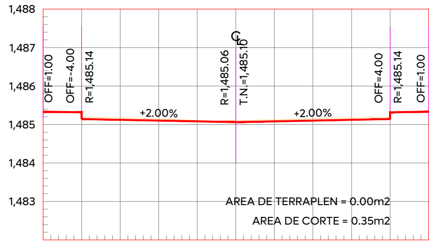
ESTACION 0+060.00 ESCALA HORIZONTAL 1:100 ESCALA VERTICAL 1:100
