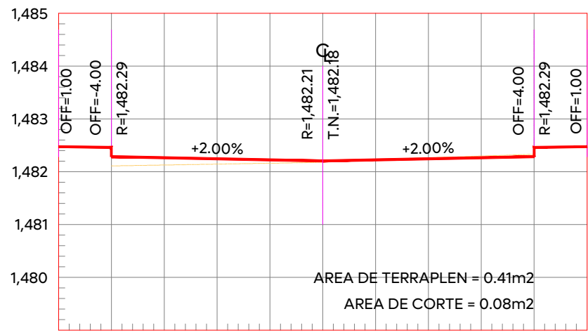
ESTACION 0+080.00 ESCALA HORIZONTAL 1:100 ESCALA VERTICAL 1:100
