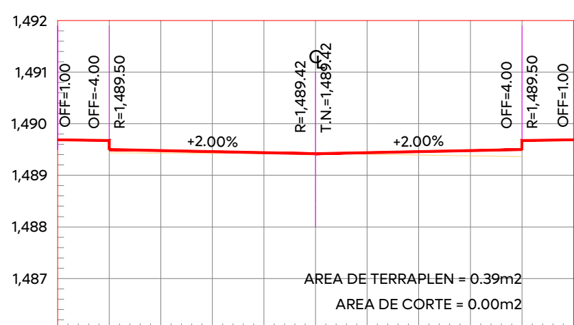
ESTACION 0+000.00 ESCALA HORIZONTAL 1:100 ESCALA VERTICAL 1:100
