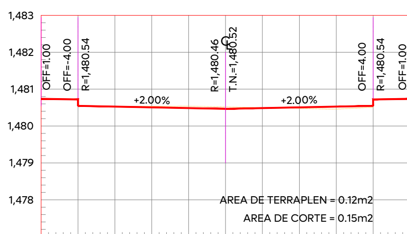
ESTACION 0+107.11 ESCALA HORIZONTAL 1:100 ESCALA VERTICAL 1:100
