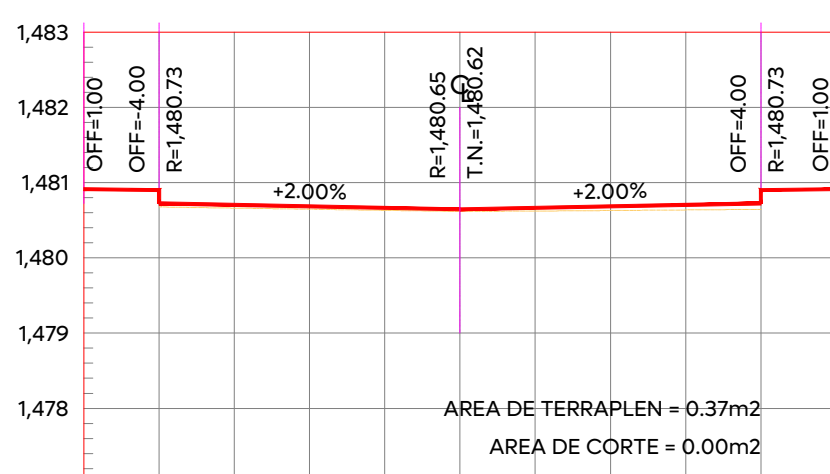
ESTACION 0+100.00 ESCALA HORIZONTAL 1:100 ESCALA VERTICAL 1:100
