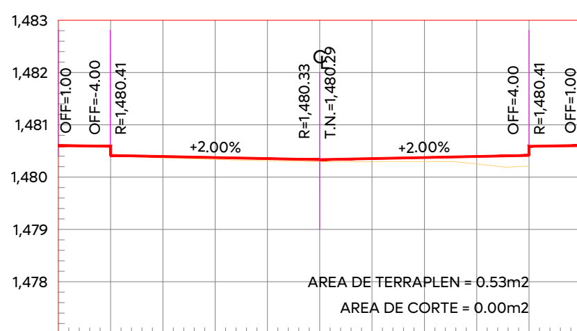
ESTACION 0+114.83 ESCALA HORIZONTAL 1:100 ESCALA VERTICAL 1:100
