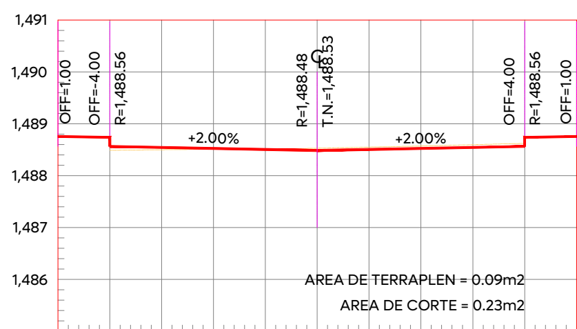
ESTACION 0+020.00 ESCALA HORIZONTAL 1:100 ESCALA VERTICAL 1:100
