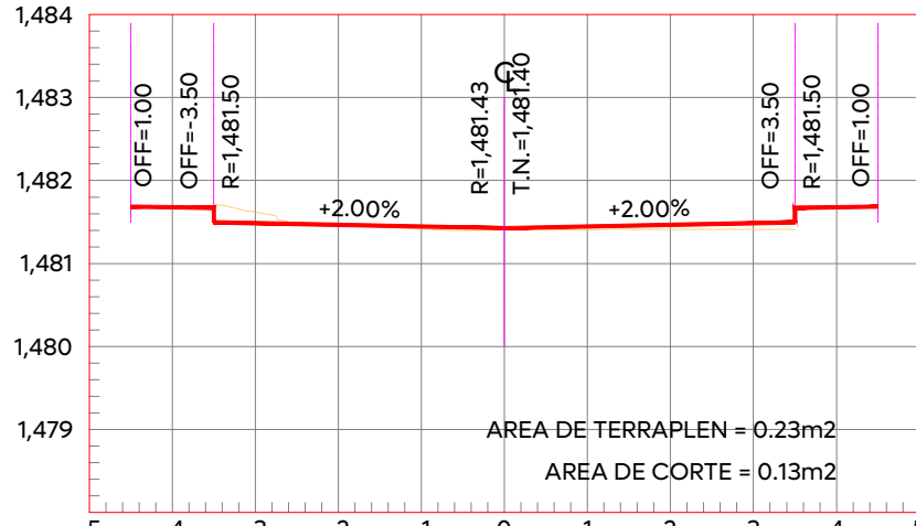
ESTACION 0+140.00 ESCALA HORIZONTAL 1:100 ESCALA VERTICAL 1:100
