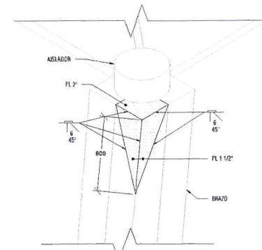
5 DETALLE DE CONEXIÓN EN ESQUINA ESC, S/E (cm)
