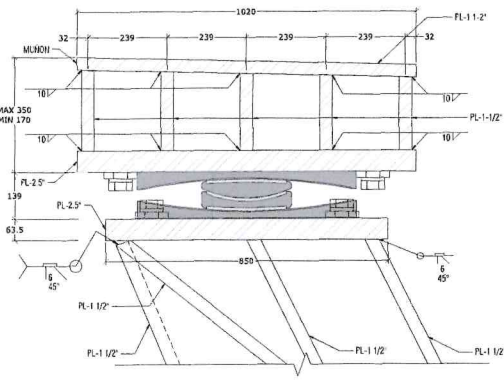
F SECCIÓN 1:10 [mm]
