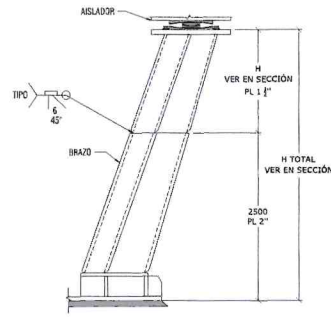
2 CONEXIÓN EN CAMBIO DE PLACA 1:50 [mm]
