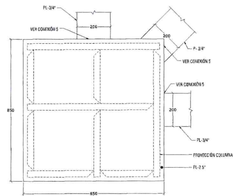
6 DETALLE DE UNIÓN TENSOR A COLUMNA 1:10 (mm)
