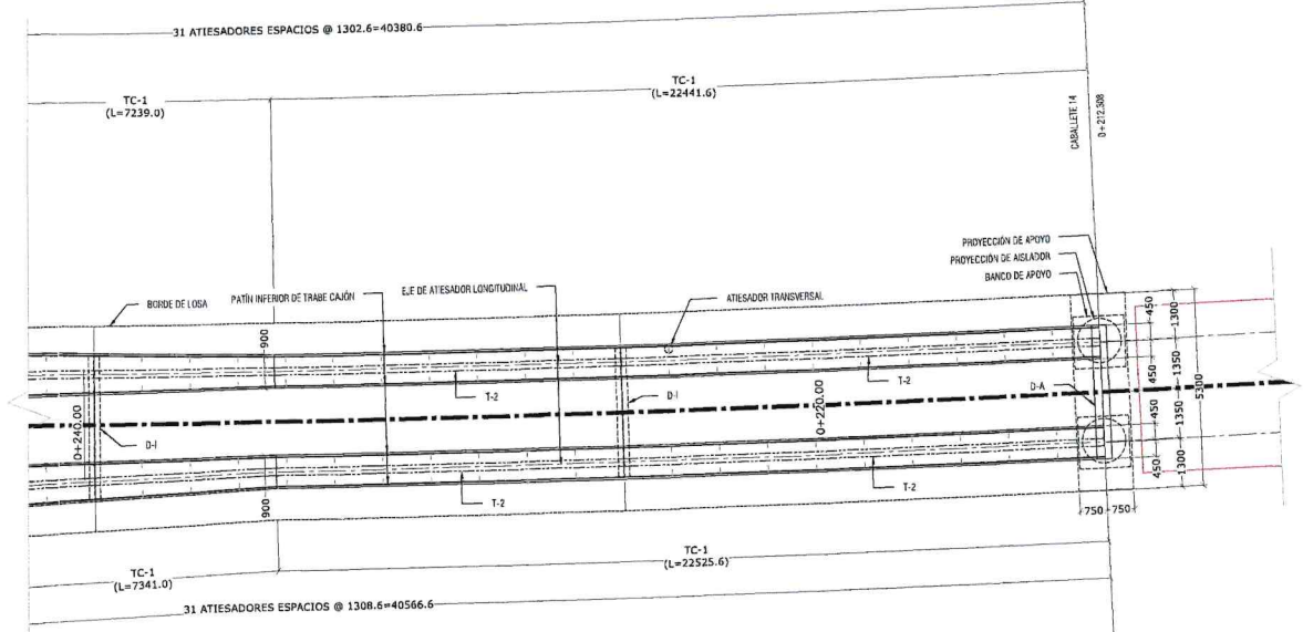
2 PLANTA LECHO INFERIOR DE TRABE CAJÓN (6-6)
