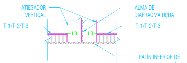
SECCIÓN TIPO (INTERSECCIÓN ENTRE ATIESADOR LONGITUDINAL CON ATIESADOR VERTICAL)
