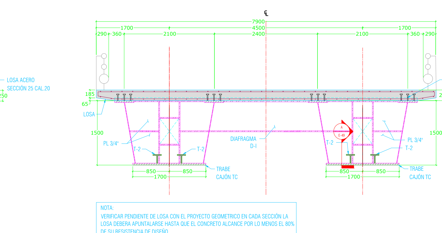
SECCIÓN DE DIAFRAGMA INTERMEDIOS D-I PARA LOSA DE ANCHO DE 7900
