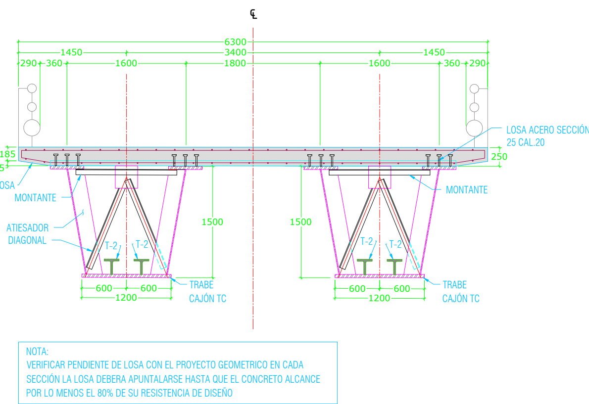
SECCIÓN TIPO DE ARRIOSTRAMIENTO LATERAL Y HORIZONTAL (@ MONTANTE EN PLANTA) PARA LOSA DE ANCHO DE 6300
