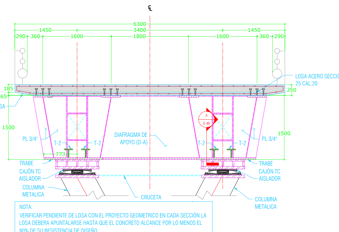
SECCIÓN DE DIAFRAGMA DE APOYO D-A PARA LOSA DE ANCHO DE 6300
