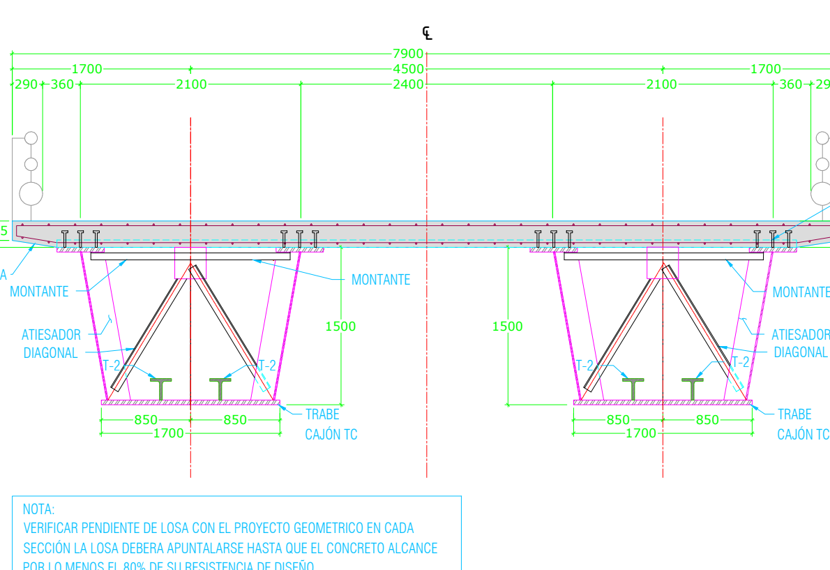
SECCIÓN TIPO DE ARRIOSTRAMIENTO LATERAL Y HORIZONTAL (@ MONTANTE EN PLANTA) PARA LOSA DE ANCHO DE 7900
