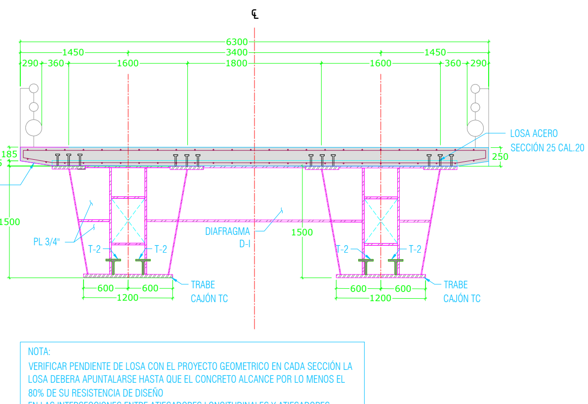
SECCIÓN DE DIAFRAGMA INTERMEDIOS D-I PARA LOSA DE ANCHO DE 6300
