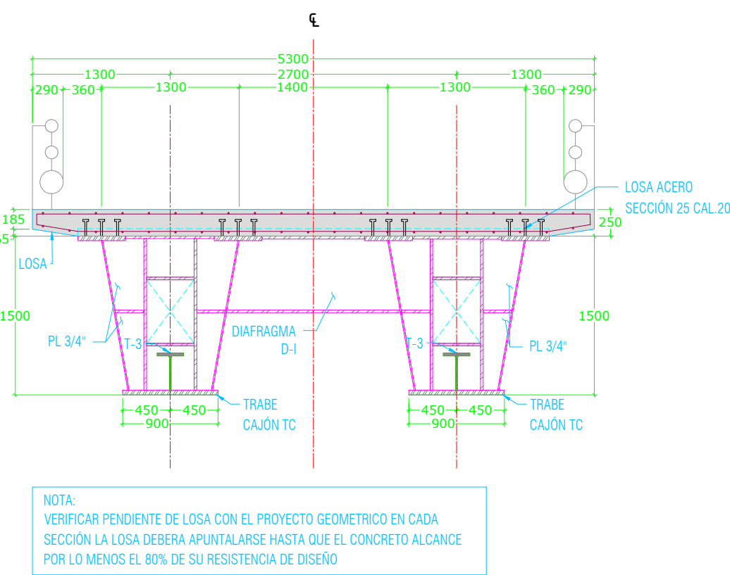
SECCIÓN DE DIAFRAGMA INTERMEDIOS D-I PARA LOSA DE ANCHO DE 5300
