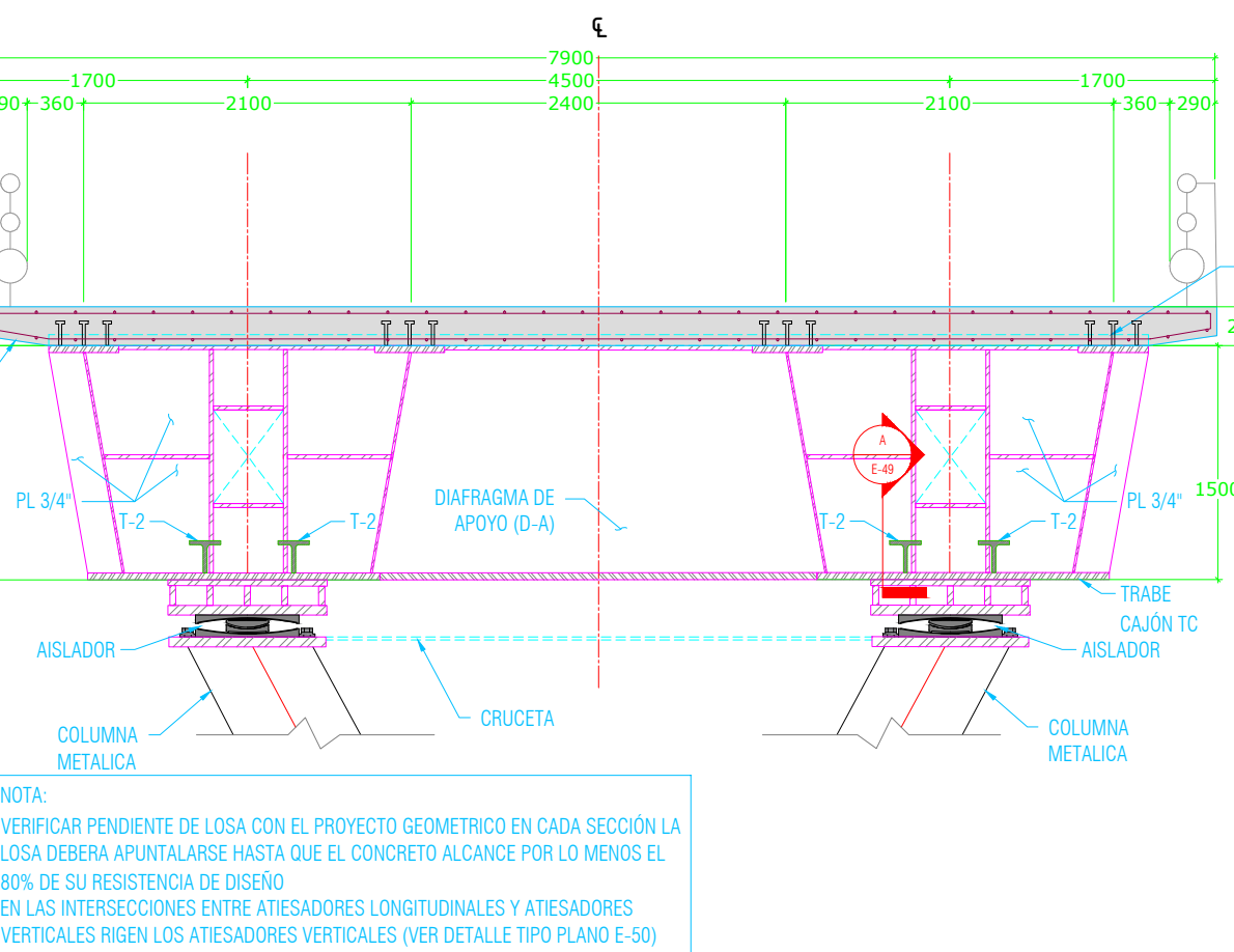
SECCIÓN DE DIAFRAGMA DE APOYO D-A PARA LOSA DE ANCHO DE 7900
