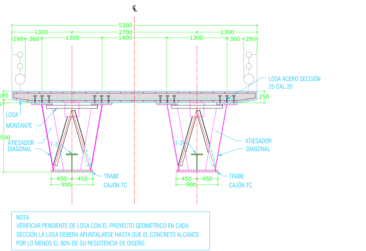
SECCIÓN TIPO DE ARRIOSTRAMIENTO LATERAL Y HORIZONTAL (@ MONTANTE EN PLANTA) PARA LOSA DE ANCHO 5300
