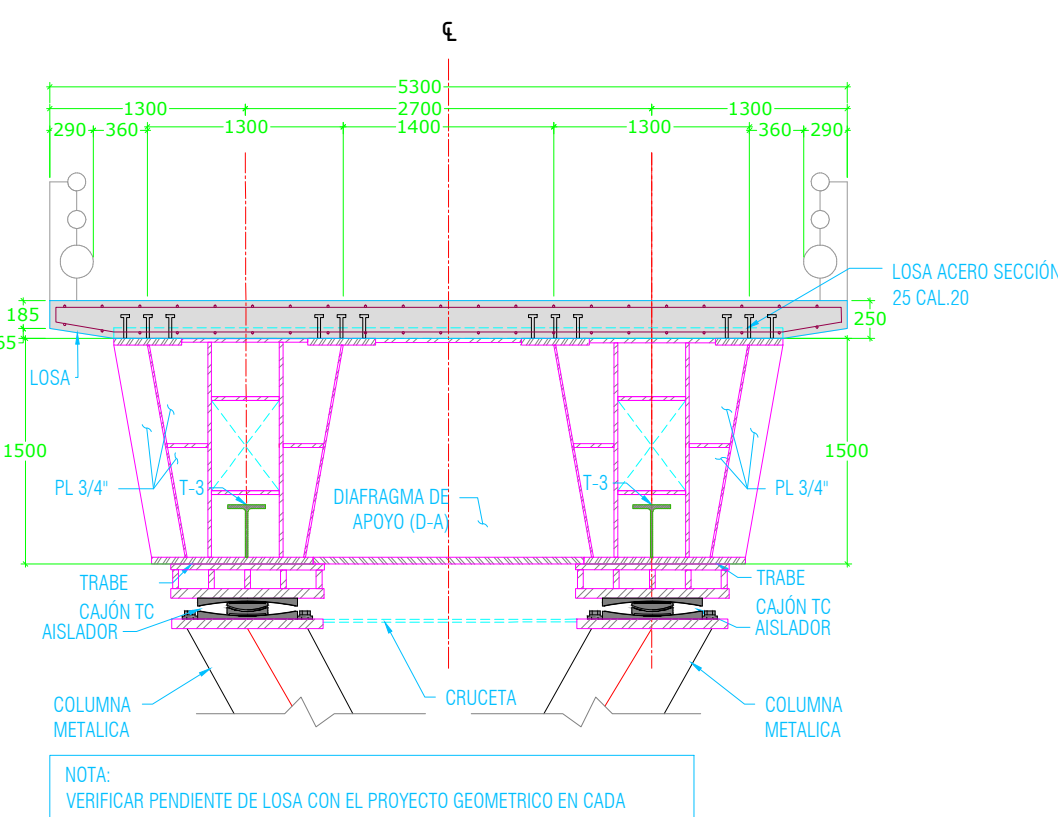
SECCIÓN DE DIAFRAGMA DE APOYO D-A PARA LOSA DE ANCHO 5300
