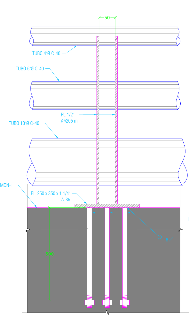
A SECCIÓN 1:10 [mm]
