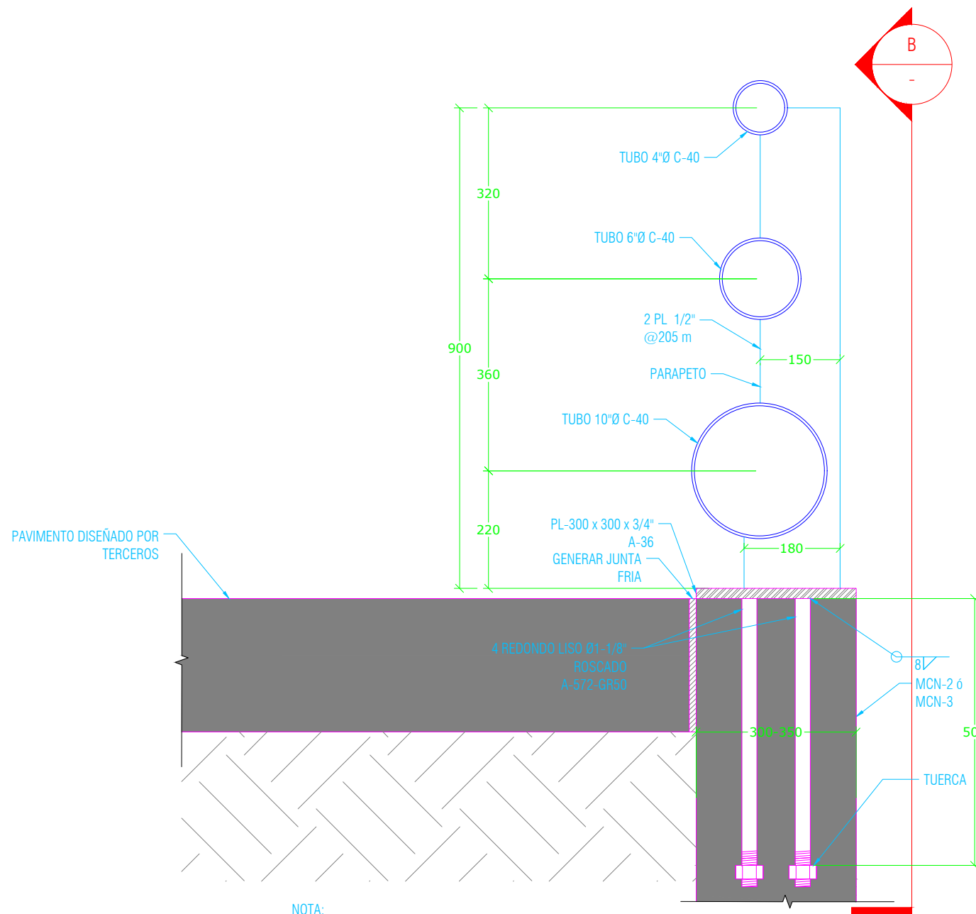
NOTA: SE OMITIÓ EL ACERO DE MURO DE CONTENCIÓN PARA MAYOR CLARIDAD DEL DETALLE 2 DETALLE ANLAJE DE PARAPETO METÁLICO PARA MCN-2 Y MCN-3 1:10 [mm]
