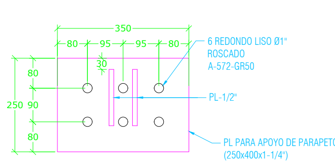
NOTA: LA PLACA APLICA PARA EL MCN-1 4 PLACA 250 x 350 x 1 1/4\" ESC. 1:10 [mm] NOTA: LAS PLACA SON DE ACERO A-36
