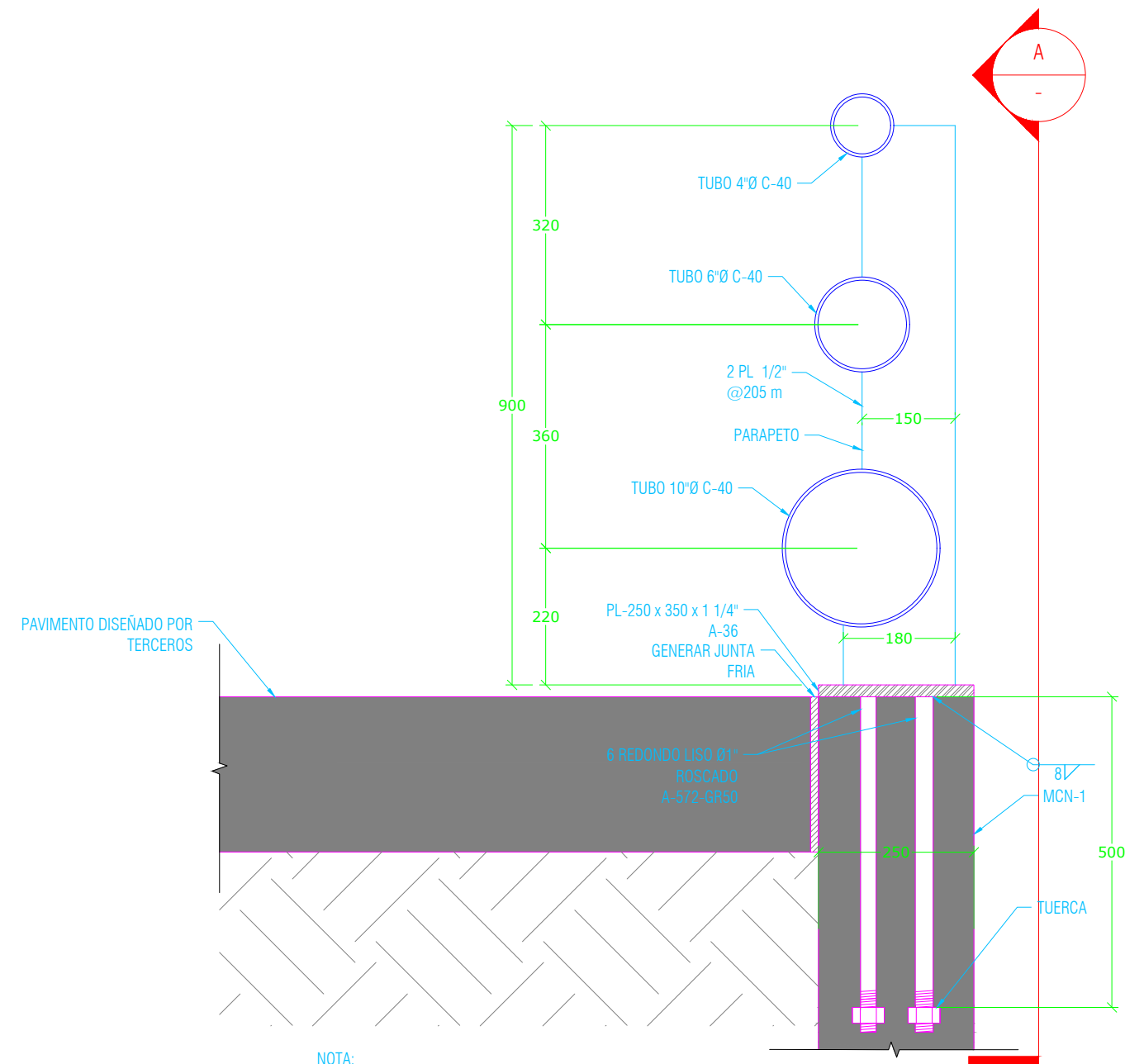
NOTA: SE OMITIÓ EL ACERO DE MURO DE CONTENCIÓN PARA MAYOR CLARIDAD DEL DETALLE 1 DETALLE ANLAJE DE PARAPETO METÁLICO PARA MCN-1 1:10 [mm]
