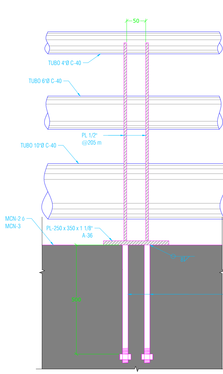
B SECCIÓN 1:10 [mm]
