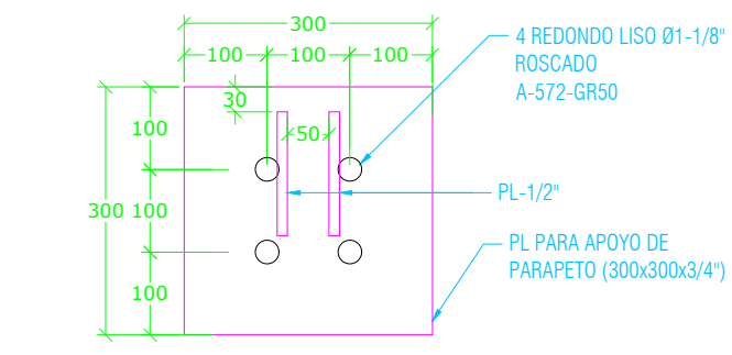
NOTA: LA PLACA APLICA PARA EL MCN-2 Y MCN-3 3 PLACA 300 x 300 x 3/4\" ESC. 1:10 [mm] NOTA: LAS PLACA SON DE ACERO A-36
