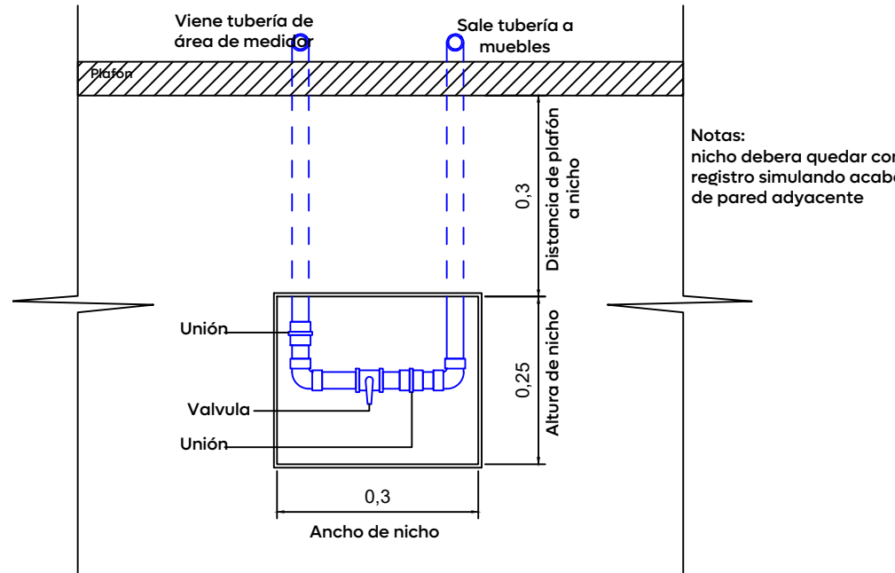
02 Nicho de válvulas Isométrico general Esc. 1:10
