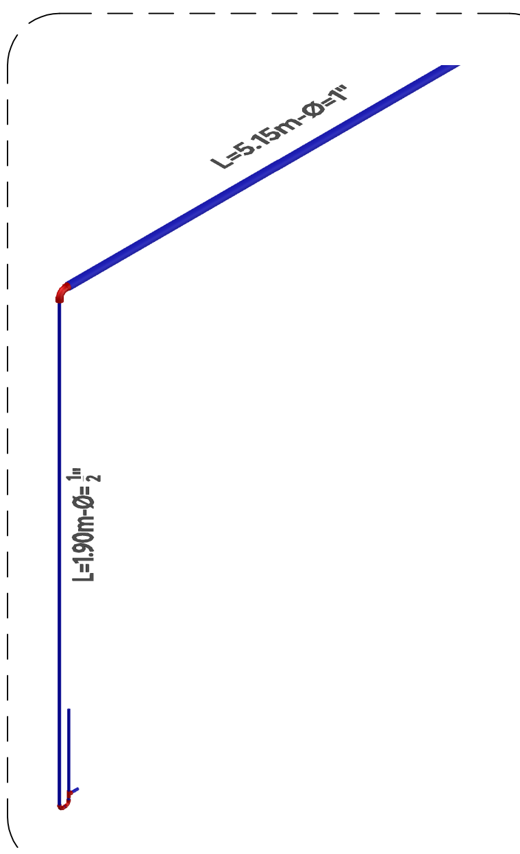
05 Microlocalización 2 Área de lactario Esc. 1:30
