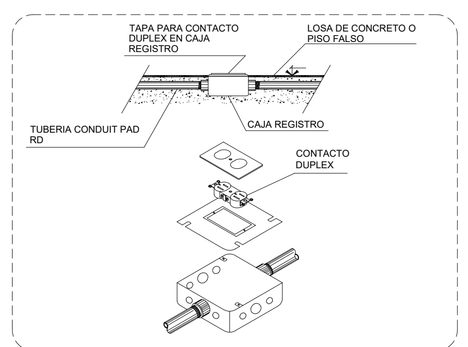
07 Detalle tipo registro en caja de PVC IE-12 S/E
