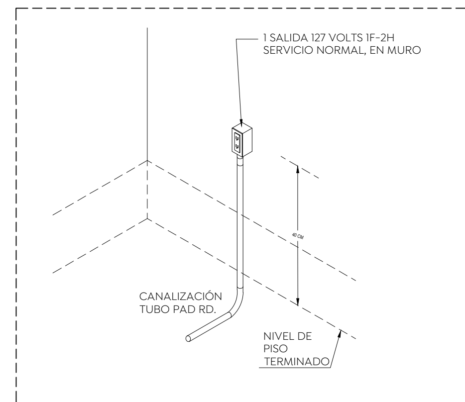
08 Detalle contacto en muro. IE-12 S/E
