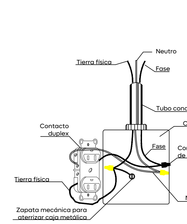
04 Detalle tipo de conexión de contacto polarizado IE-12 S/E
