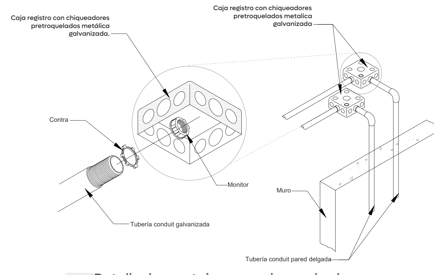
06 Detalle de montaje para caja cuadrada IE-12 S/E
