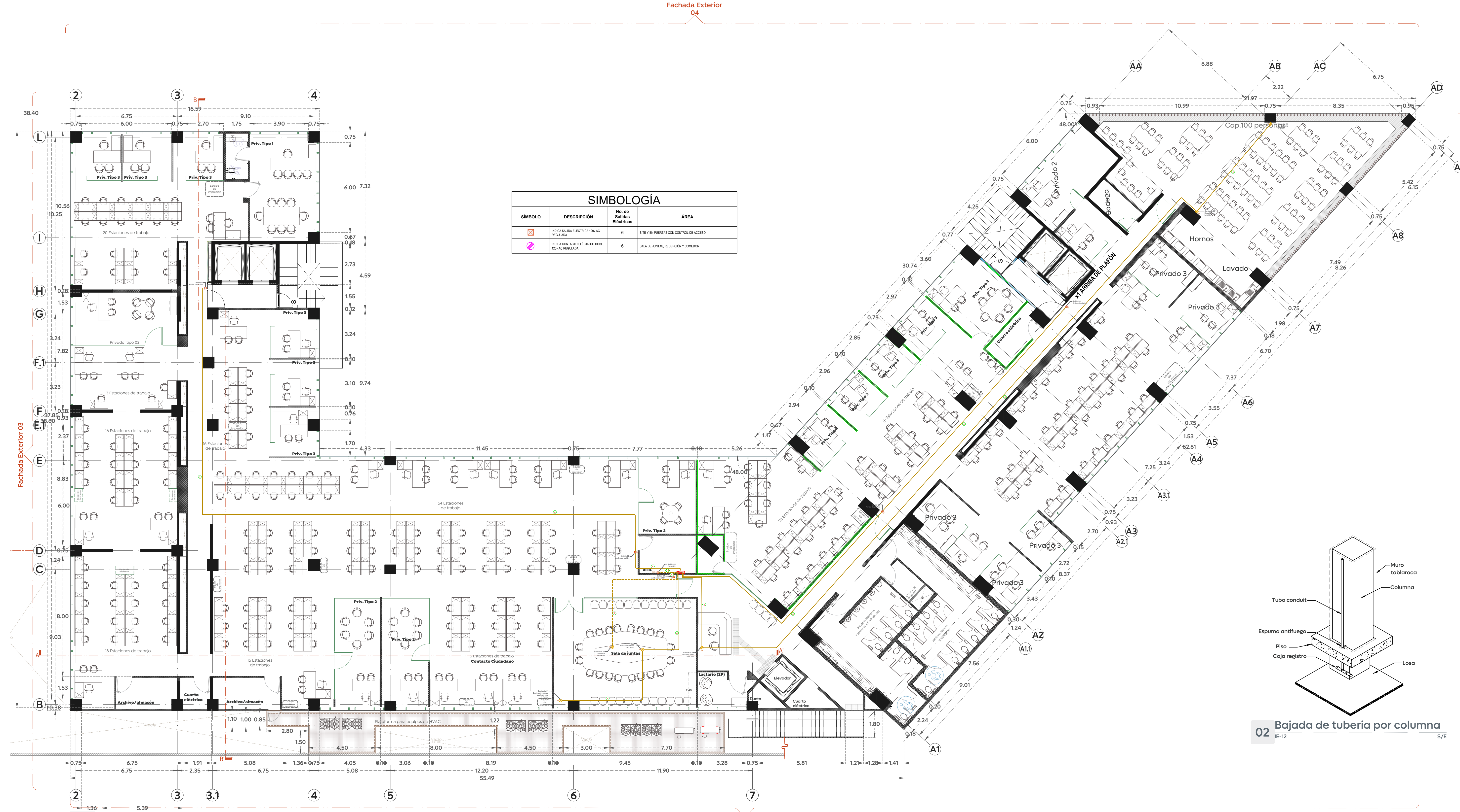
01 Planta alta, N+ 4.43 m Planta de distribución arquitectónica Esc. 1:150
