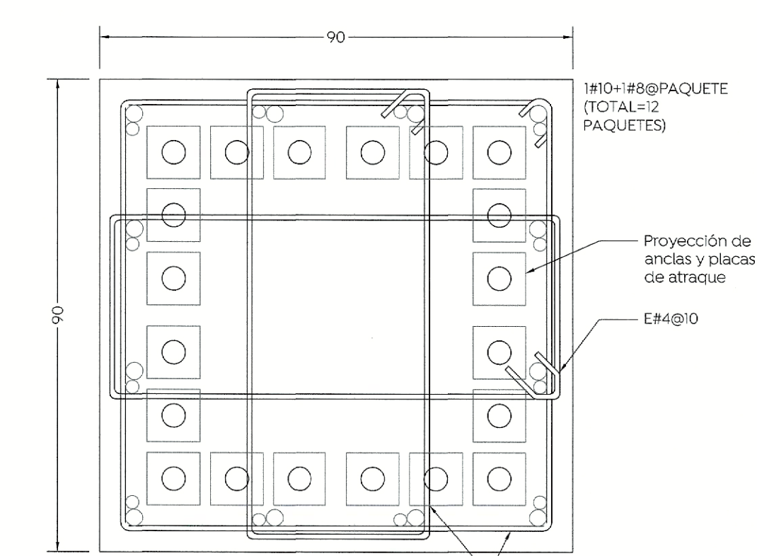
DADO DA-1 ESC 1:10 (cm)
