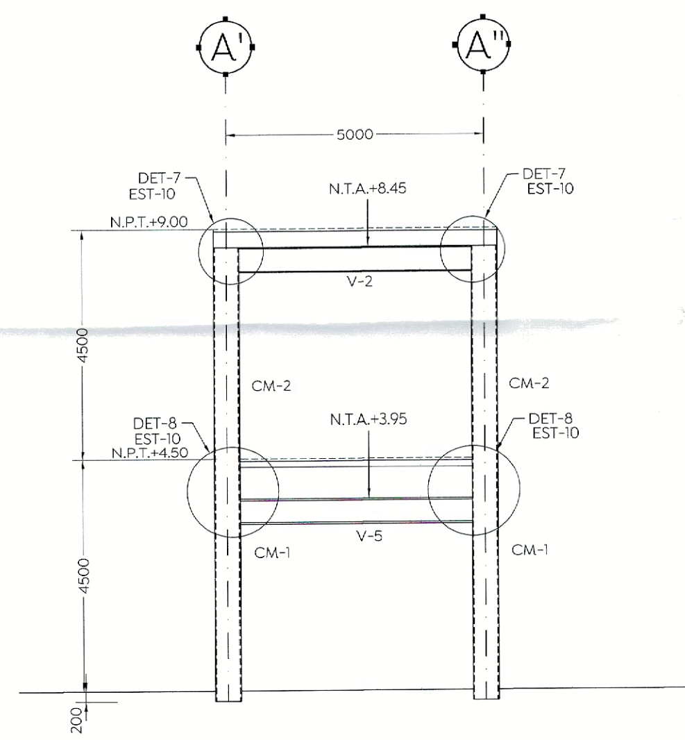
ALZADO MARCO EJE 5', 6' y 7' ESC. 1:100 (mm)
