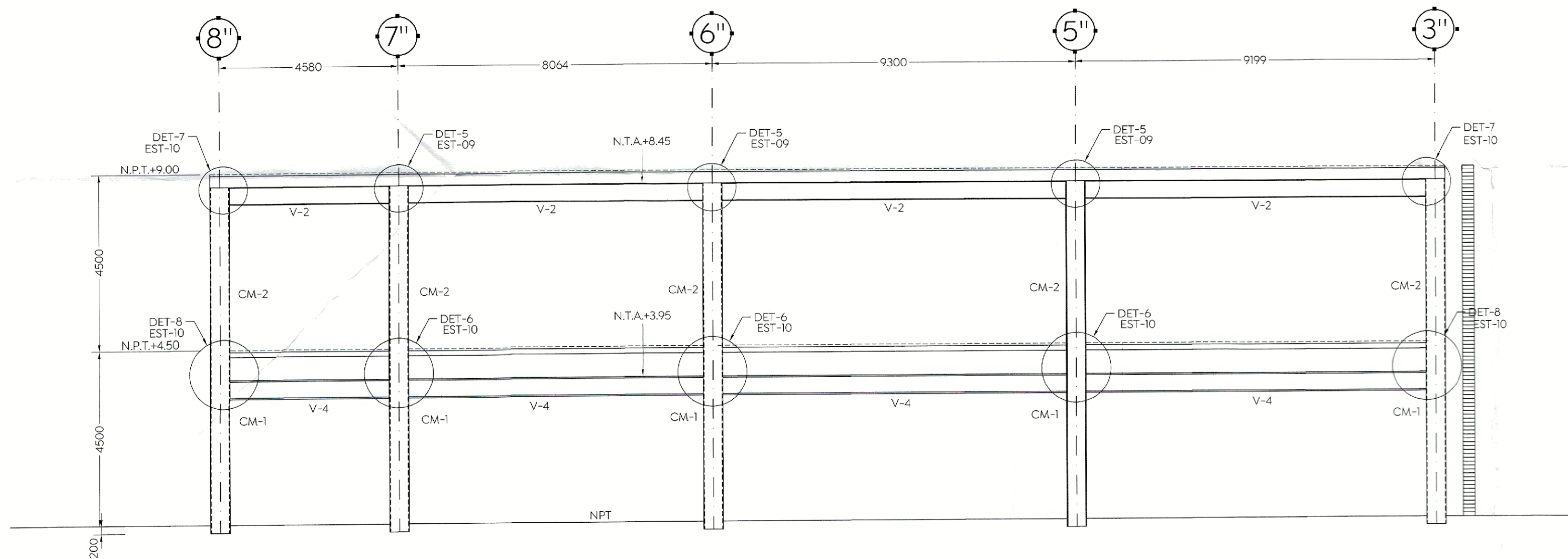
ALZADO MARCO EJE J' ESC. 1:100 (mm)
