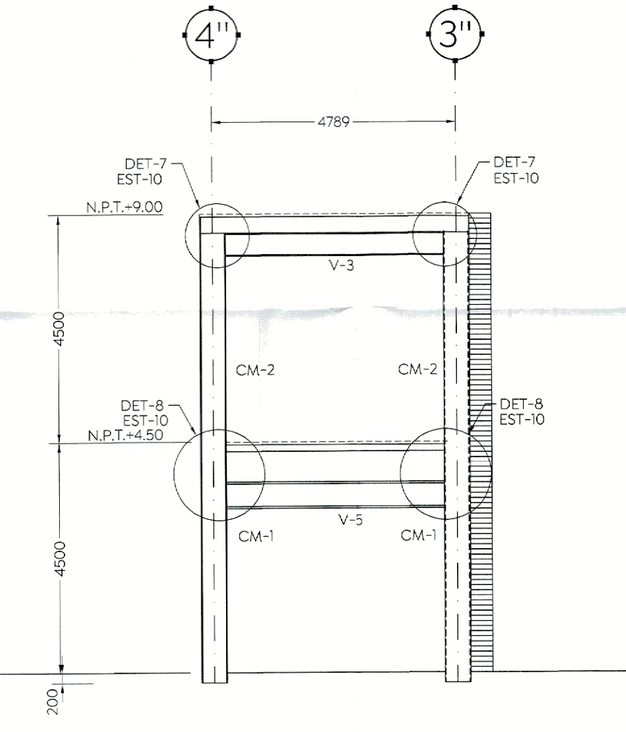
ALZADO MARCO EJE G' ESC. 1:100 (mm)
