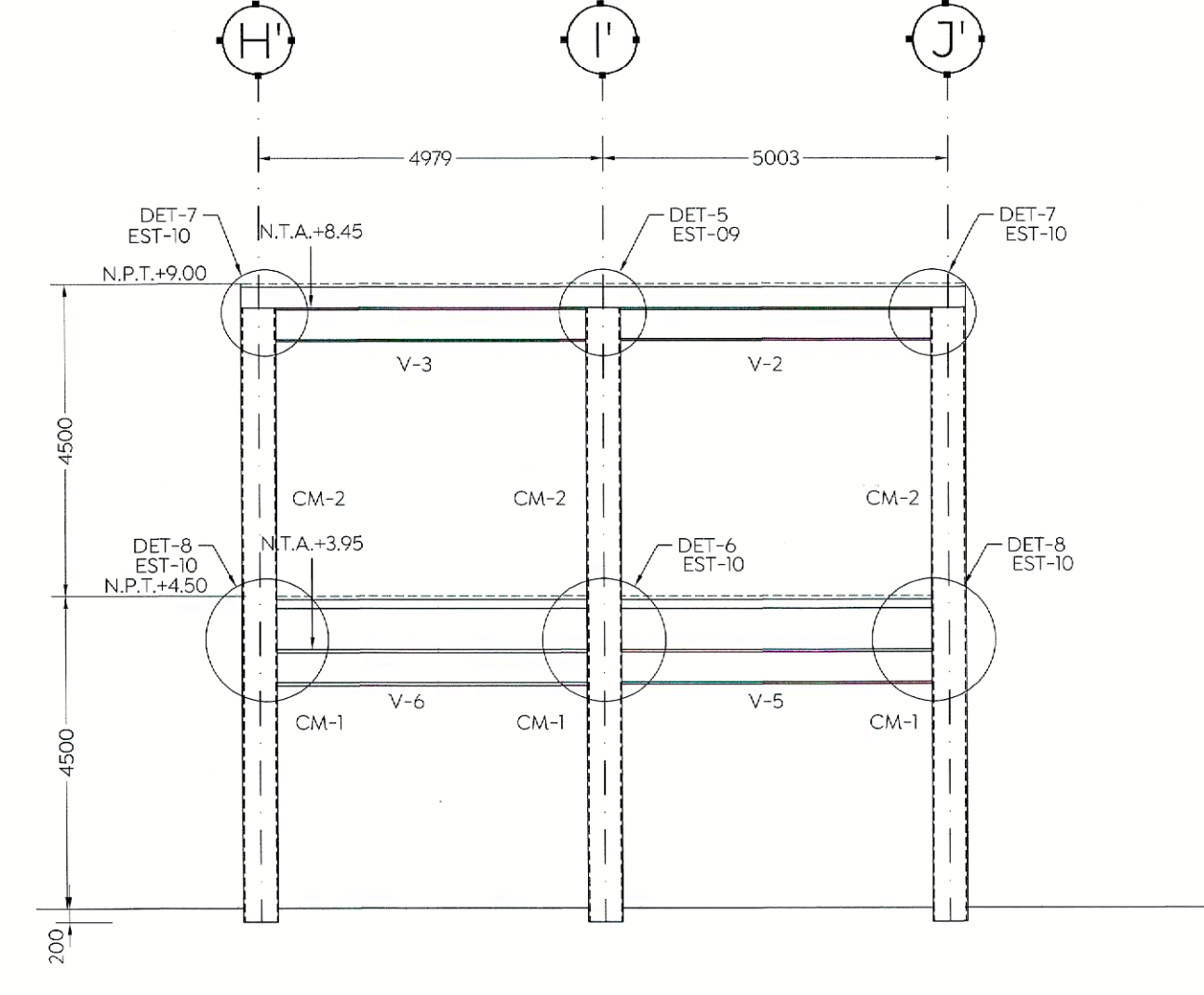
ALZADO MARCO EJE 8' ESC. 1:100 (mm)
