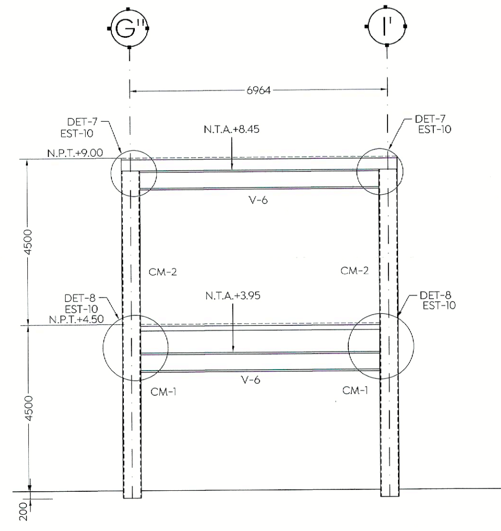
ALZADO MARCO EJE 4' ESC. 1:100 (mm)
