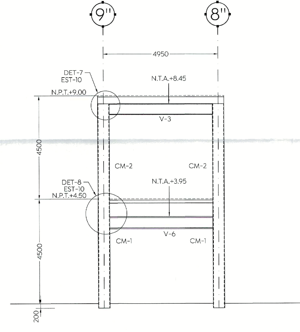
ALZADO MARCO EJE H' ESC. 1:100 (mm)
