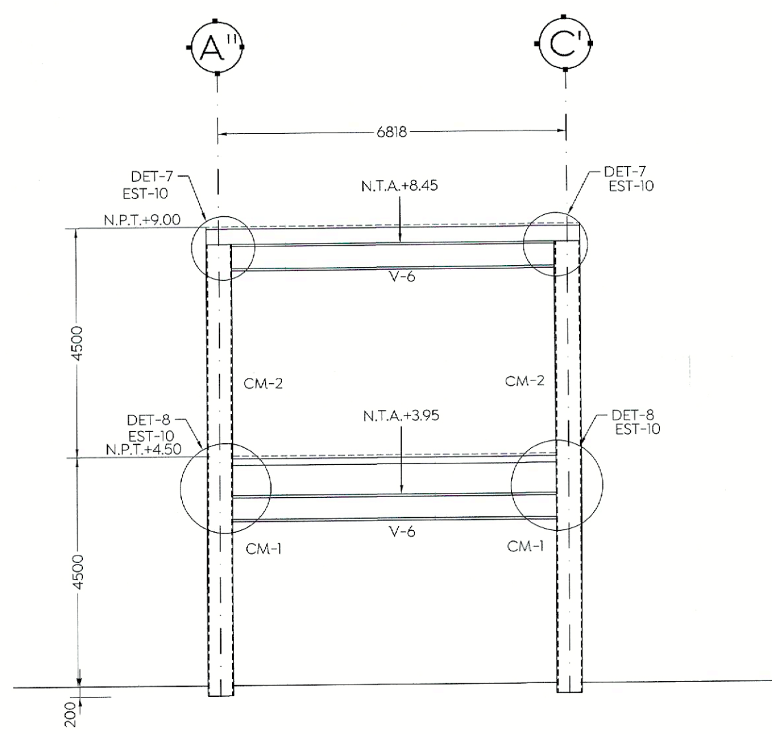
ALZADO MARCO EJE 4' ESC. 1:100 (mm)
