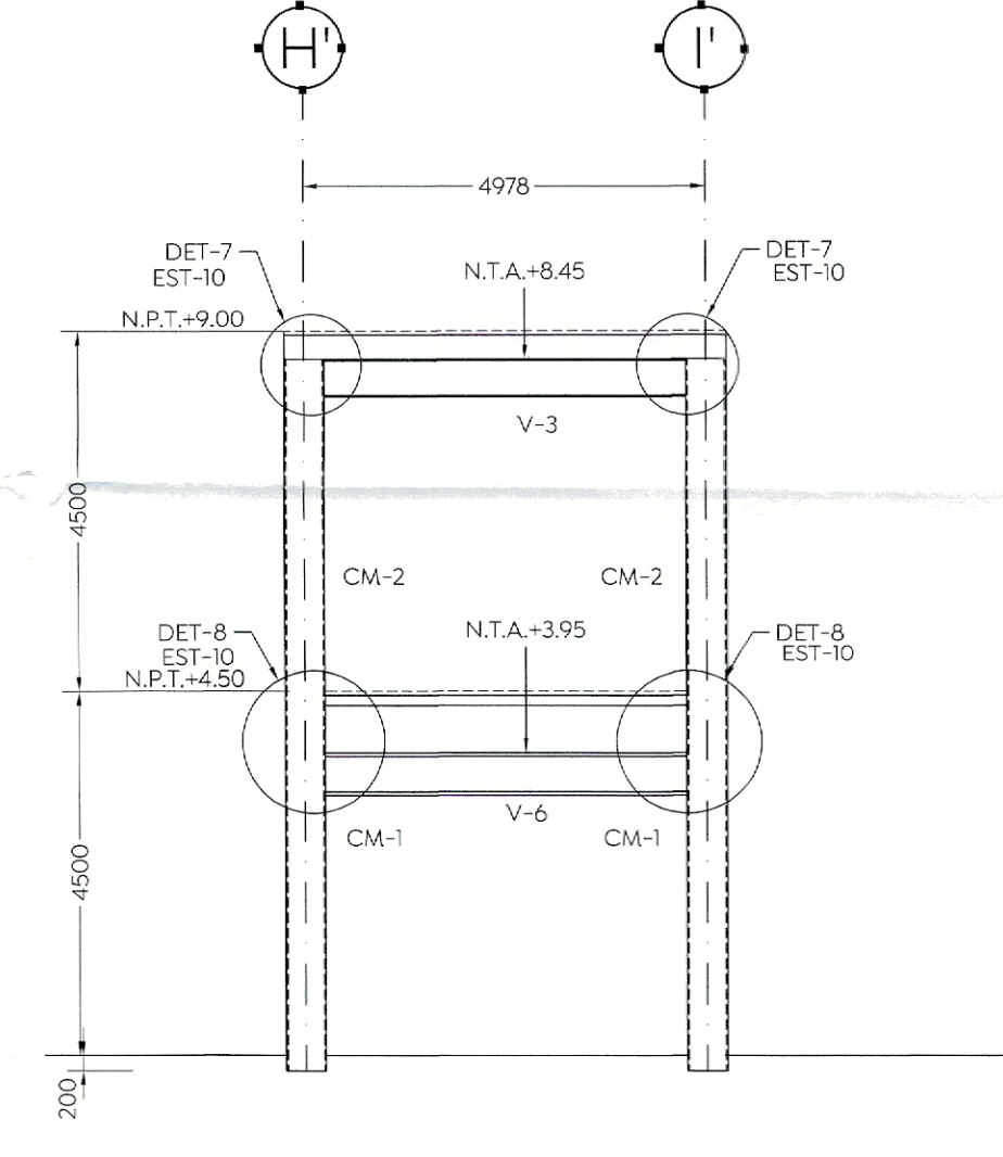
ALZADO MARCO EJE 9' ESC. 1:100 (mm)
