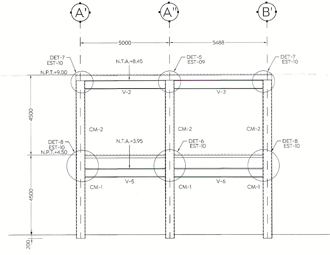
ALZADO MARCO EJE 8' ESC. 1:100 (mm)
