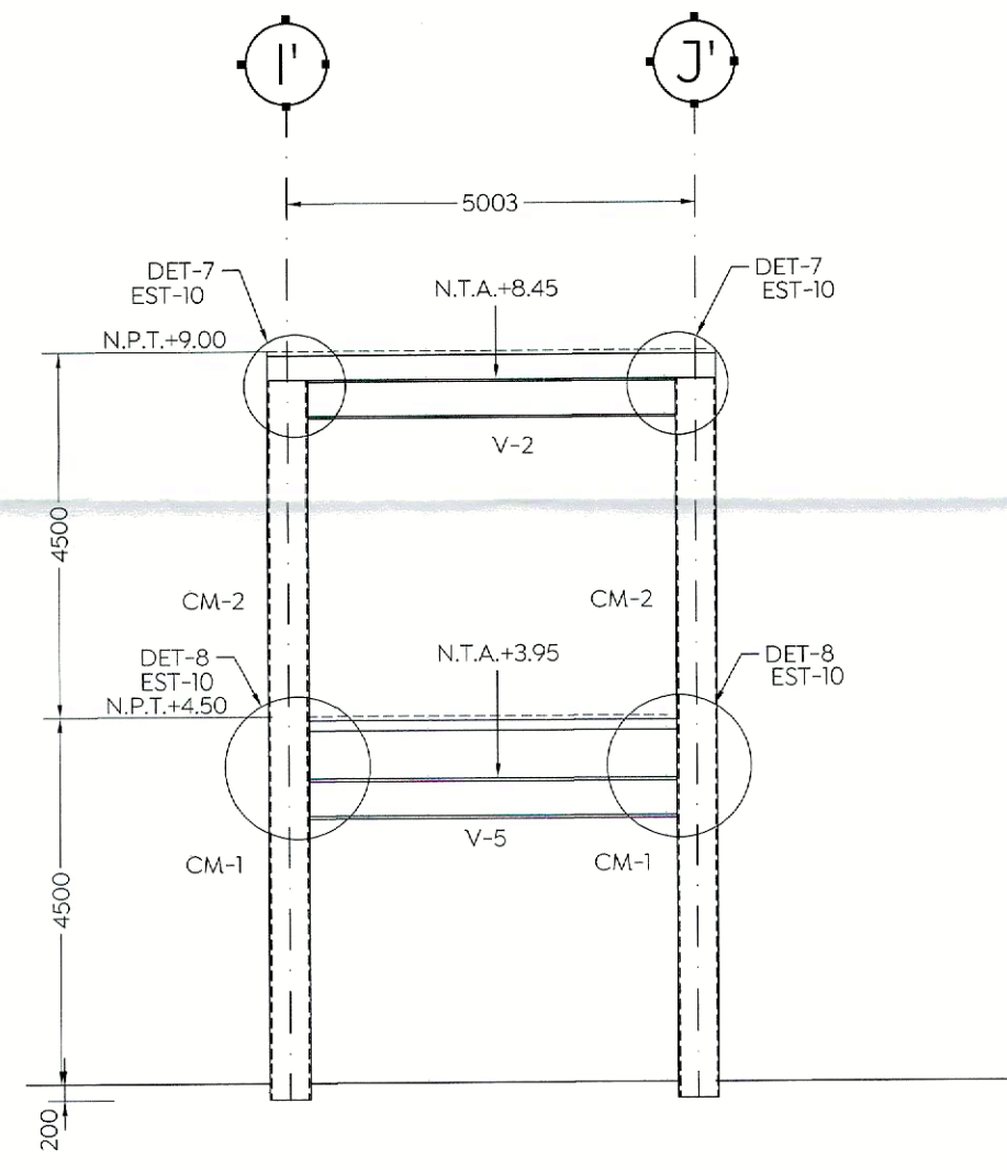
ALZADO MARCO EJE 5', 6' y 7' ESC. 1:100 (mm)
