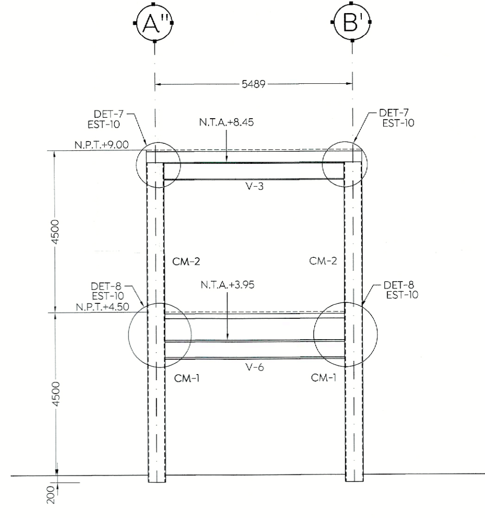
ALZADO MARCO EJE 9' ESC. 1:100 (mm)
