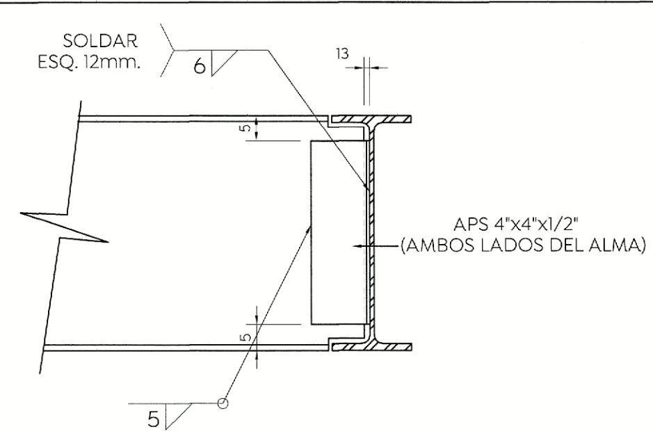
DETALLE TÍPICO DE CONEXIÓN A CORTANTE
