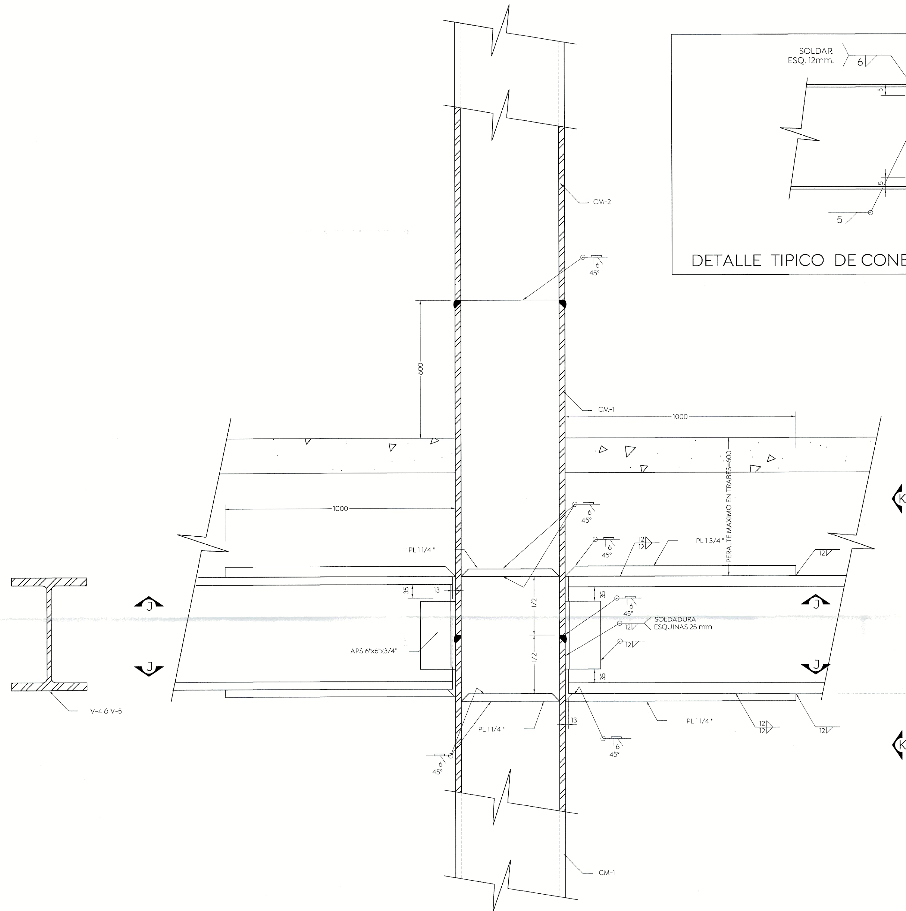
DETALLE 6
