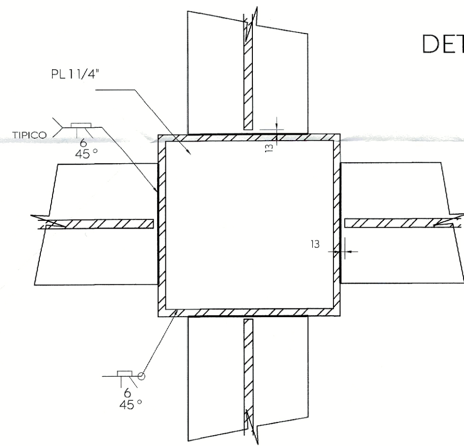
SECCIÓN J-J
