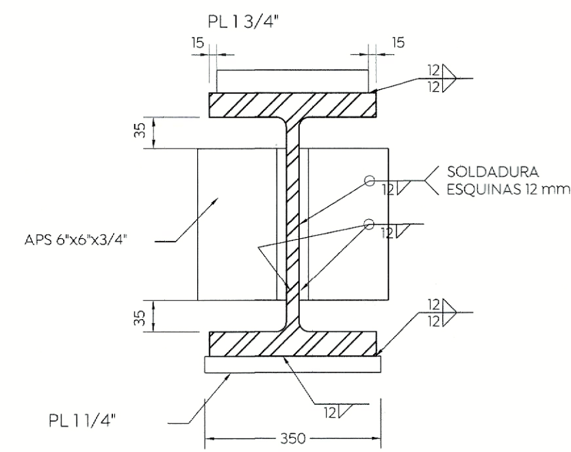
SECCIÓN K-K
