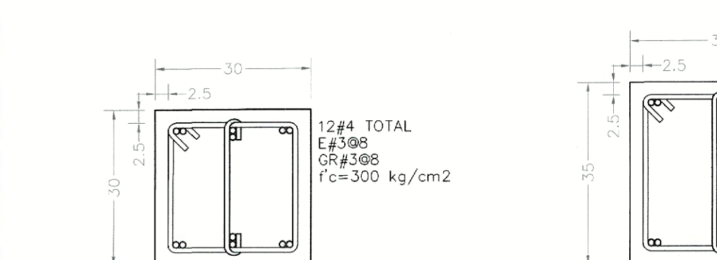
CASTILLO CABEZAL KC-1 VISTA EN SECCIÓN ESC. 1:10
