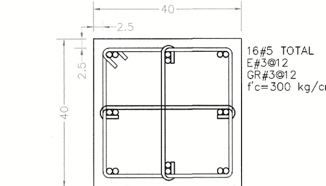
CASTILLO CABEZAL KC-3 VISTA EN SECCIÓN ESC. 1:10
