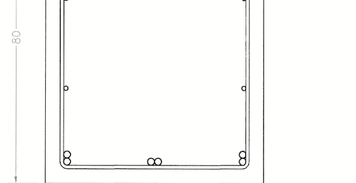
CONTRATRABE CT-2 VISTA EN SECCIÓN ESC. 1:10
