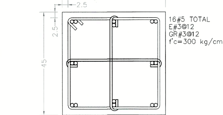
CASTILLO CABEZAL KC-4 VISTA EN SECCIÓN ESC. 1:10
