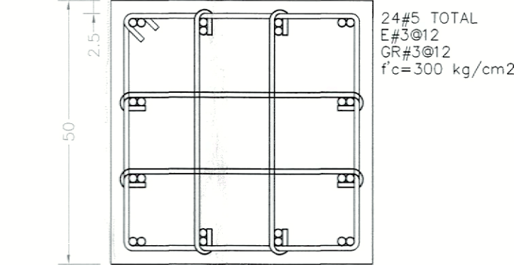
CASTILLO CABEZAL KC-5 VISTA EN SECCIÓN ESC. 1:10
