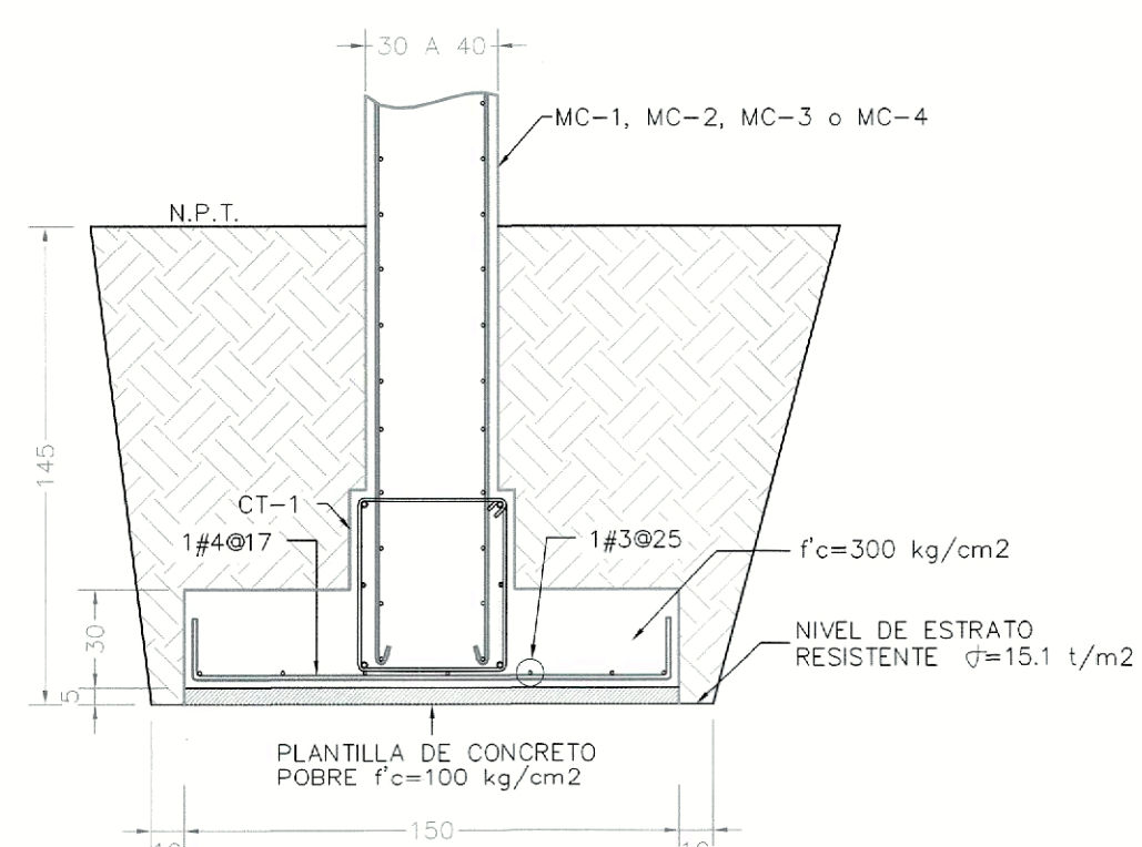
ZAPATA CORRIDA ZC-1 VISTA EN SECCIÓN ESC. 1:25
