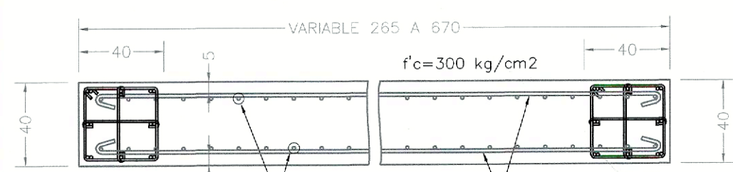
MURO DE CONCRETO MC-3 VISTA EN PLANTA ESC. 1:25
