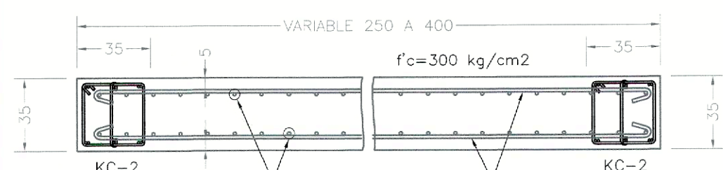
MURO DE CONCRETO MC-2 VISTA EN PLANTA ESC. 1:25
