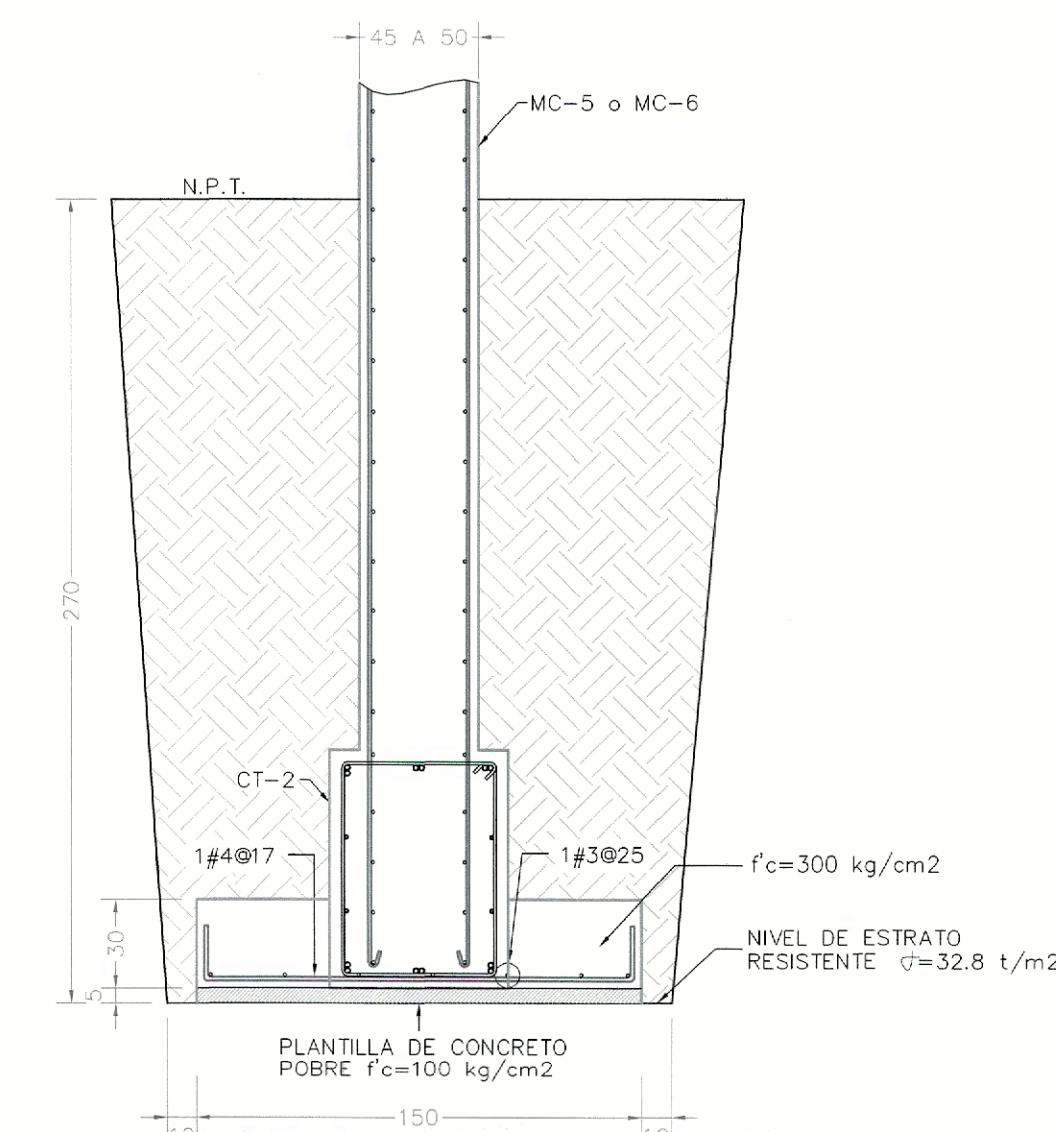
ZAPATA CORRIDA ZC-3 VISTA EN SECCIÓN ESC. 1:25
