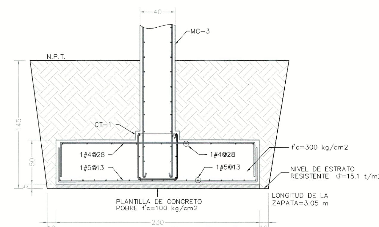
ZAPATA CORRIDA ZC-2 VISTA EN SECCIÓN ESC. 1:25
