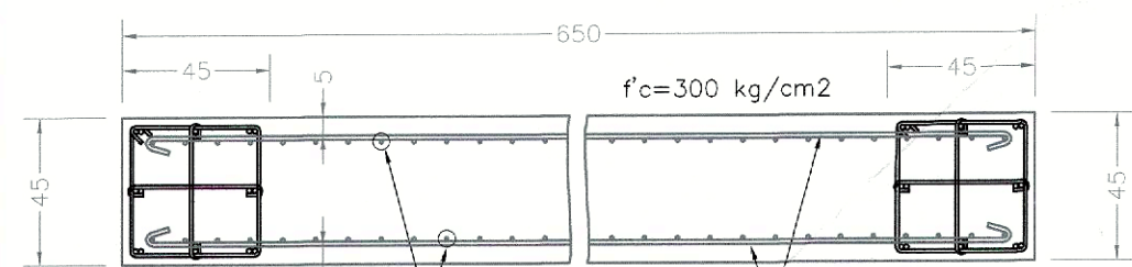
MURO DE CONCRETO MC-4 VISTA EN PLANTA ESC. 1:25
