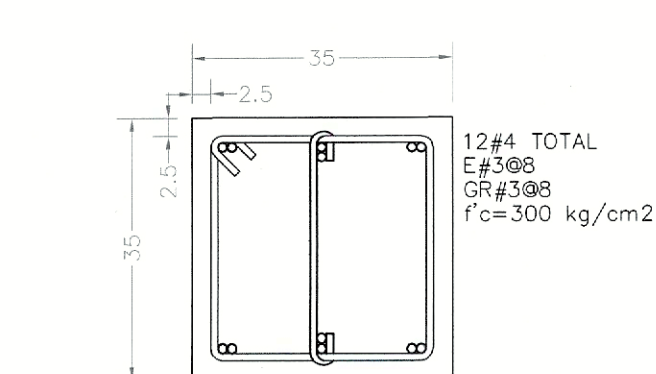
CASTILLO CABEZAL KC-2 VISTA EN SECCIÓN ESC. 1:10
