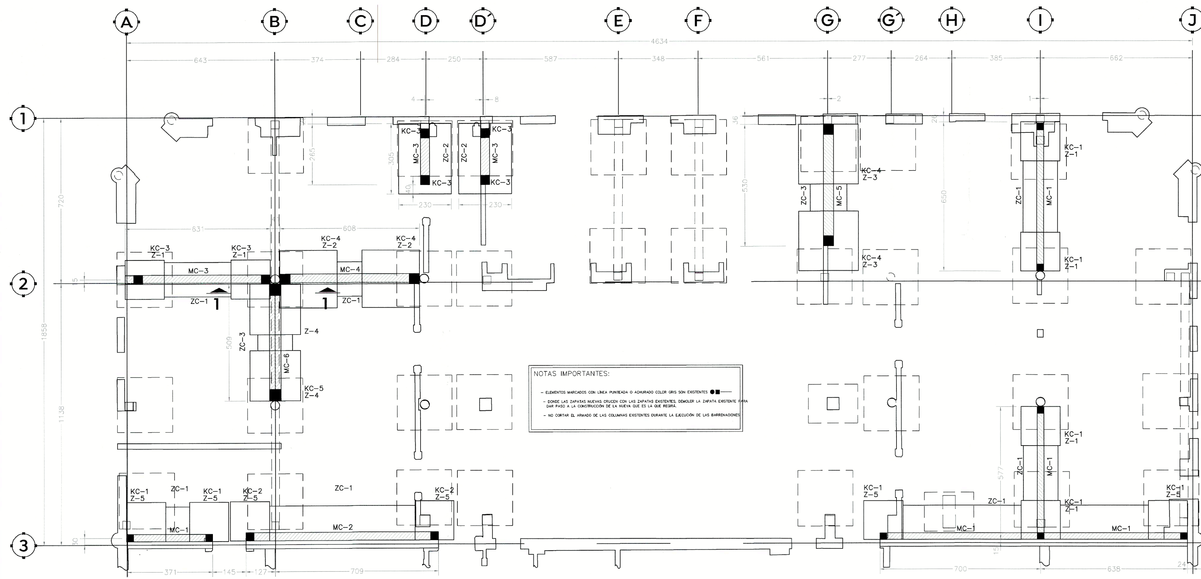
PLANTA DE CIMENTACIÓN ESC. 1:300
