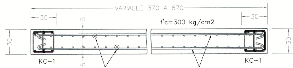
MURO DE CONCRETO MC-1 VISTA EN PLANTA ESC. 1:25
