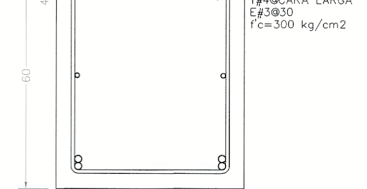
CONTRATRABE CT-1 VISTA EN SECCIÓN ESC. 1:10
