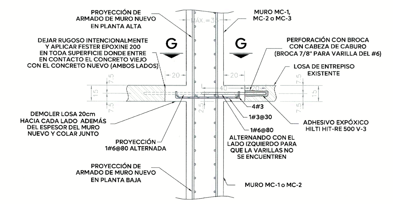
DETALLE 8: CONEXIÓN ENTRE MUROS NUEVOS MC-1 Y MC-2 A LOSA EXISTENTE (APLICA SÓLO DONDE NO HAY TRABE) VISTA EL ALZADO ESC. 1:20
