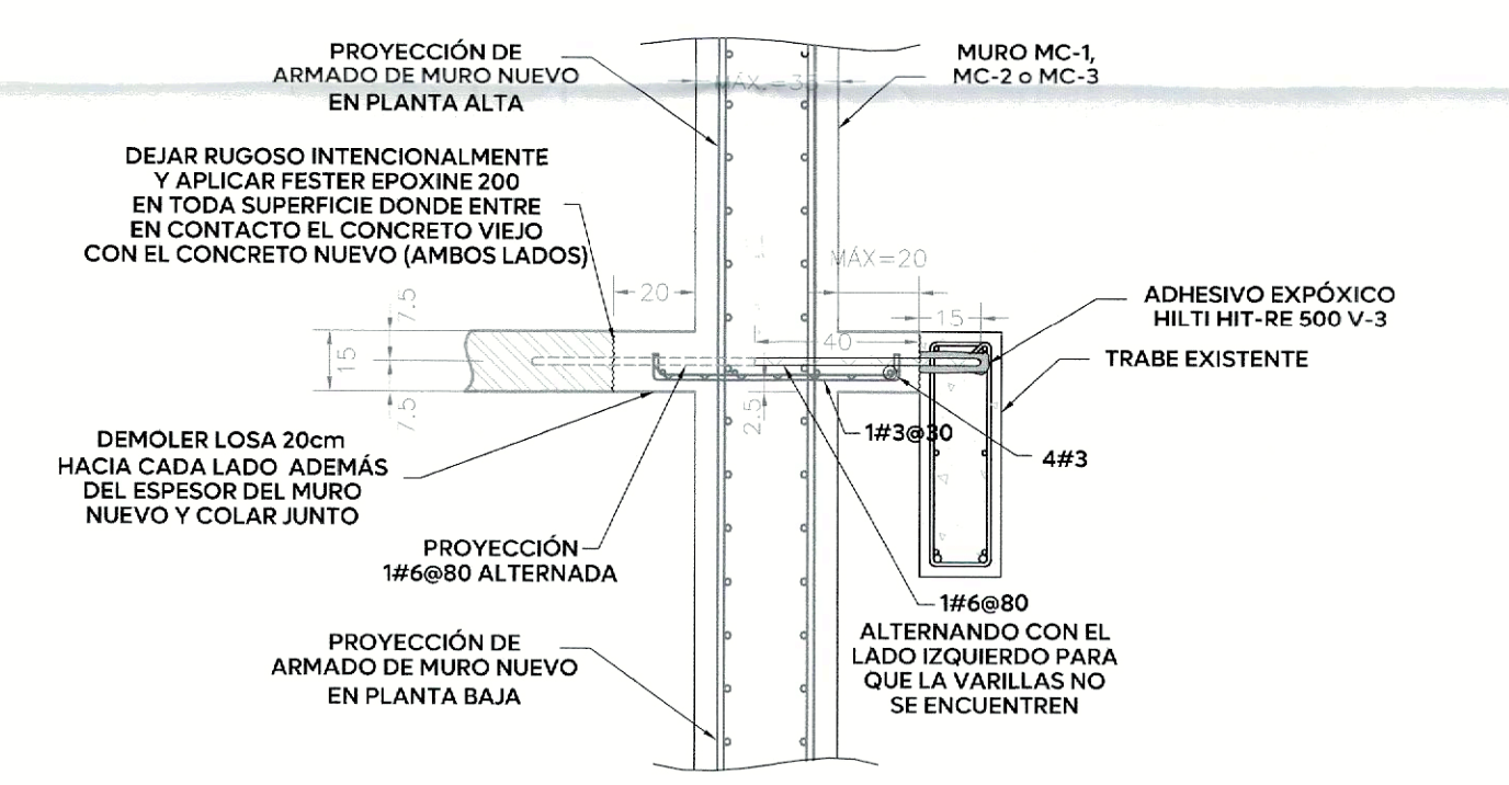
DETALLE 9: CONEXIÓN ENTRE MUROS NUEVOS A LOSA Y TRABE EXISTENTES VISTA EL ALZADO ESC. 1:20
