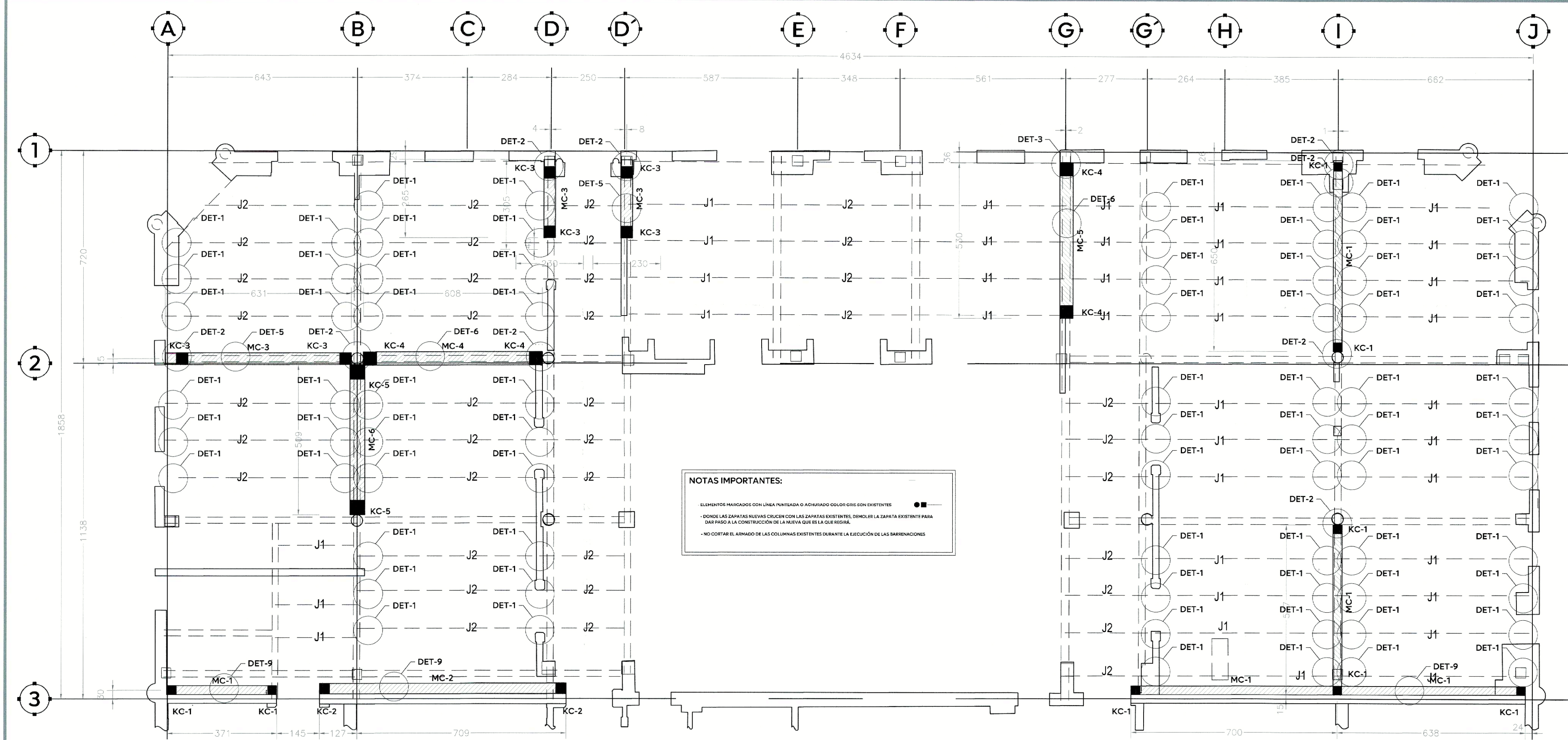
PLANTA BAJA ESC: 1:100
