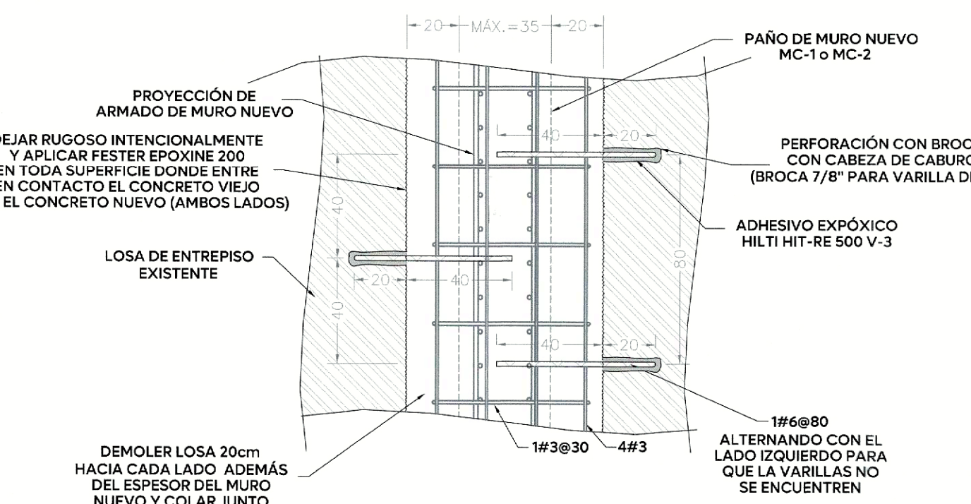
SECCIÓN G-G VISTA EN PLANTA ESC. 1:20
