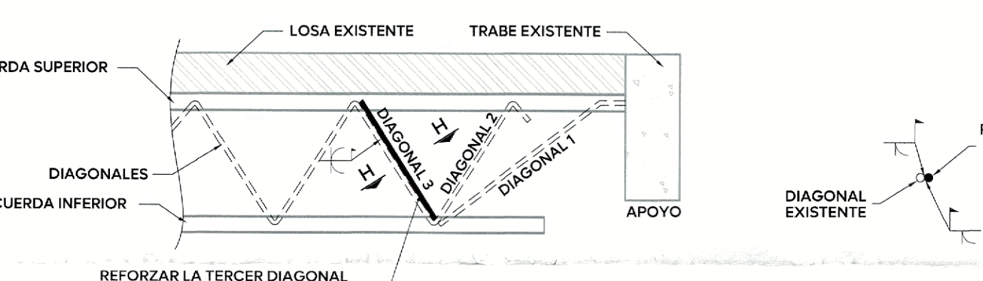
DETALLE 1: REFUERZO DE JOIST VISTA EL ALZADO ESC. 1:20
