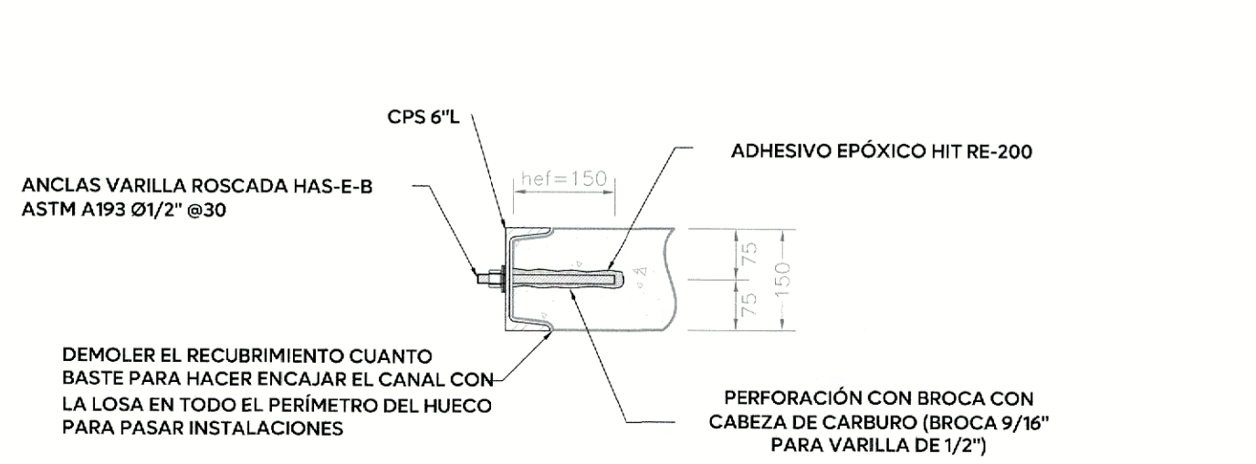
DETALLE DE REFUERZO PARA EL CONFINAMIENTO PERIMETRAL DE PASOS DE INSTALACIONES A TRAVÉS DE LAS LOSAS EXISTENTES VISTA EN SECCIÓN ESC. 1:10
