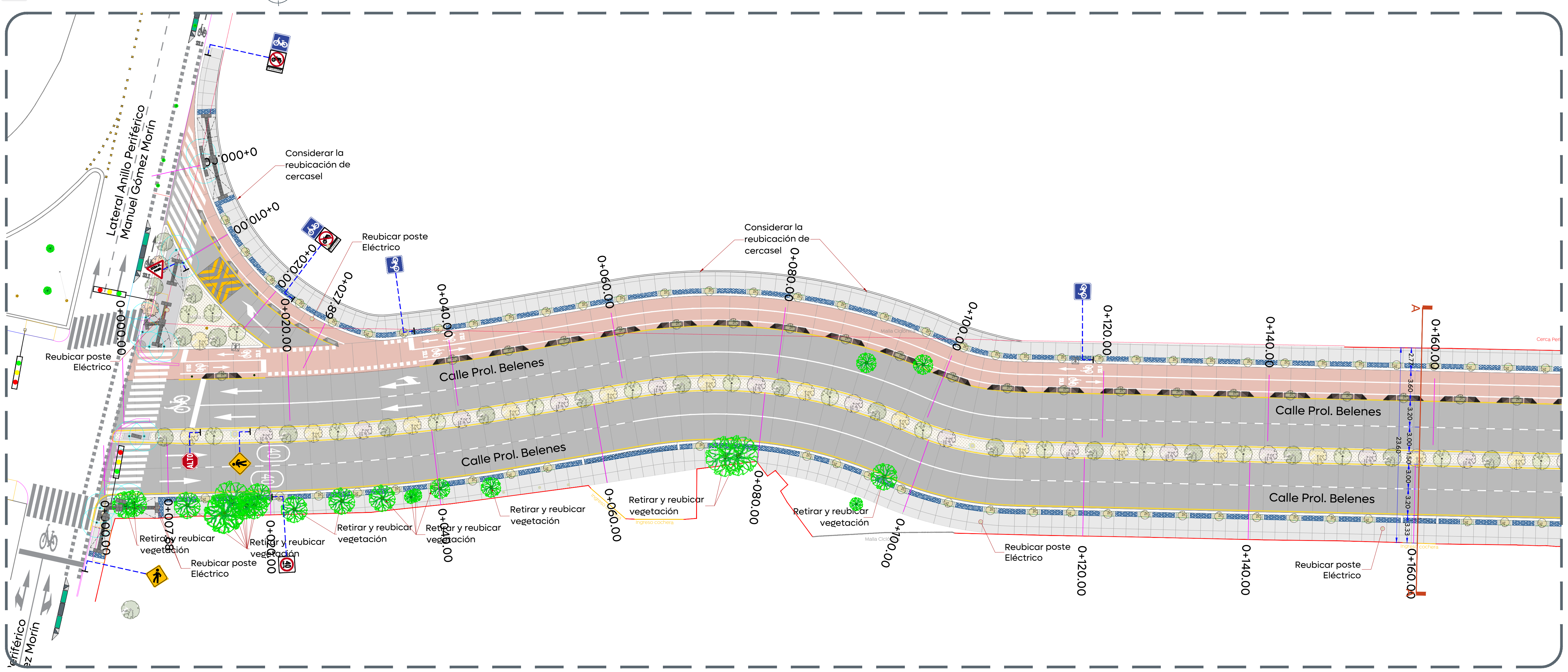
01 Planta arquitectónica Prol. Belenes (frente 01) 1:250
