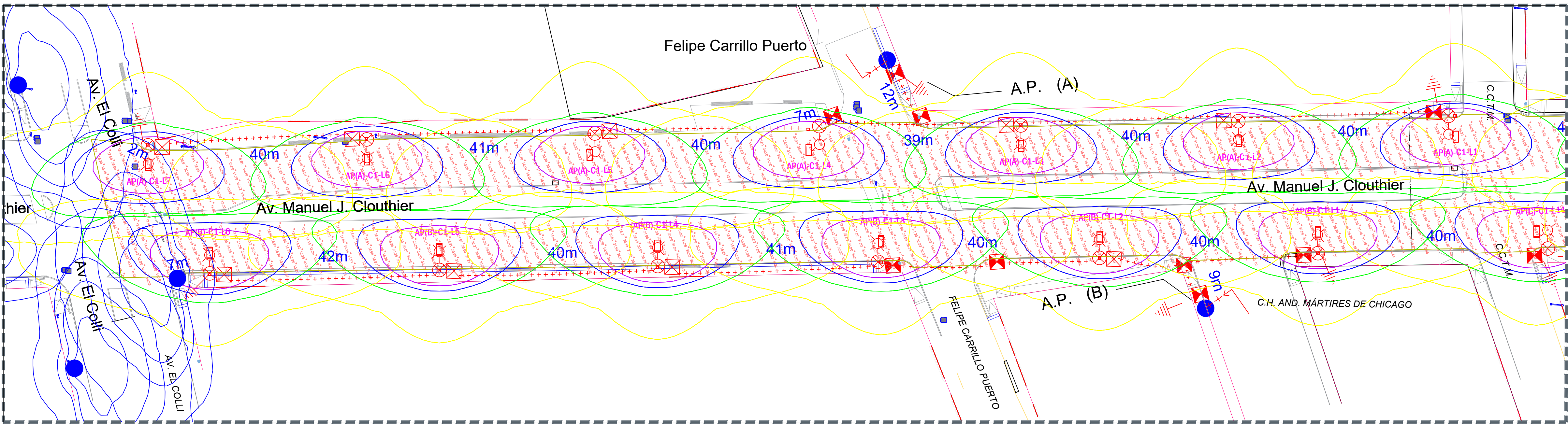
02 Planta Fotométrico URB_AP.02 Escala: 1:450
