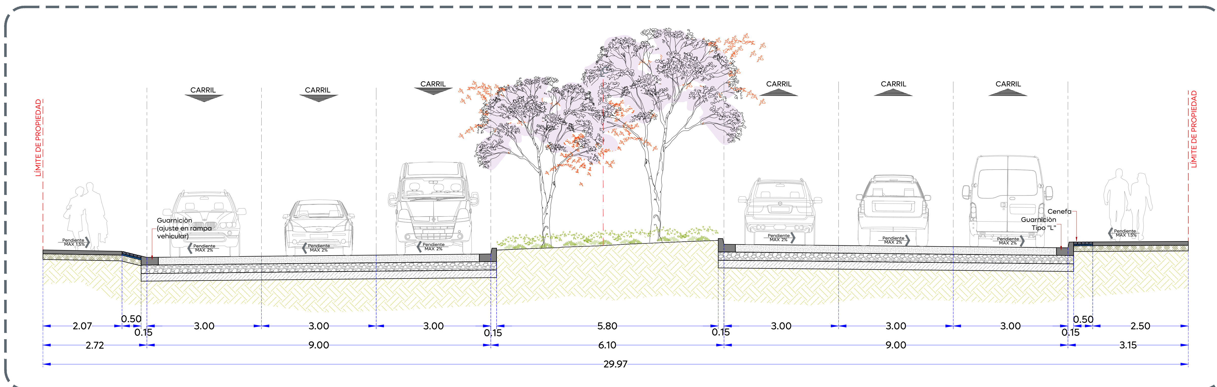
Sección A-A Esc. 1:50
