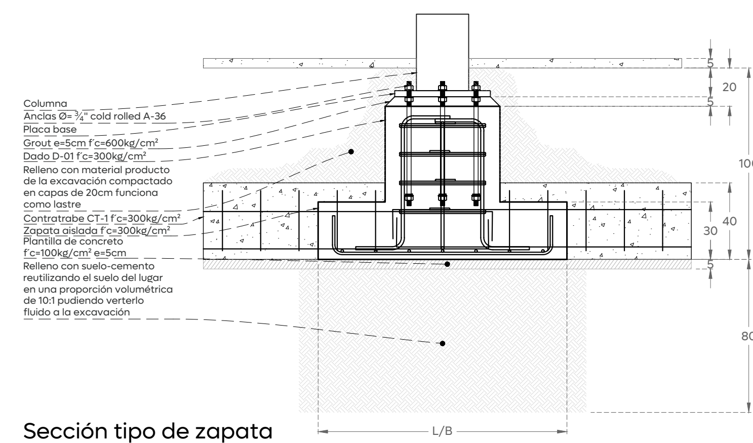
03 Detalle de zapatas Detalles estructurales COTAS: cm Esc. 1:20
