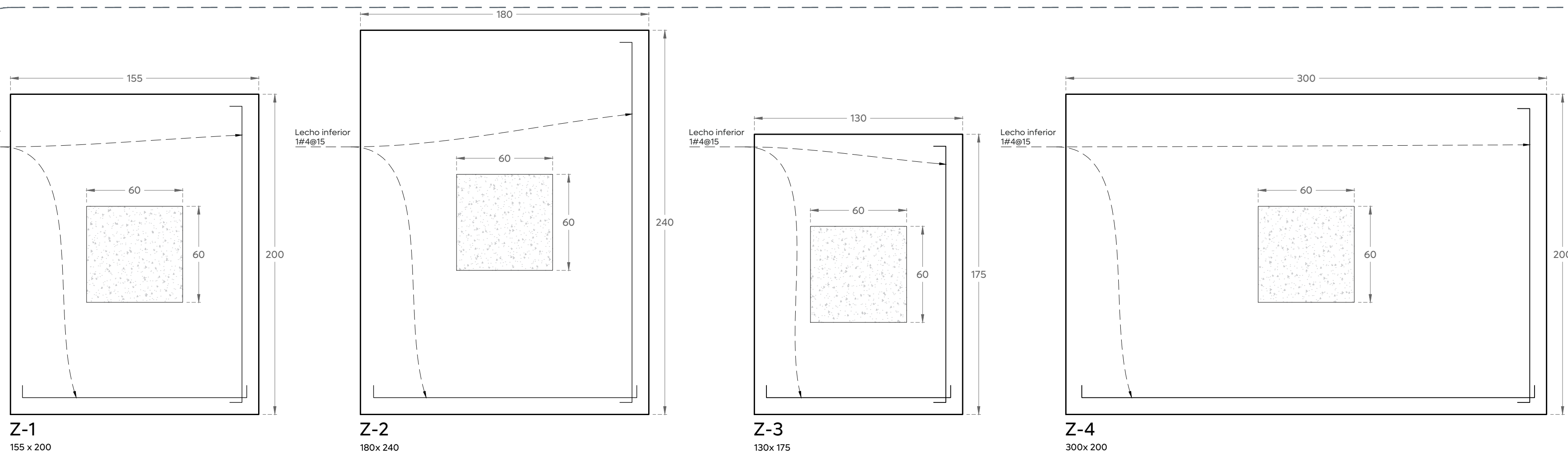
02 Detalle de zapatas Detalles estructurales COTAS: cm Esc. 1:20
