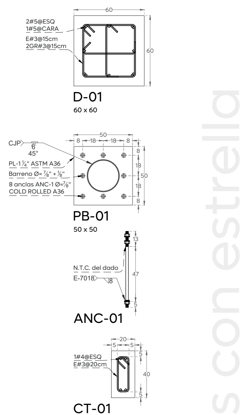
04 Dado, Placa base, Ancla, Contratrabe Detalles estructurales COTAS: cm Esc. 1:20
