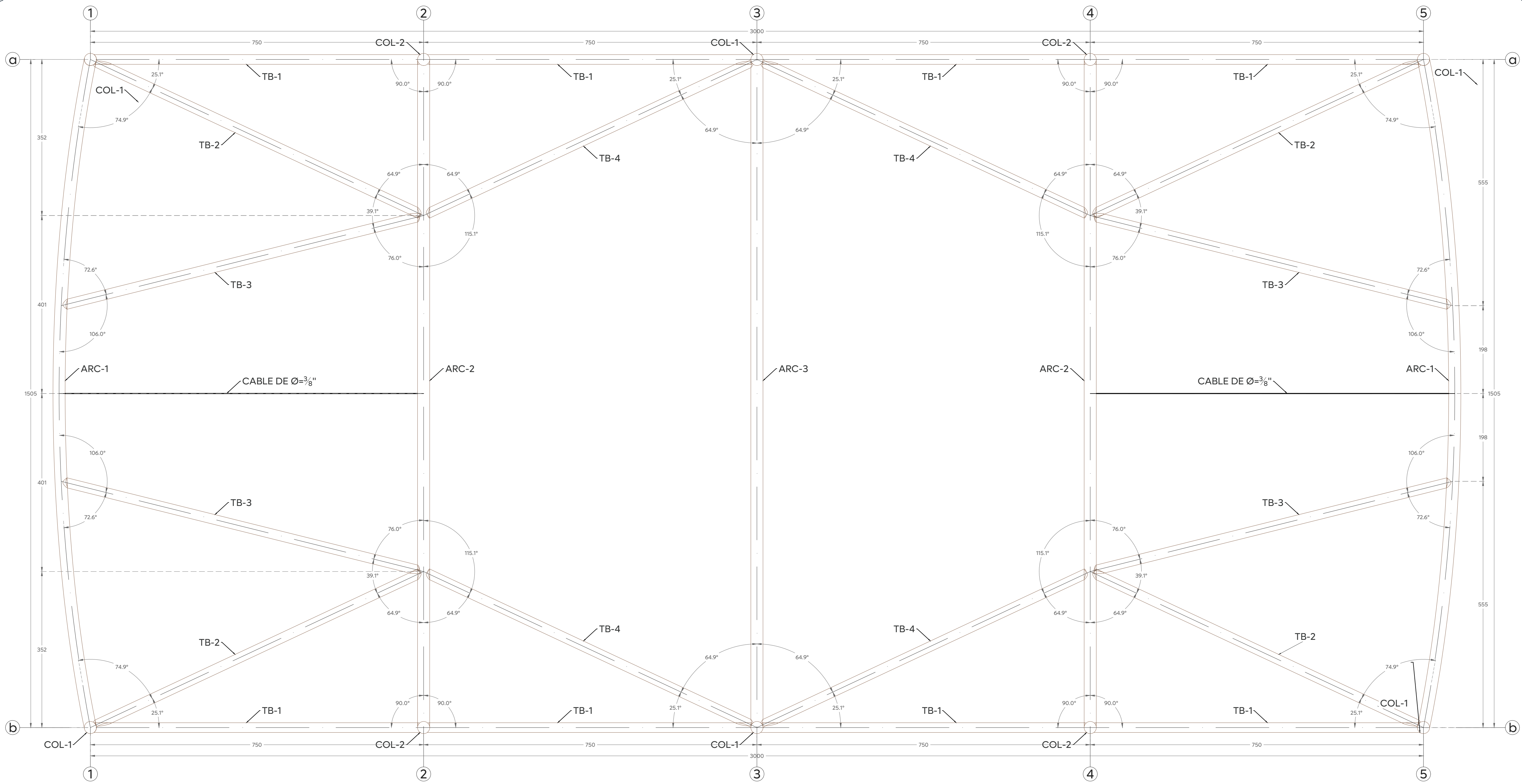
01 Planta estructural
