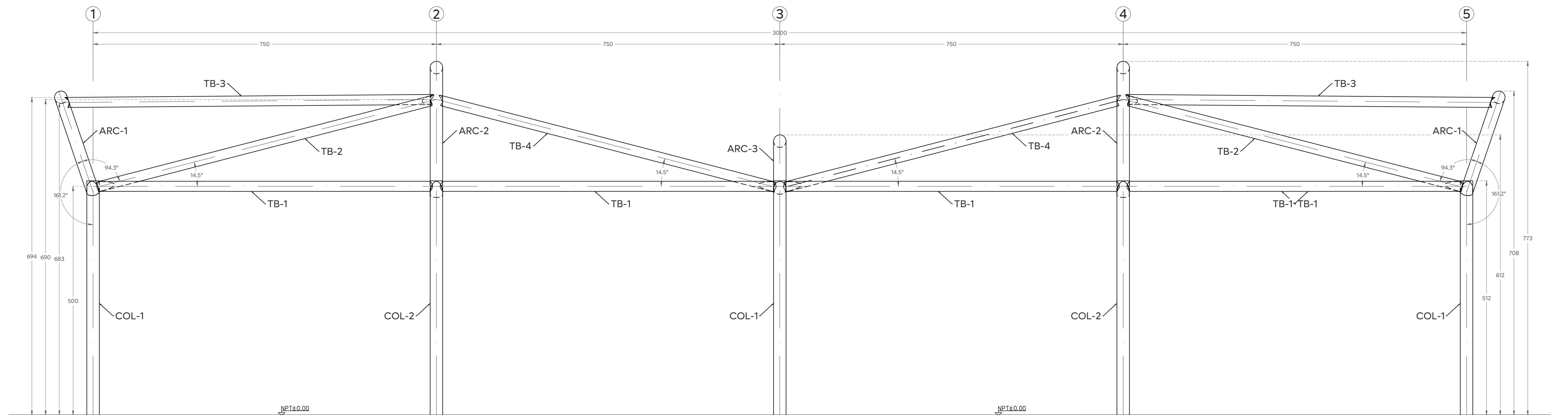
02 Alzado lateral
