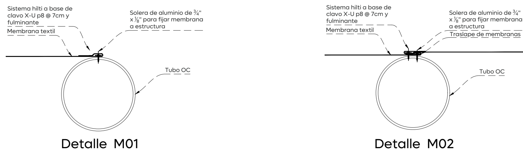
02 Detalle de fijación de membrana, simple M01 y doble M02 Detalle de construcción Esc. 1:20
