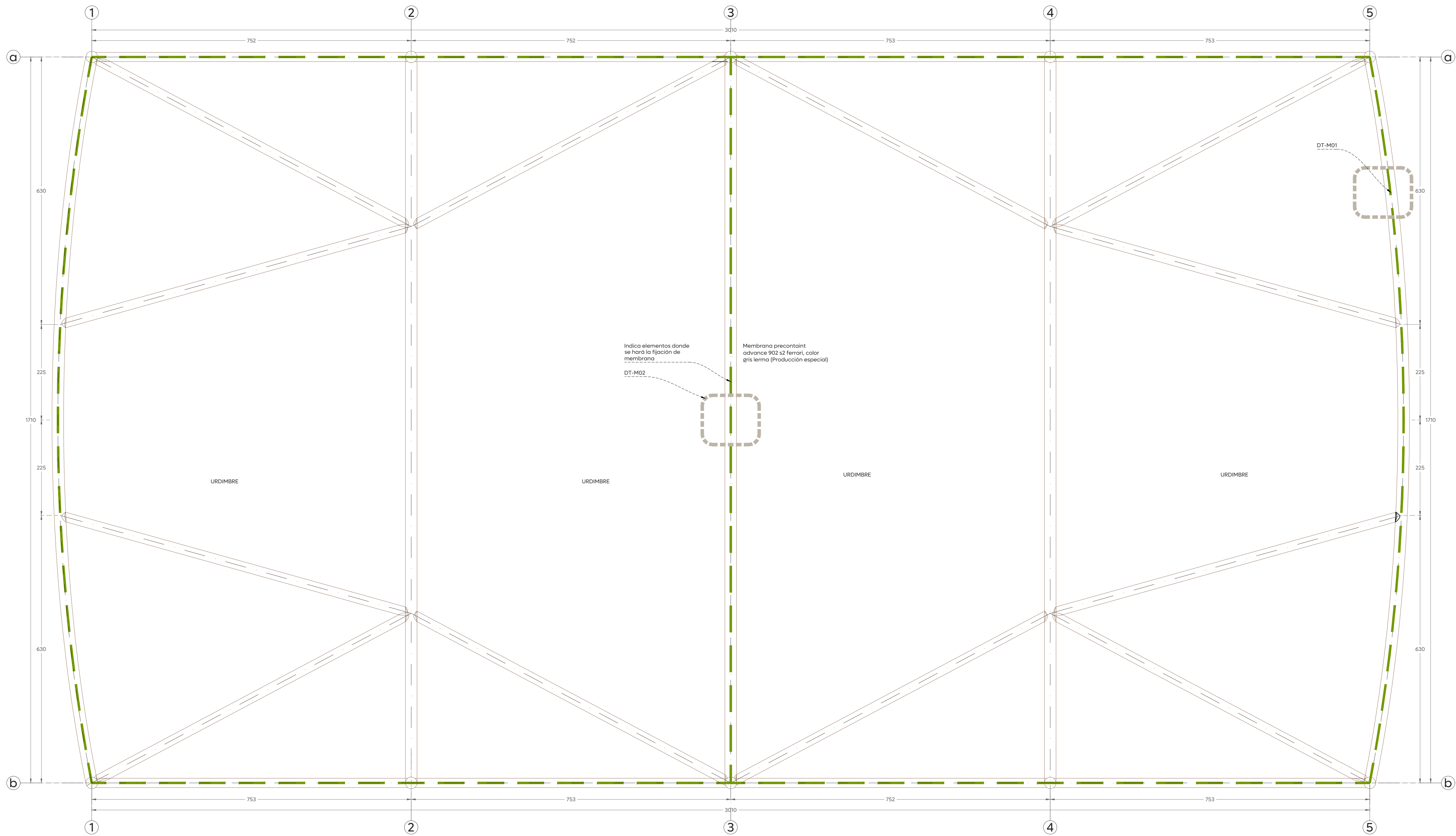
01 Planta de membrana Estructural cotas: cm Esc. 1:50
