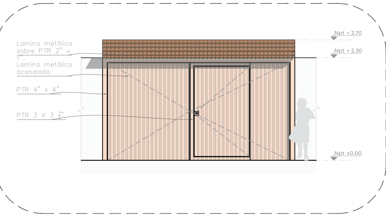
04 Puerta de ingreso Demoliciones y retiros 1:50
