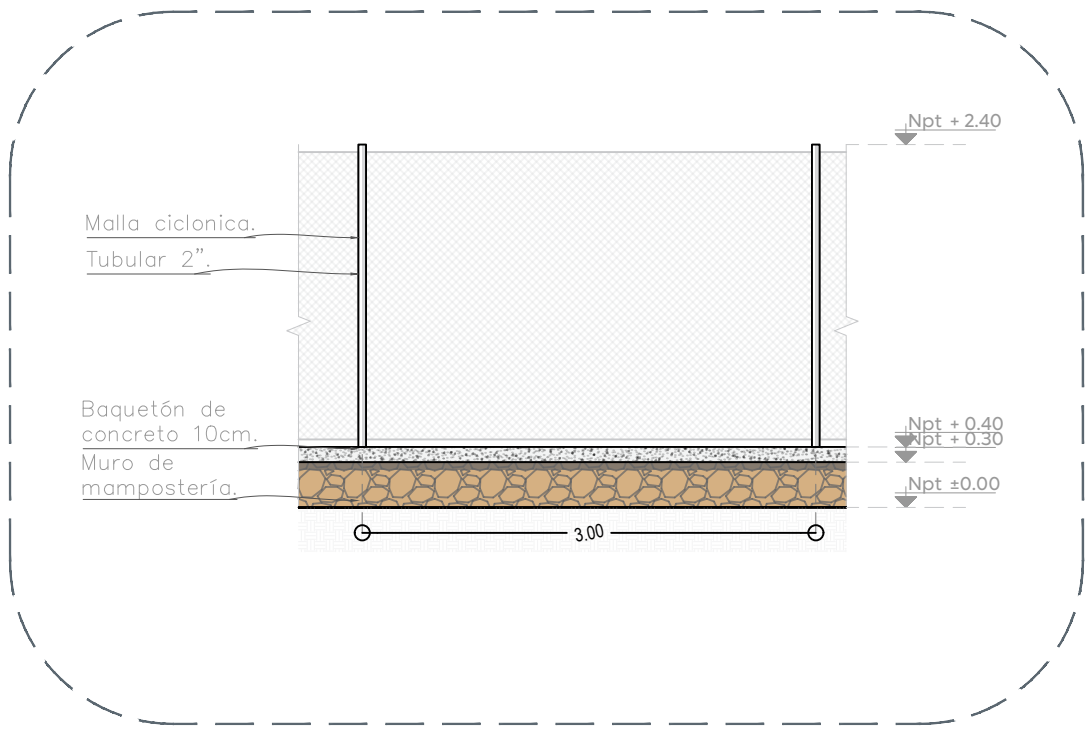
02 Reja perimetral Demoliciones y retiros 1:50
