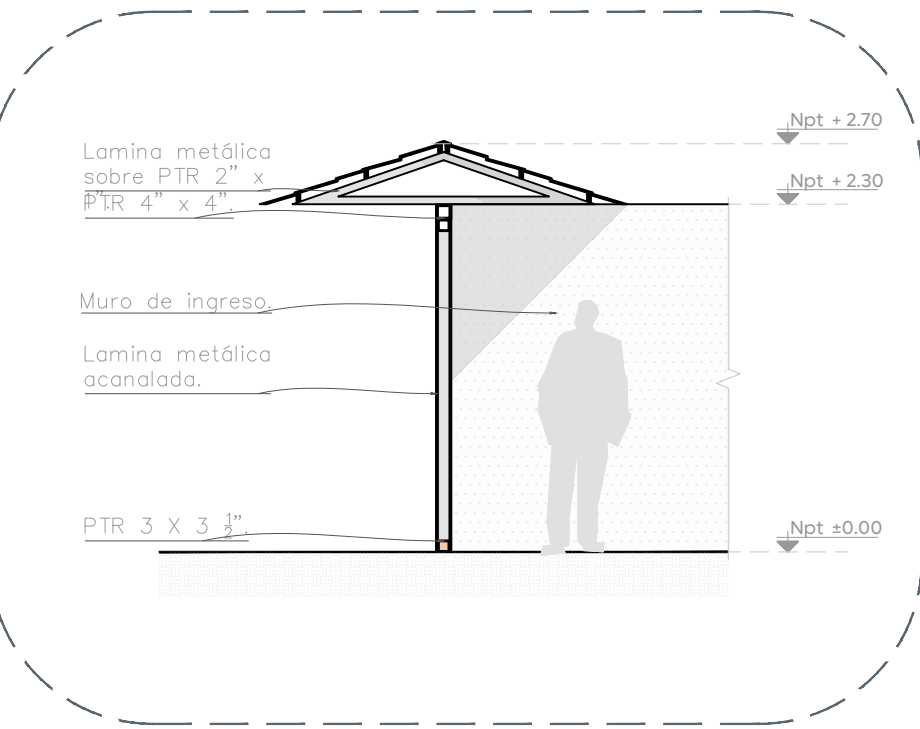
05 Cubierta en ingreso Demoliciones y retiros 1:50
