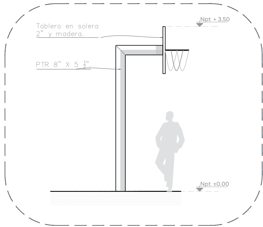
03 Tablero Demoliciones y retiros 1:50
