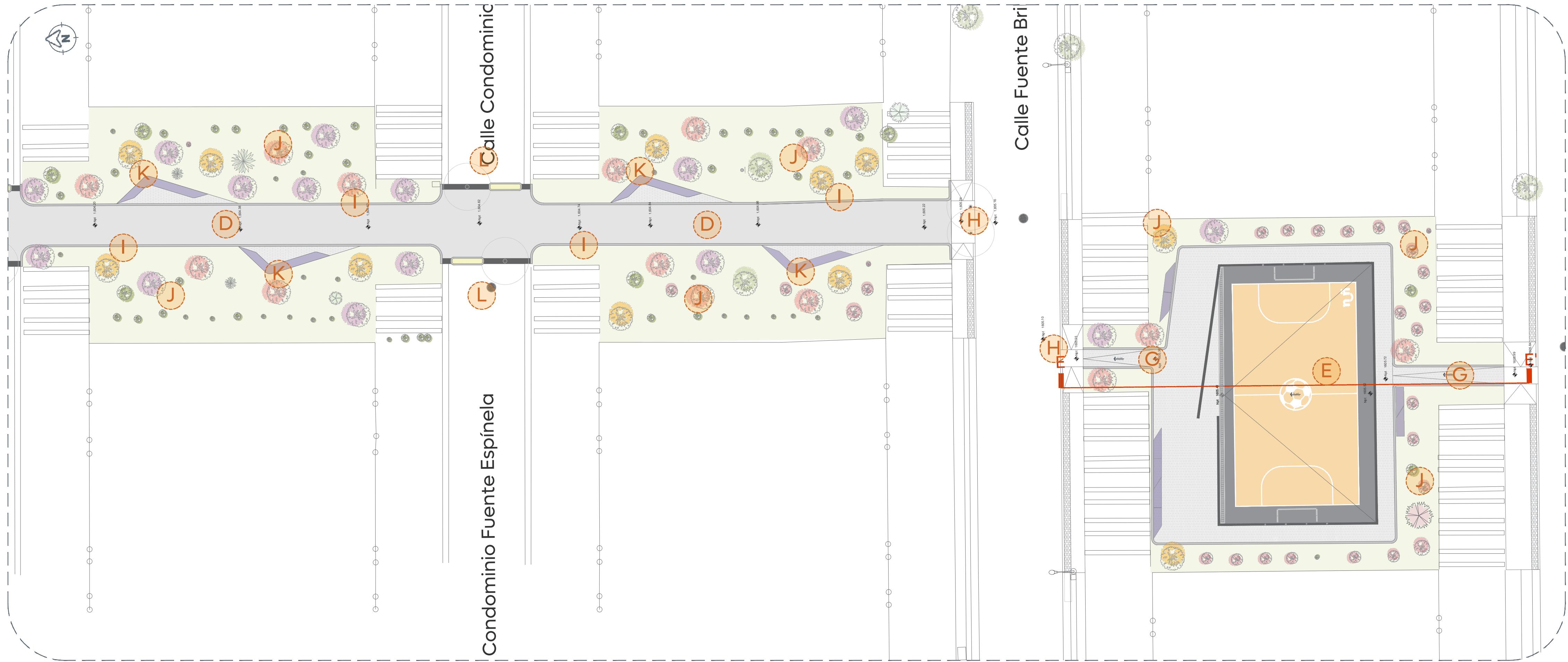
01 Planta de Conjunto Tramo 3 Alcances Generales 1:200
