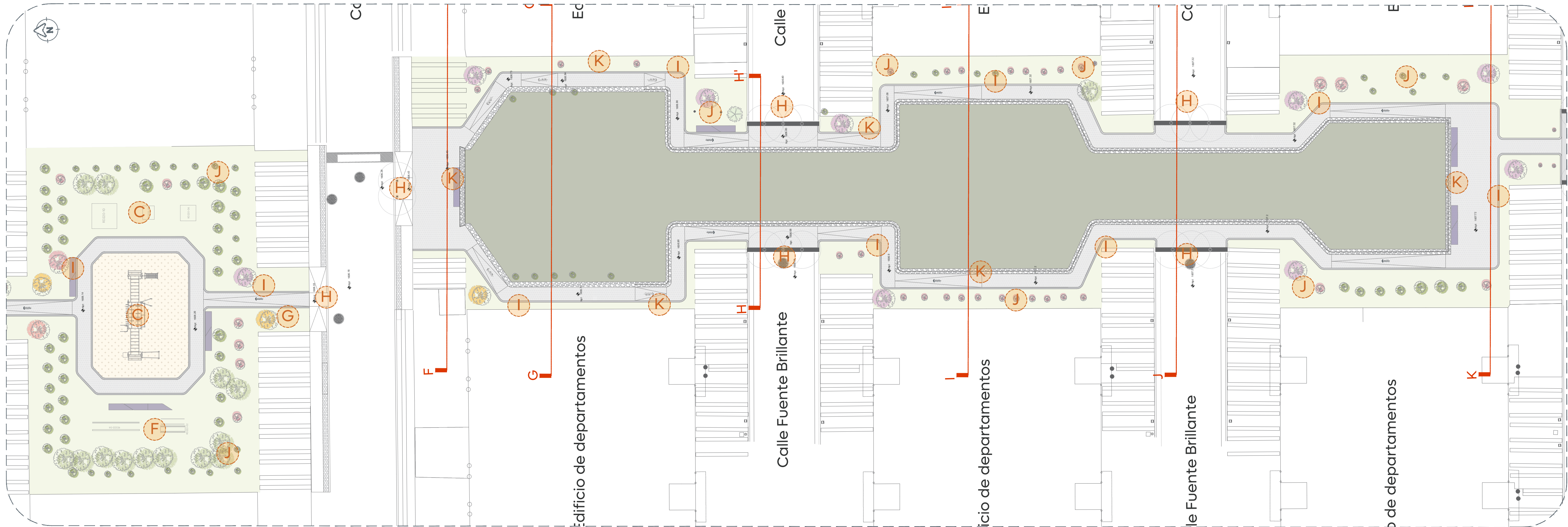
02 Planta de Conjunto Tramo 4 Alcances Generales 1:200
