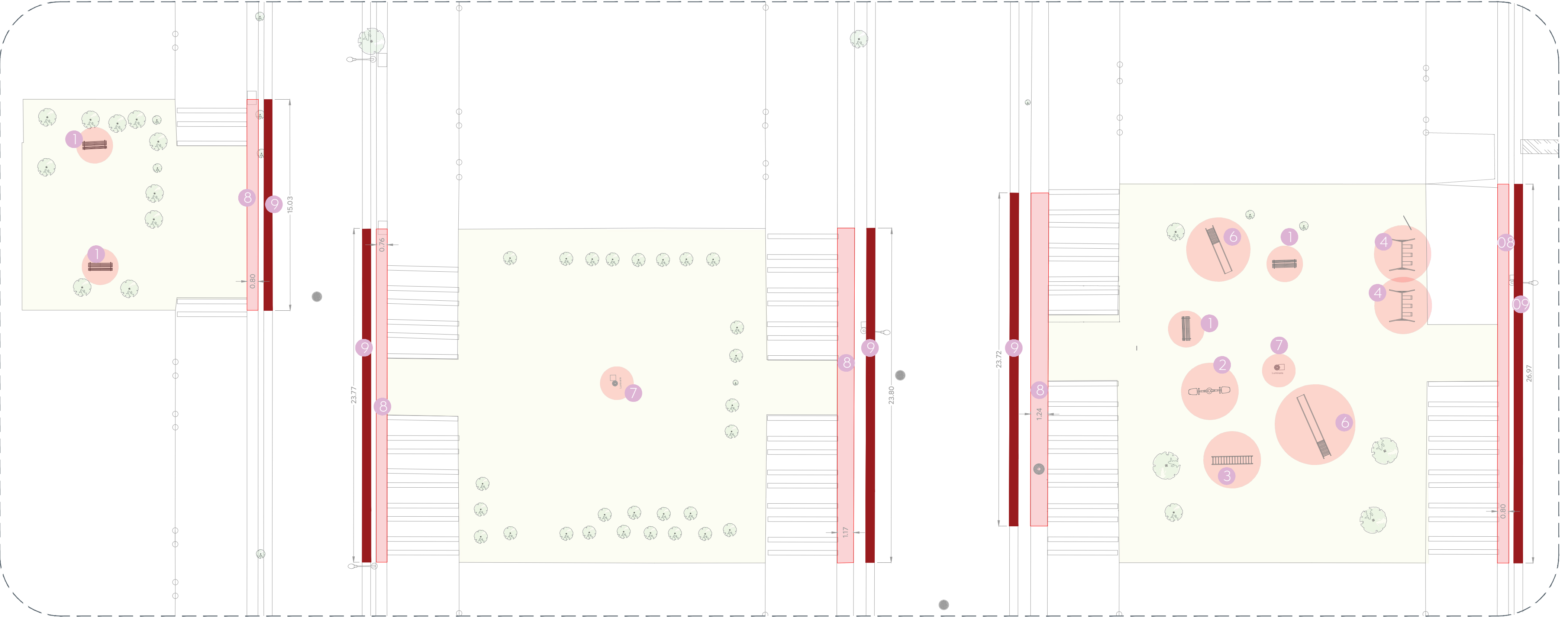
02 Planta de Conjunto Tramo 1 Demoliciones y desmontajes 1:200
