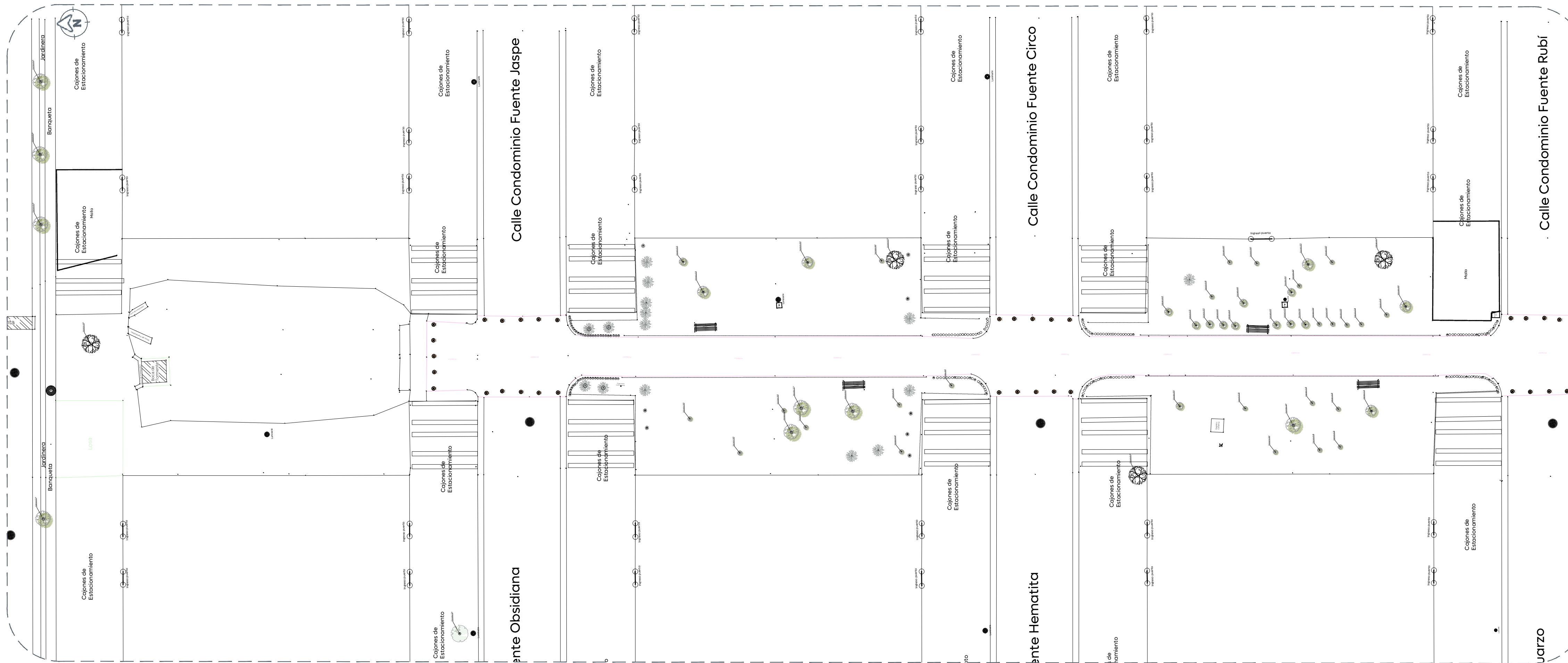
03 Planta de Conjunto Tramo 2 Topografía 1:200
