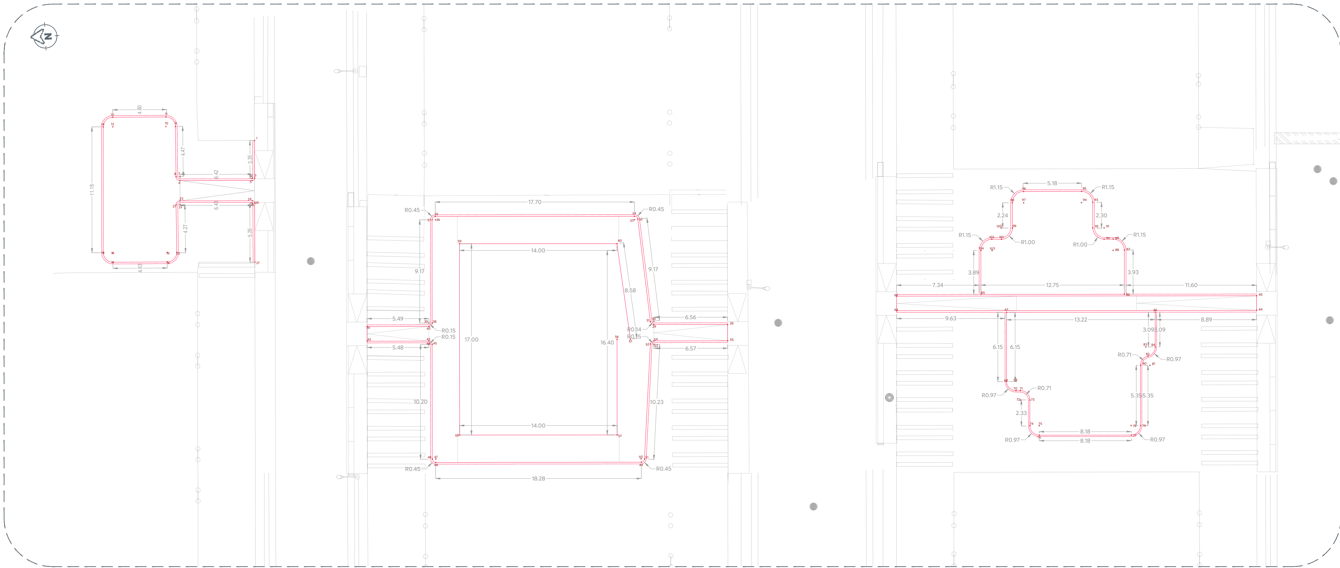
02 Planta de Conjunto Tramo 1 Trazo General
