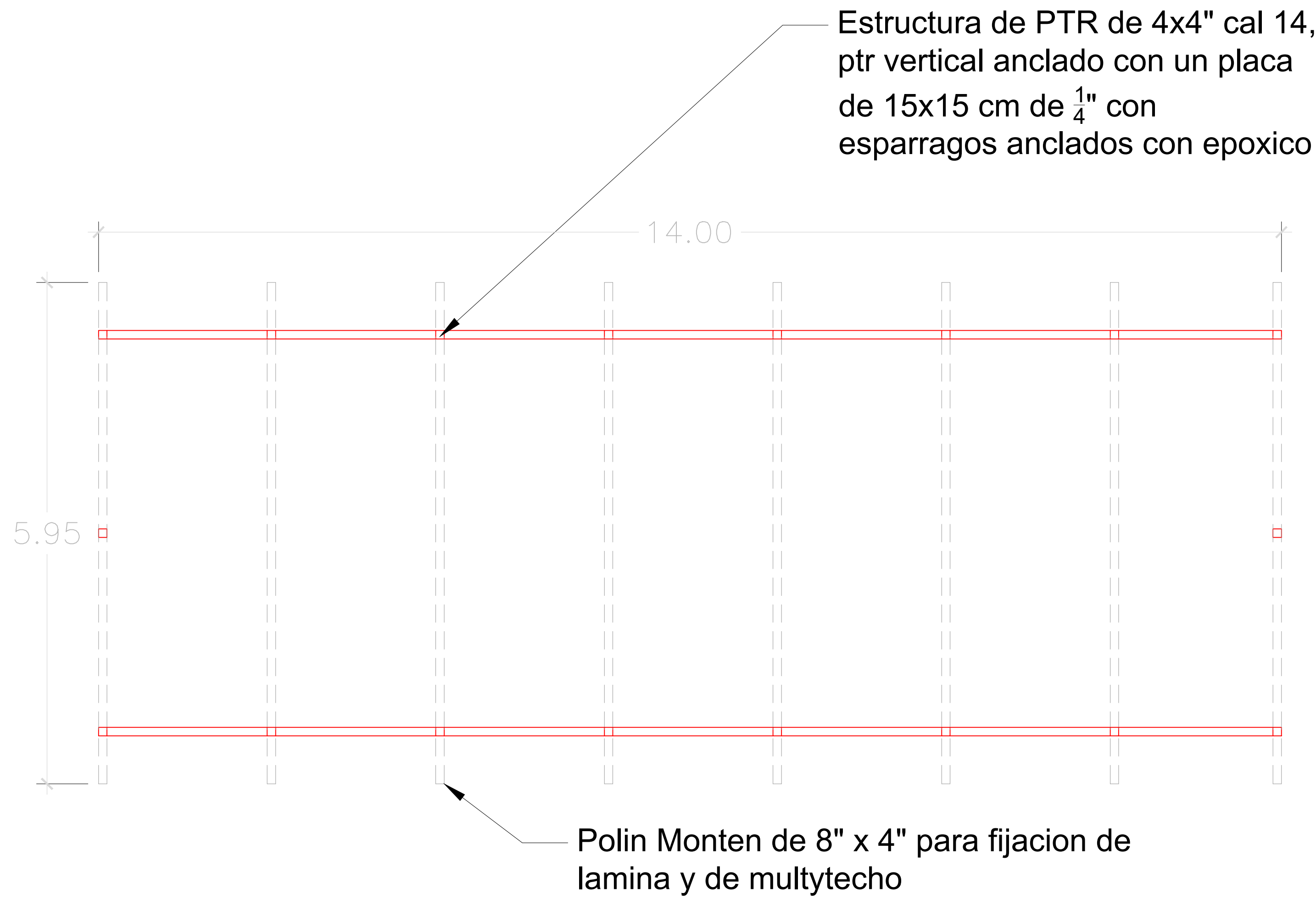
01 DETALLE ESTRUCTURA ESC. 1:125
