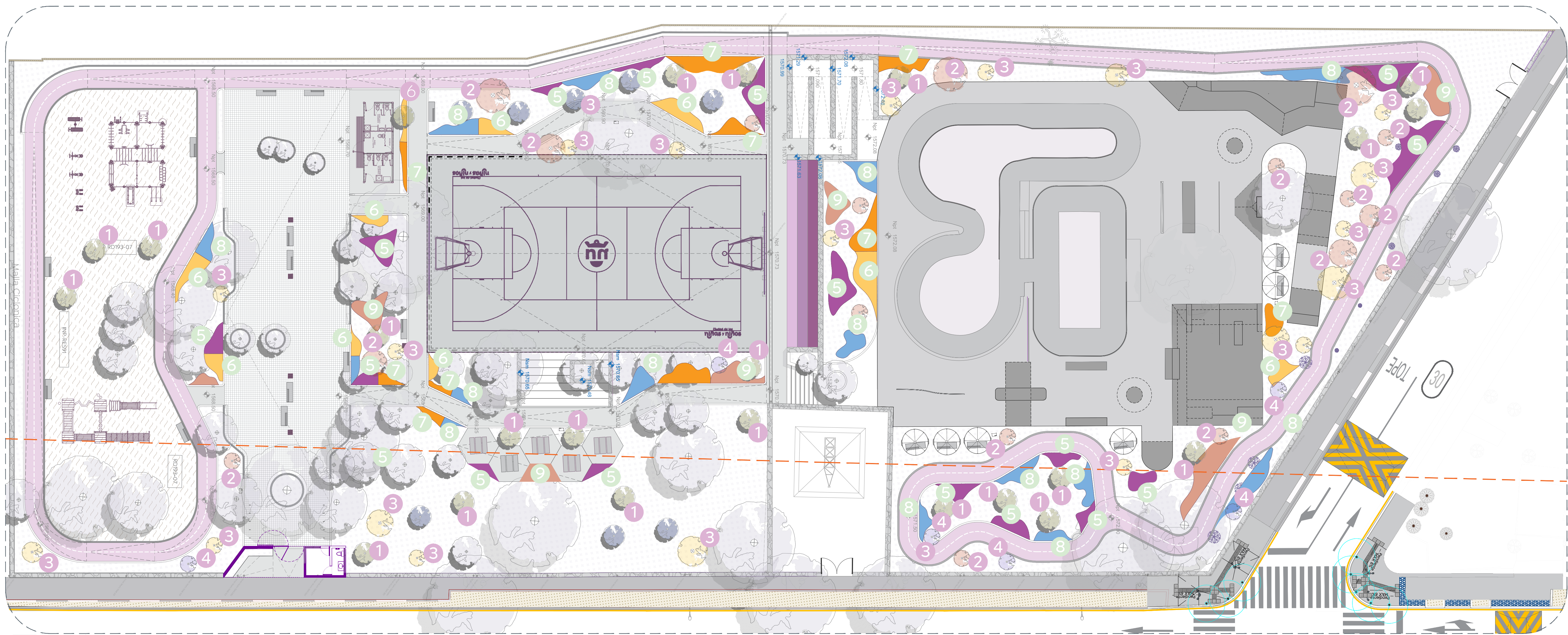
01 Planta de Conjunto Alcances generales 1:200
