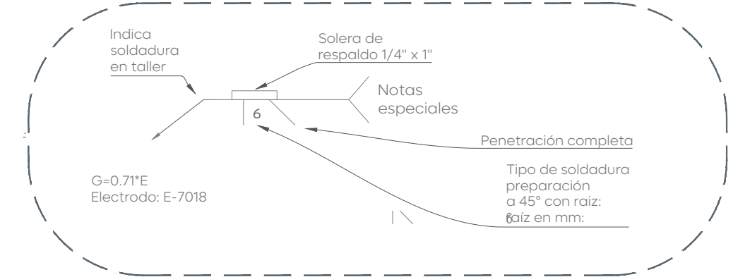
06 Simbología de soldadura
