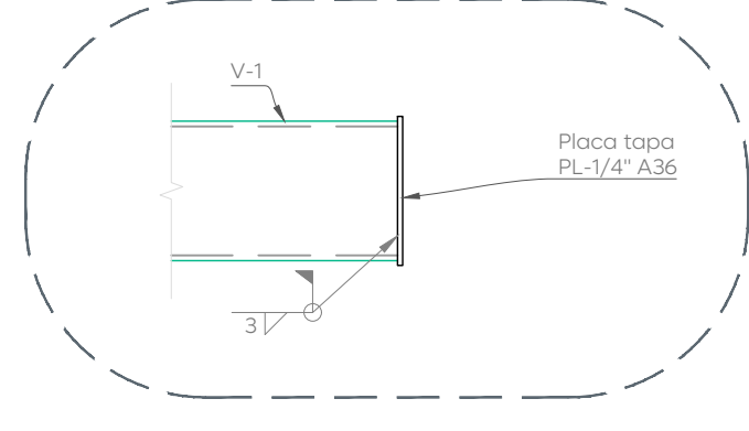
08 Placas tapa de extremo
