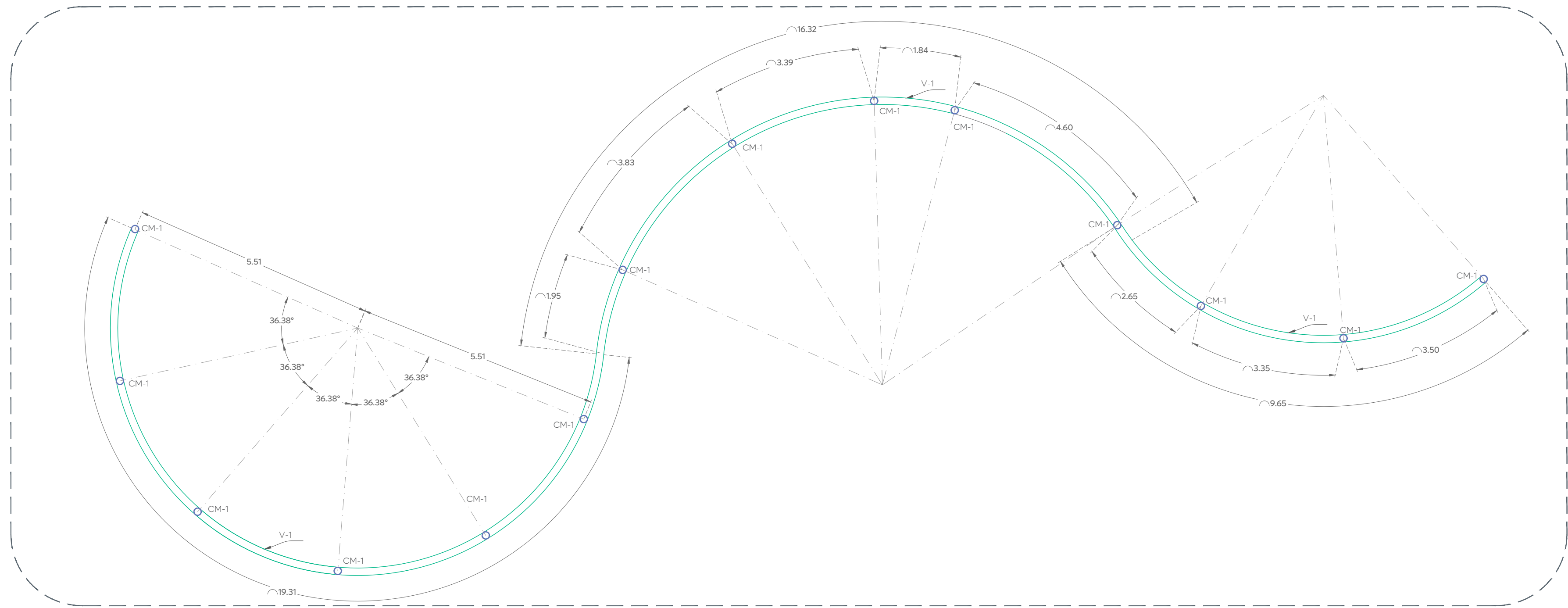
02 Estructura juego - planta de estructura (NTEM+2.80)
