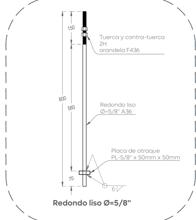
15 Anclas, AN-1
