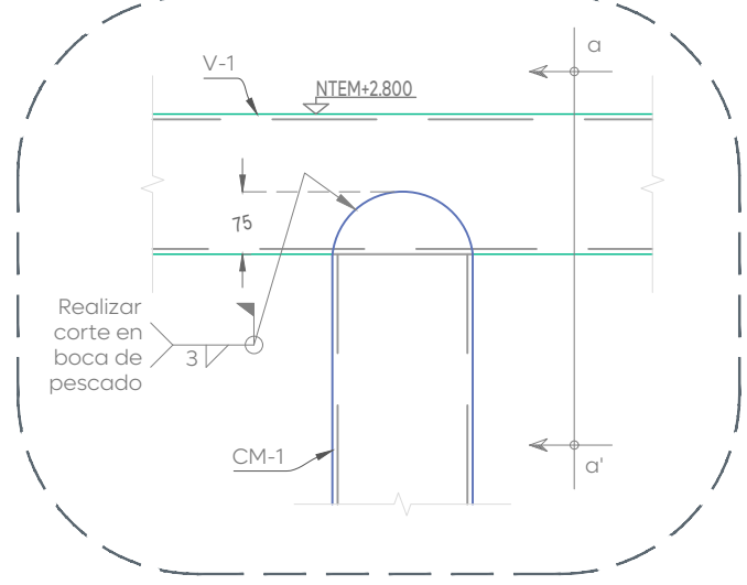
11 Conexión tipo viga-columna
