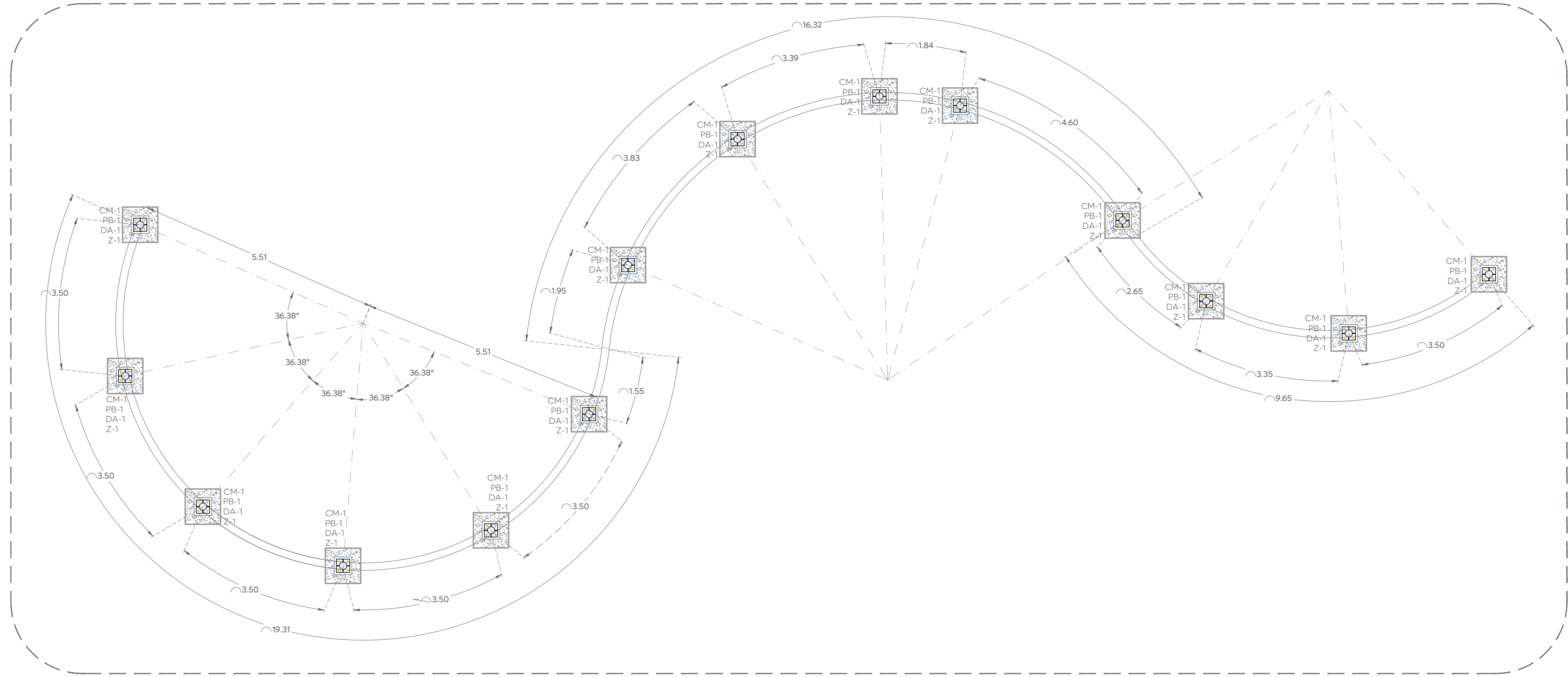
01 Estructura juego - planta de cimentación (NDZ - 1.15)
