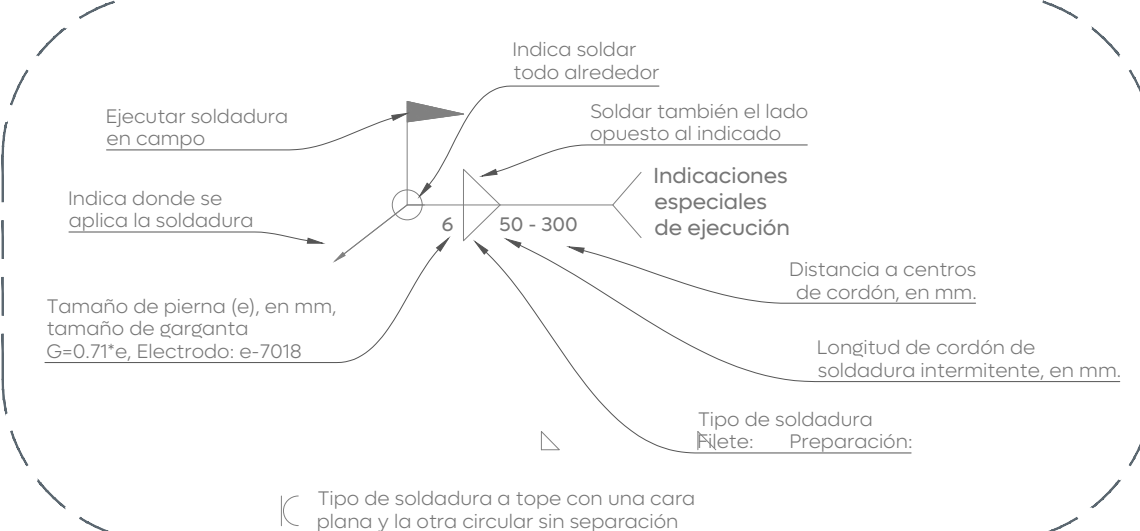
05 Simbología de soldadura
