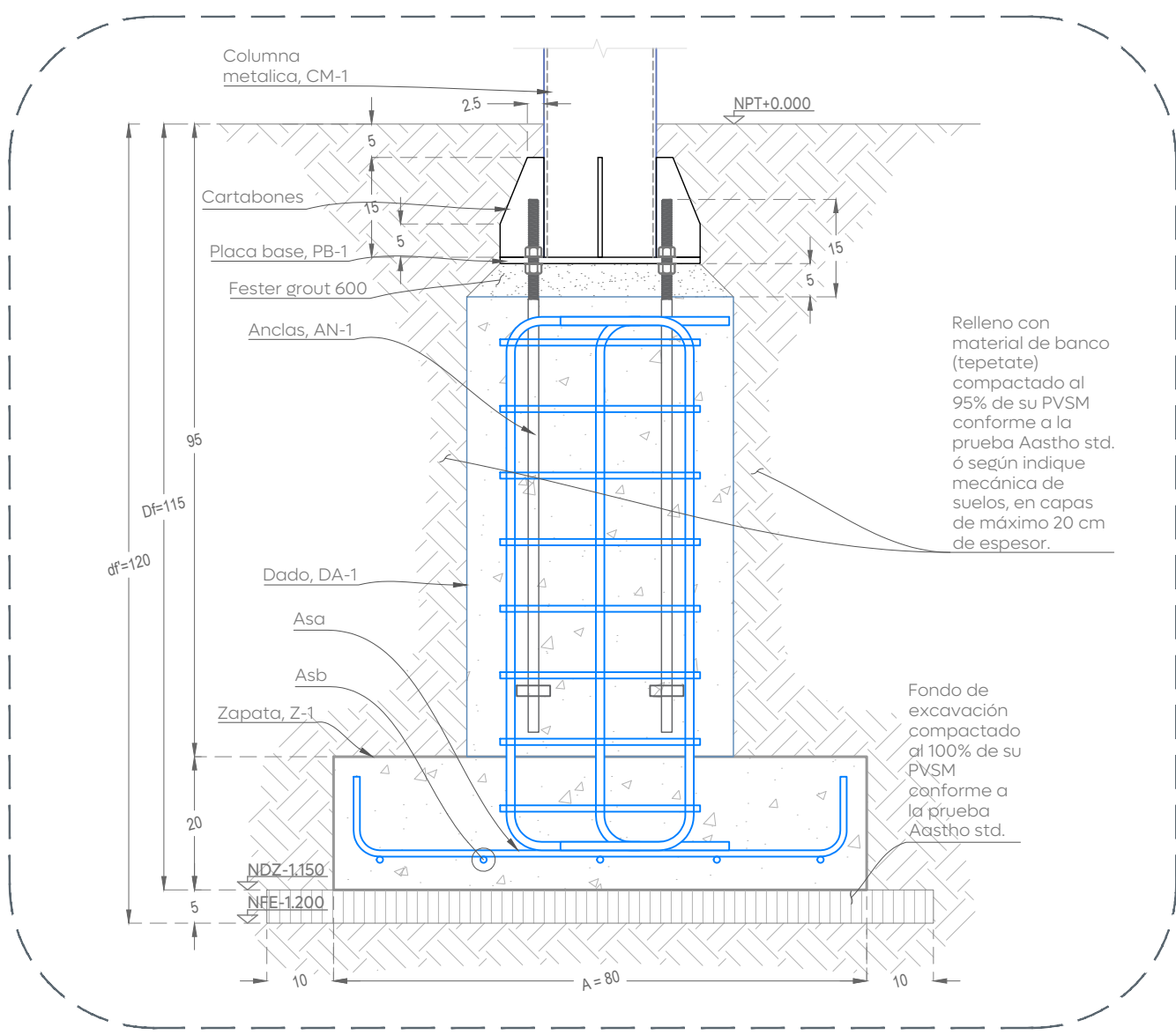
04 Desplante de zapatas
