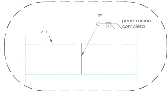
07 Empate tipo de vigas
