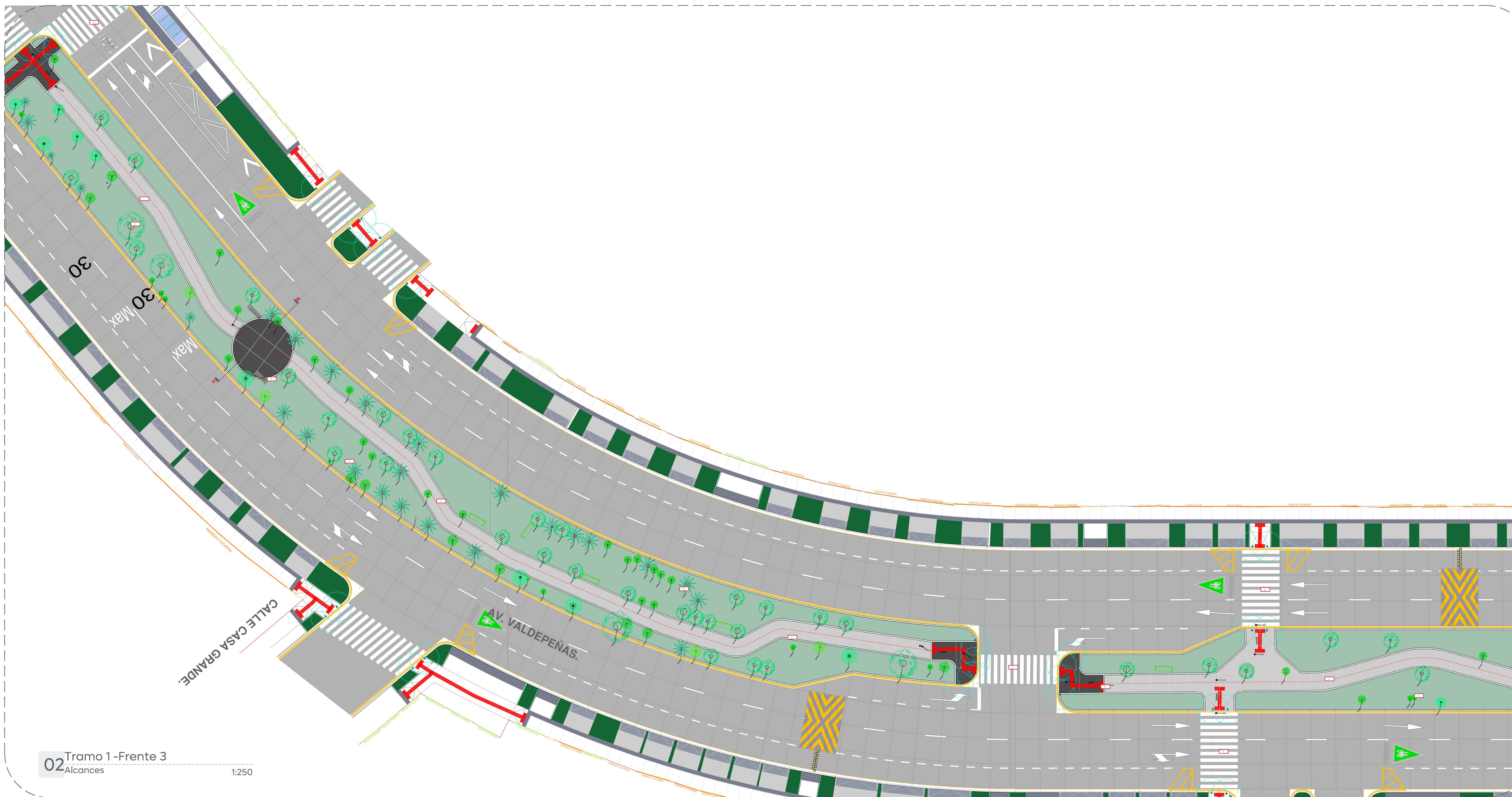
01 Plano llave conjunto - frente 3 Alcances 1:1200
