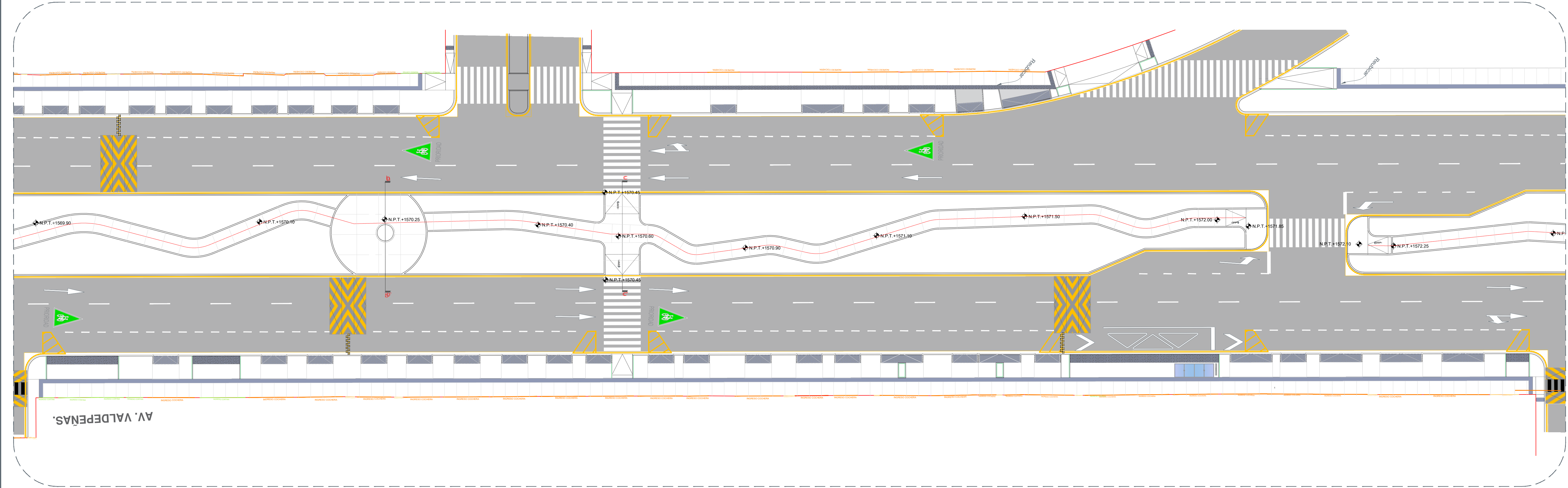
02 Planta de Conjunto | Tramo 2 - Frente 3 Nivelación 1:250
