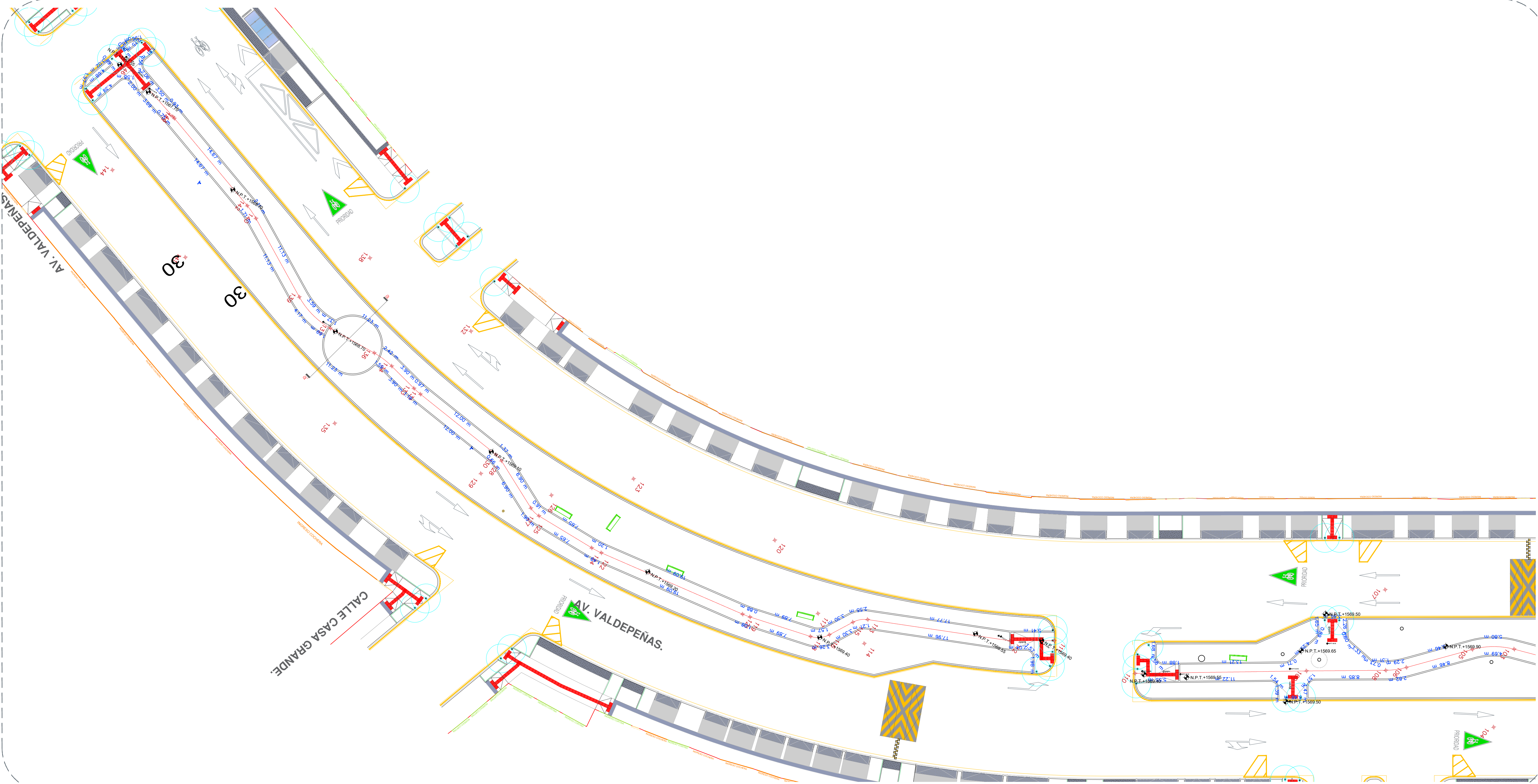
02 Planta de Conjunto | Tramo 1 - Frente 3 Trazo 1:250
