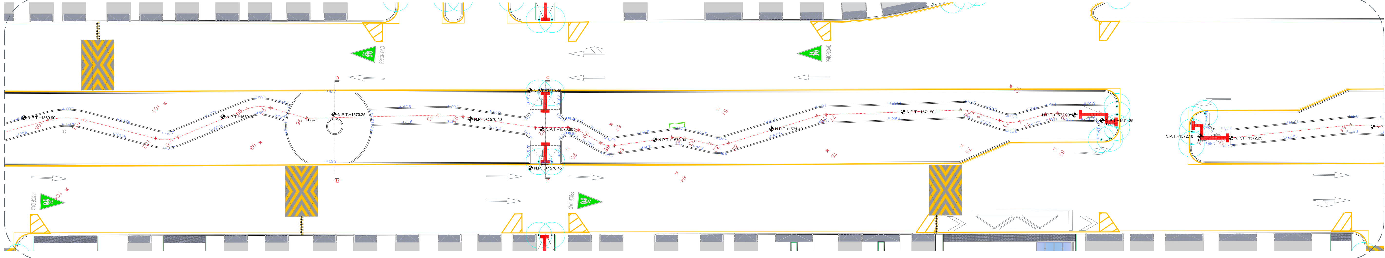
02 Planta de Conjunto | Tramo 2 - Frente 3 Trazo 1:250
