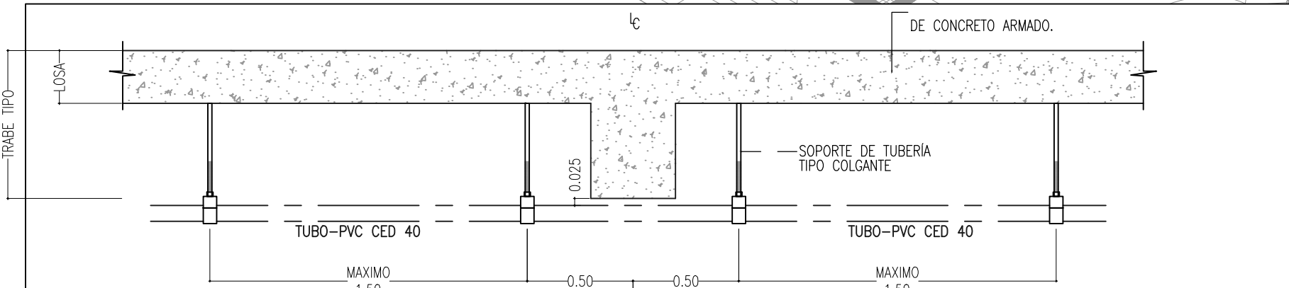
DETALLE DE MONTAJE LINEA PRINCIPAL
