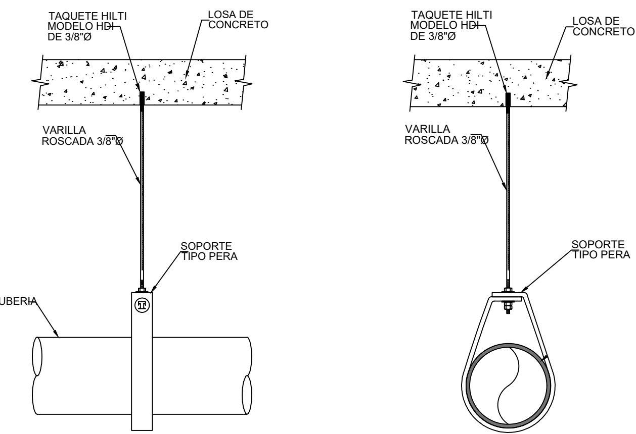
DETALLES DE LA SOPORTERIA TIPO COLGANTE
