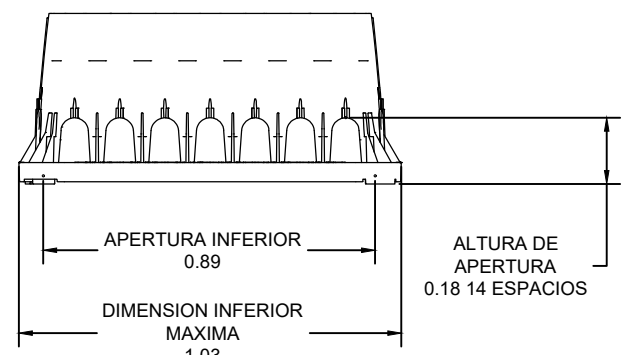
CAJA DE VÁLVULAS MAXI JUMBO SIN ESCALA
