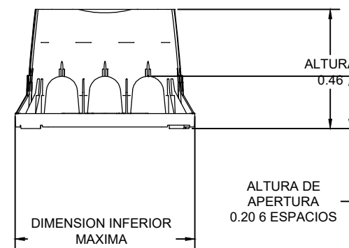
CAJA DE VÁLVULAS MAXI JUMBO SIN ESCALA
