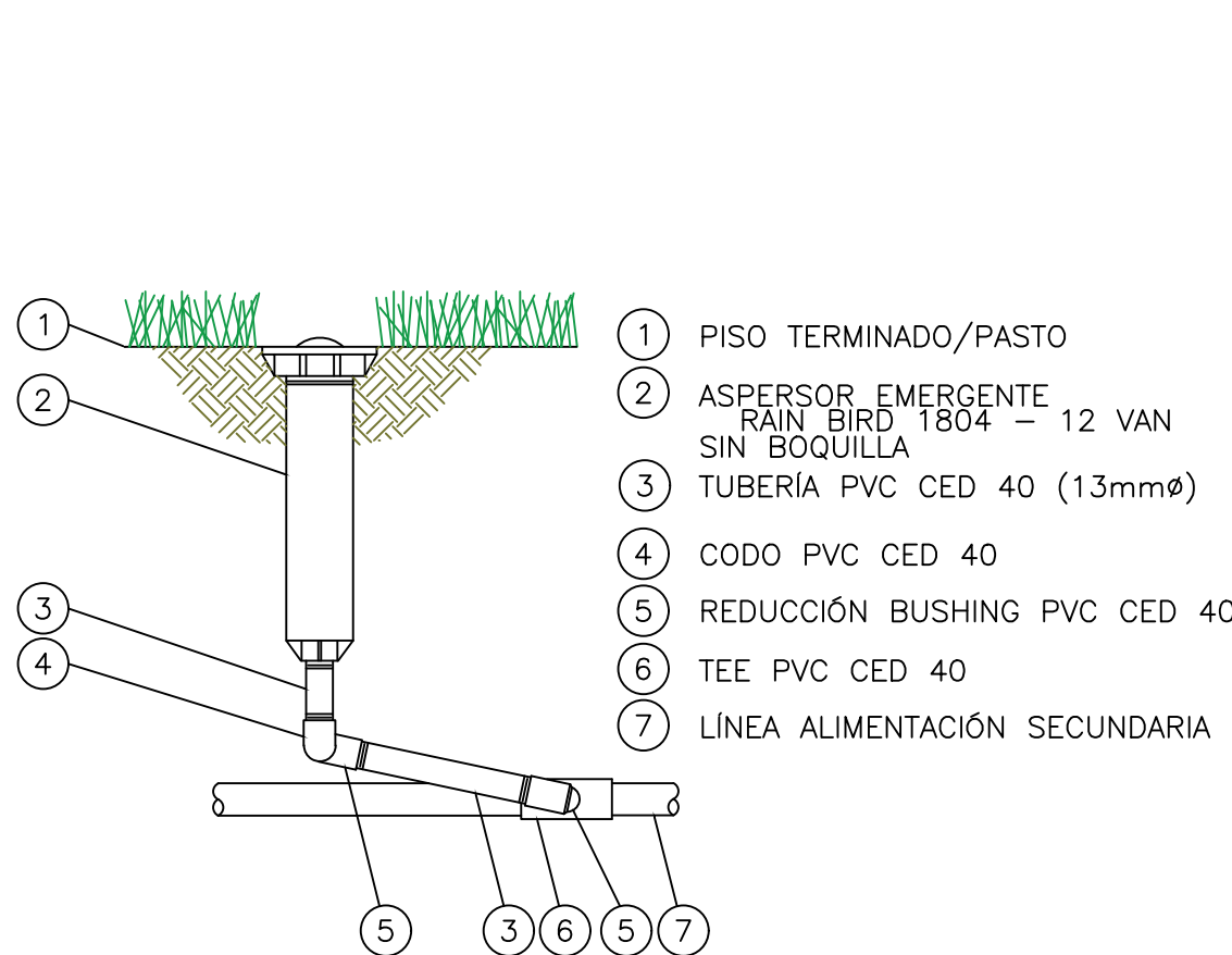
CONEXION ASPIRSOR SIN ESCALA
