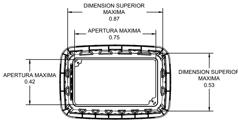
CAJA DE VÁLVULAS MAXI JUMBO SIN ESCALA
