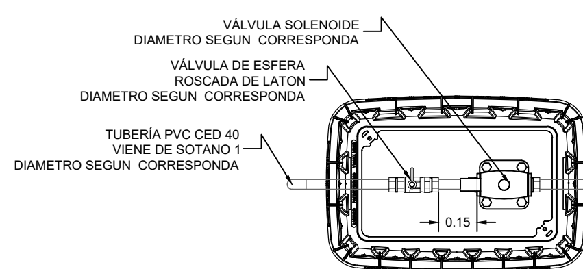
ARREGLO EN CAJA DE VÁLVULAS SIN ESCALA
