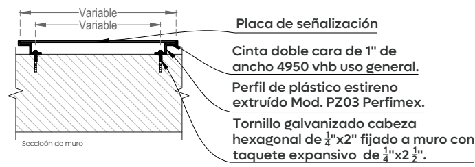
03 SÑ-01 Fijación en superficies irregulares Esc. 1:10
