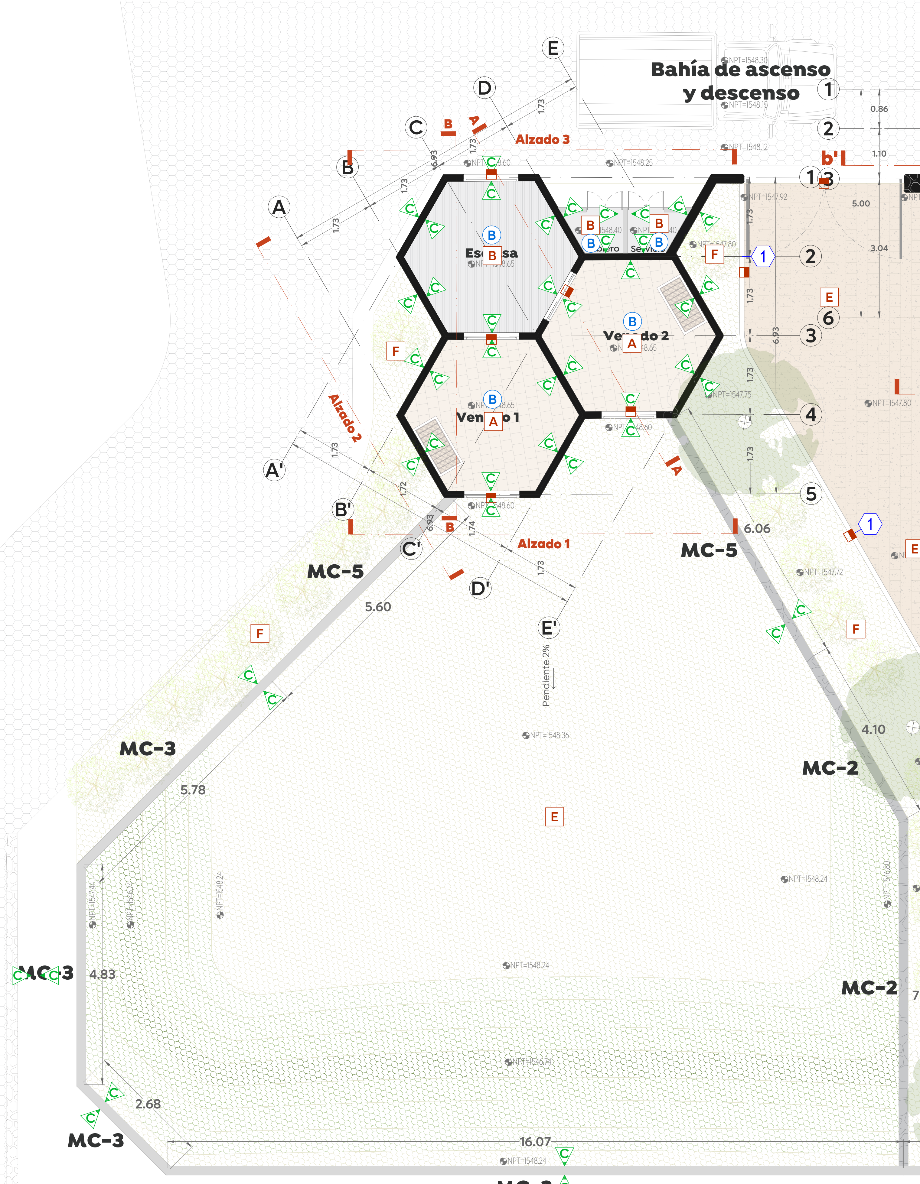
01 Planta de acabados Hábitat de venados Esc. 1:50
