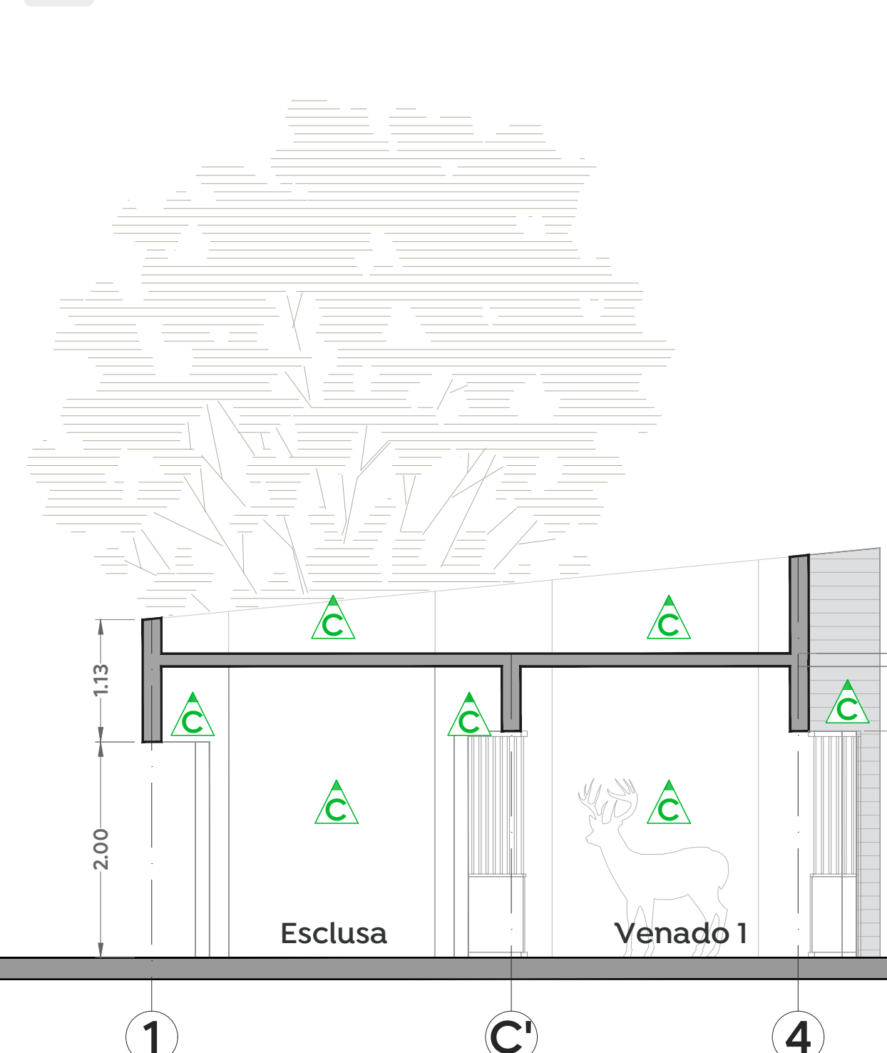
05 Sección A-A de acabados Venados Esc. 1:50
