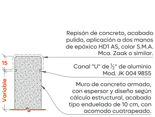
07 DT-02 Detalle de repisón Esc. 1:25
