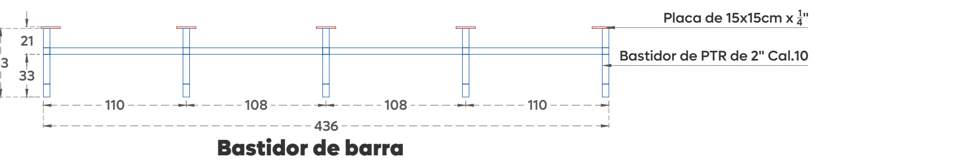
14 DT-05 Detalle de jardineras Esc. 1:25
