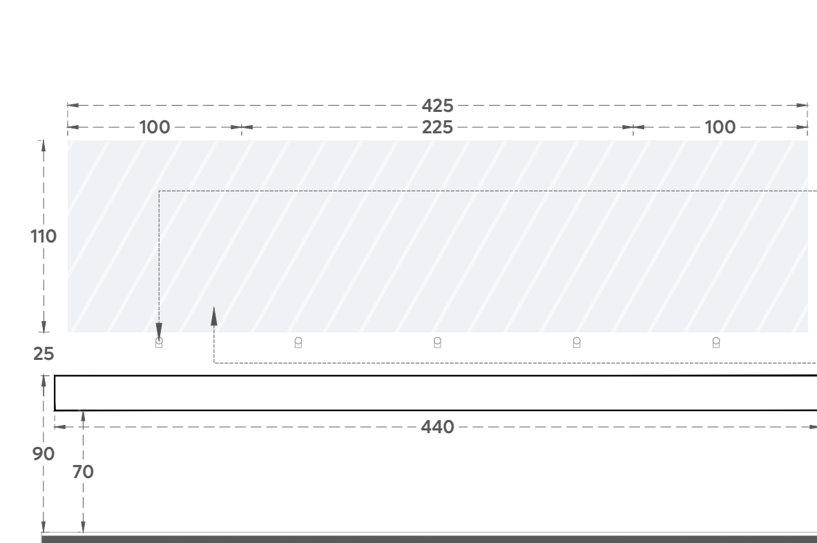
16 DT-07 Detalle de repisón Esc. 1:25
