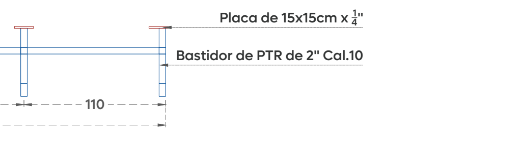
14 DT-05 Detalle de jardineras Esc. 1:25
