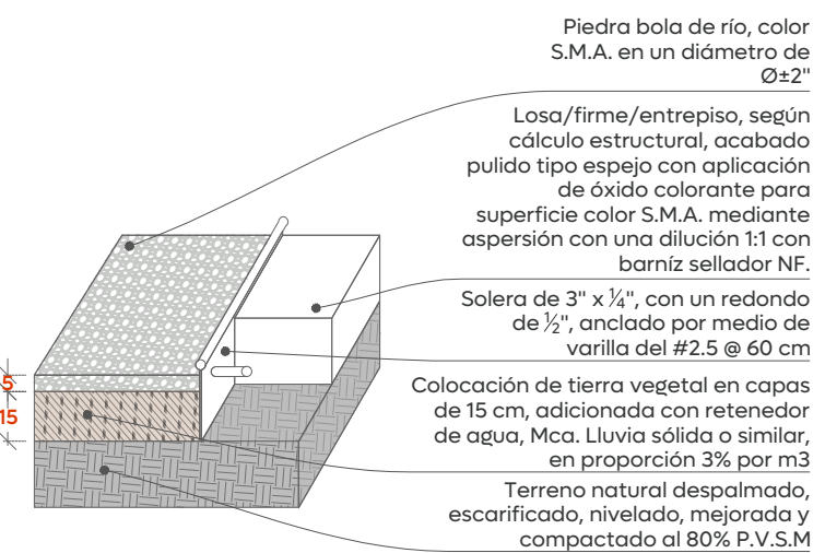
11 DT-05 Detalle de jardineras Esc. 1:25
