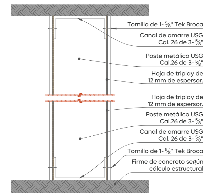
10 DT-06 Detalle de acabado en muro tablayeso Esc. 1:25
