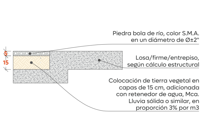
08 DT-03 Detalle de losa/firme Esc. 1:25
