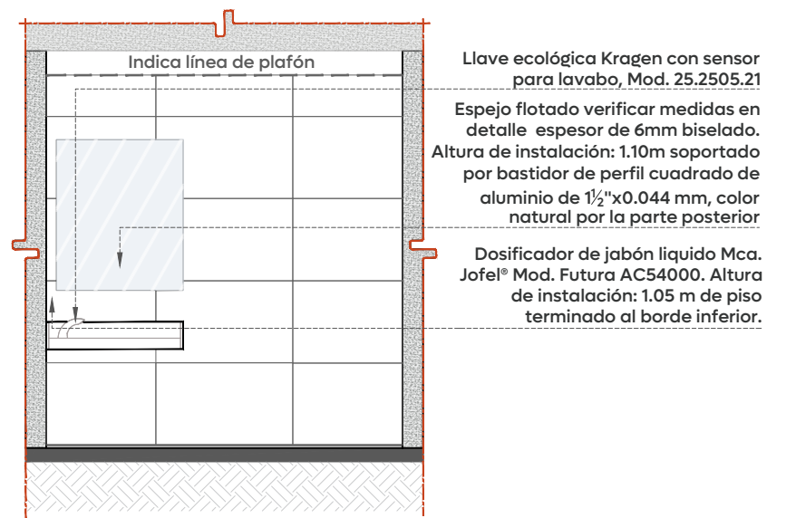
13 DT-04 Detalle remate de muro lambrín Esc. 1:25
