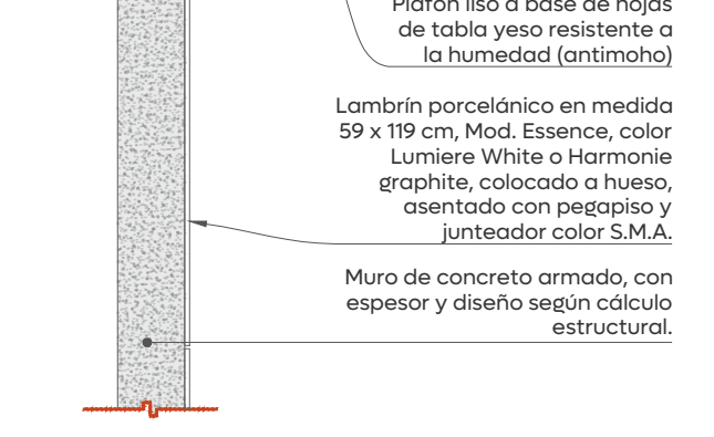
09 DT-04 Detalle remate de muro lambrín Esc. 1:25
