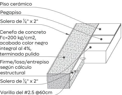
06 DT-01 Detalle de Cenefa Esc. 1:25
