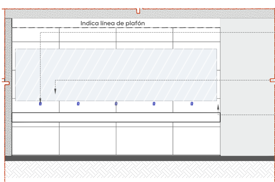
12 DT-03 Detalle de losa/firme Esc. 1:25
