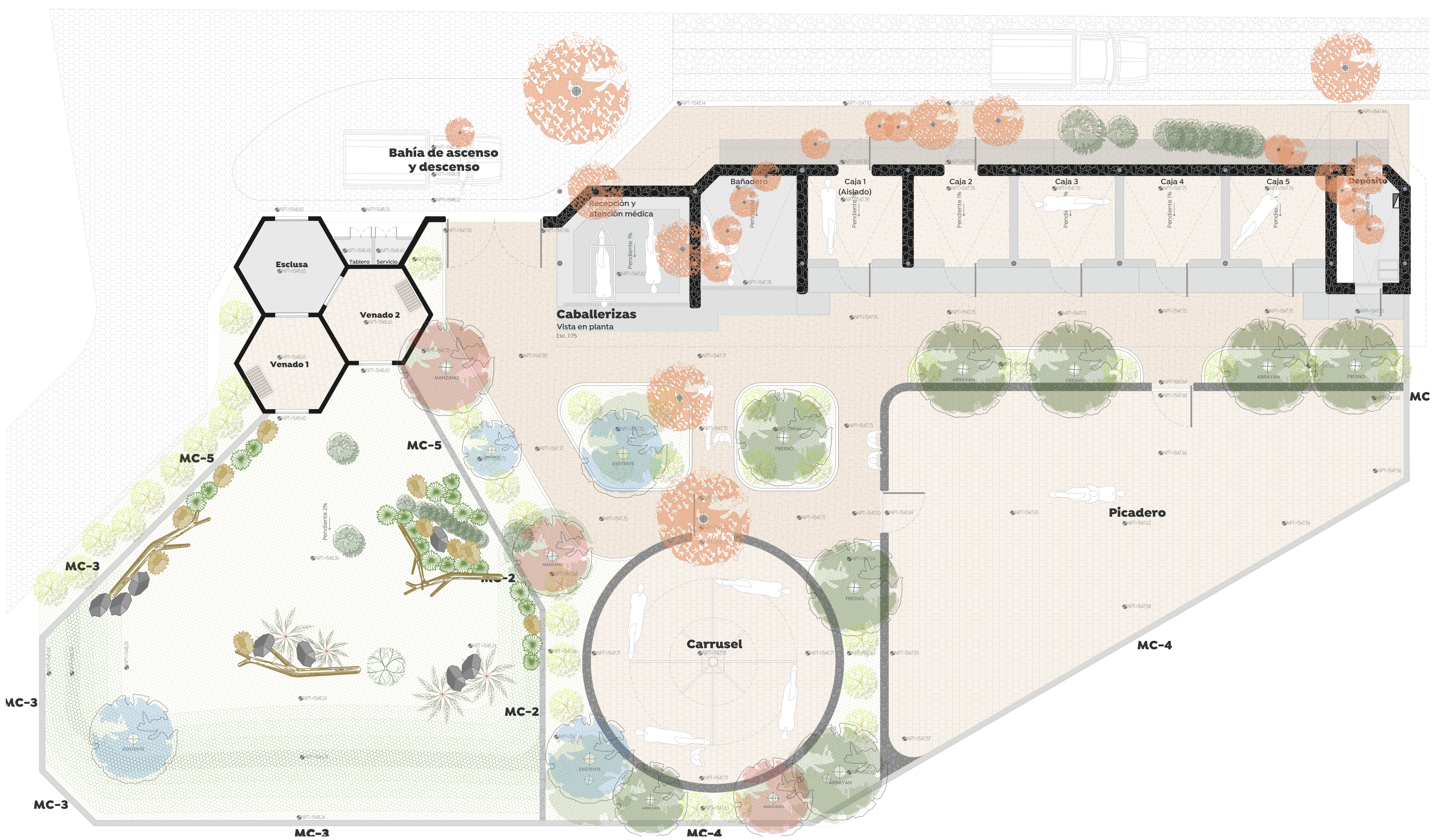
01 Planta de vegetación Hábitat de venados y caballerizas Esc. 1:75
