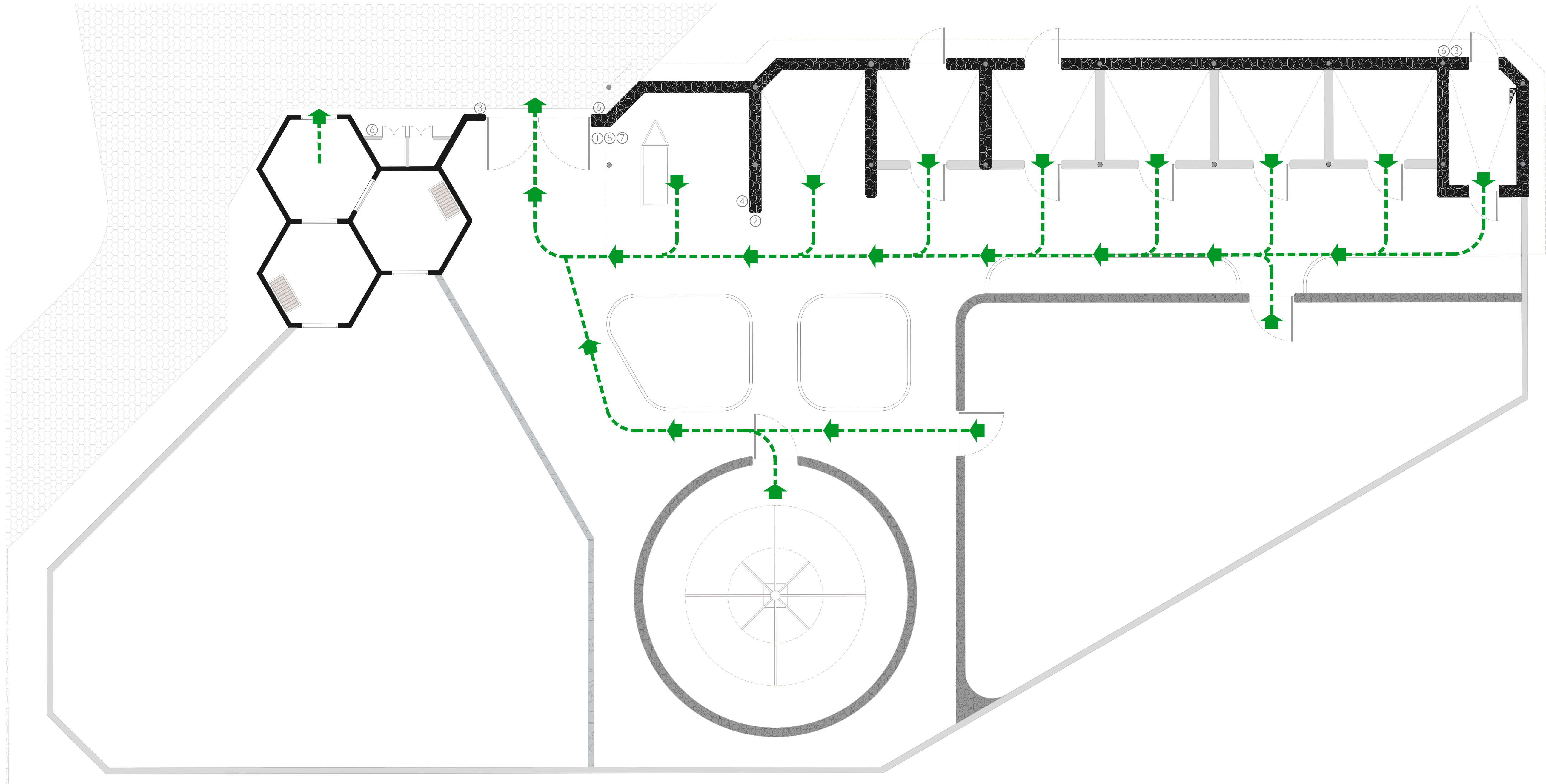
01 Planta de hábitat de venados y caballerizas Ubicación de señalética y ruta de evacuación Esc. 1:75
