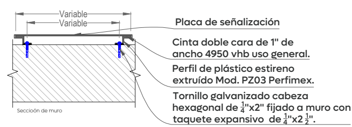
04 SÑ-01 Fijación en superficies irregulares Esc. 1:10
