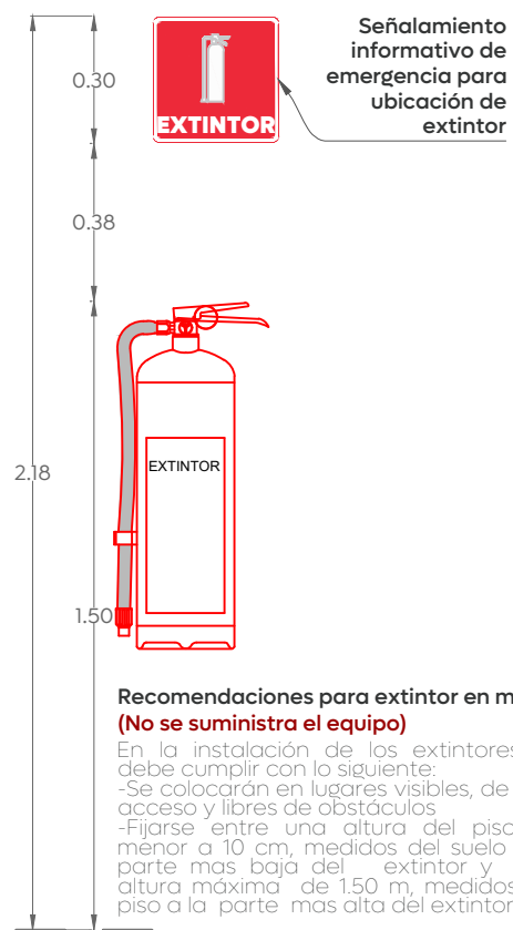
03 Extintores Recomendaciones Esc. 1:20
