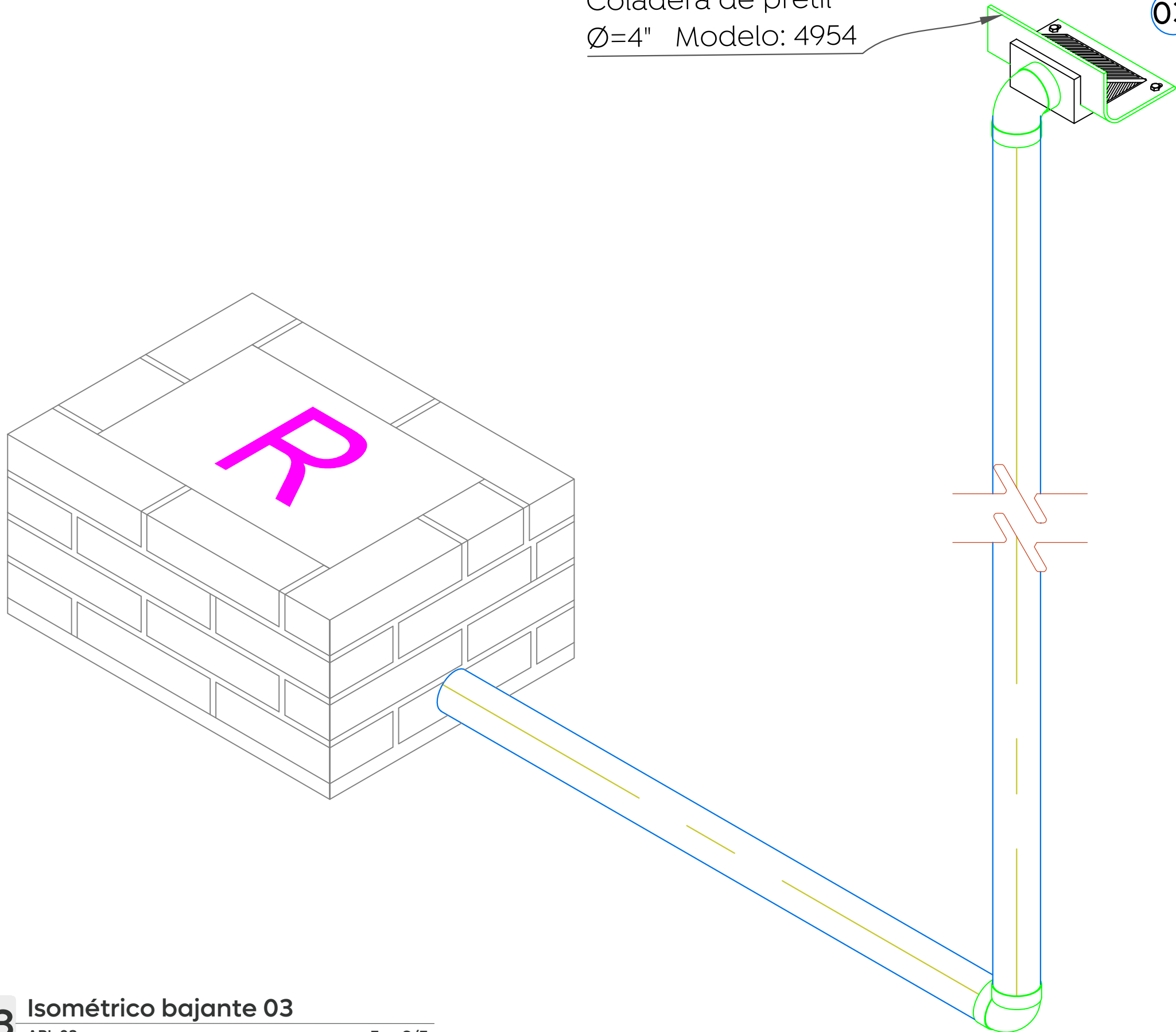
03 Isométrico bajante 03 APL.03 Esc. S/E
