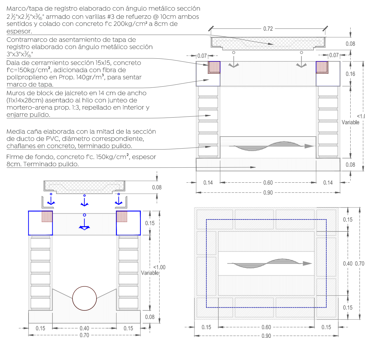
02 Detalle de registro (Menor a 1 m.)
