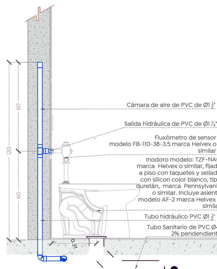
Instalaciones de inodoro
