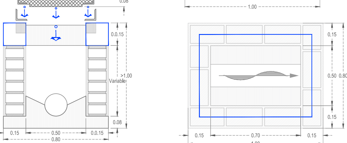
01 Detalle de registro (Mayor a 1 m.)
