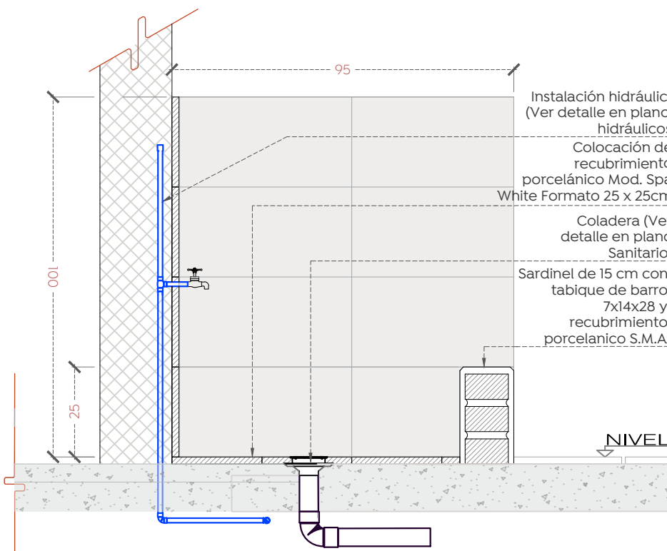
Instalaciones de vertedero
