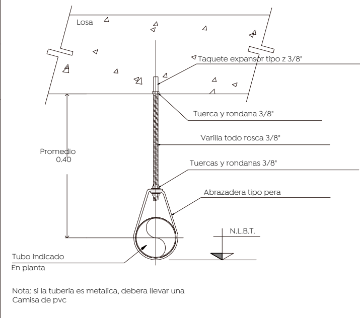
Detalle de soporteria tipo pera para tubería horizontal
