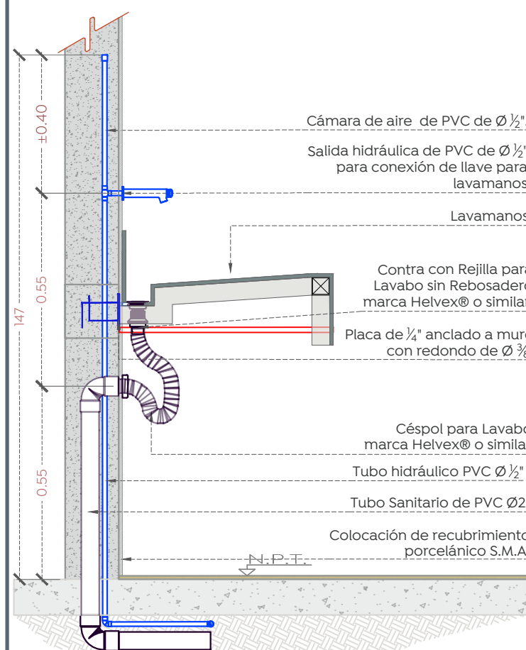
Instalaciones de lavamanos
