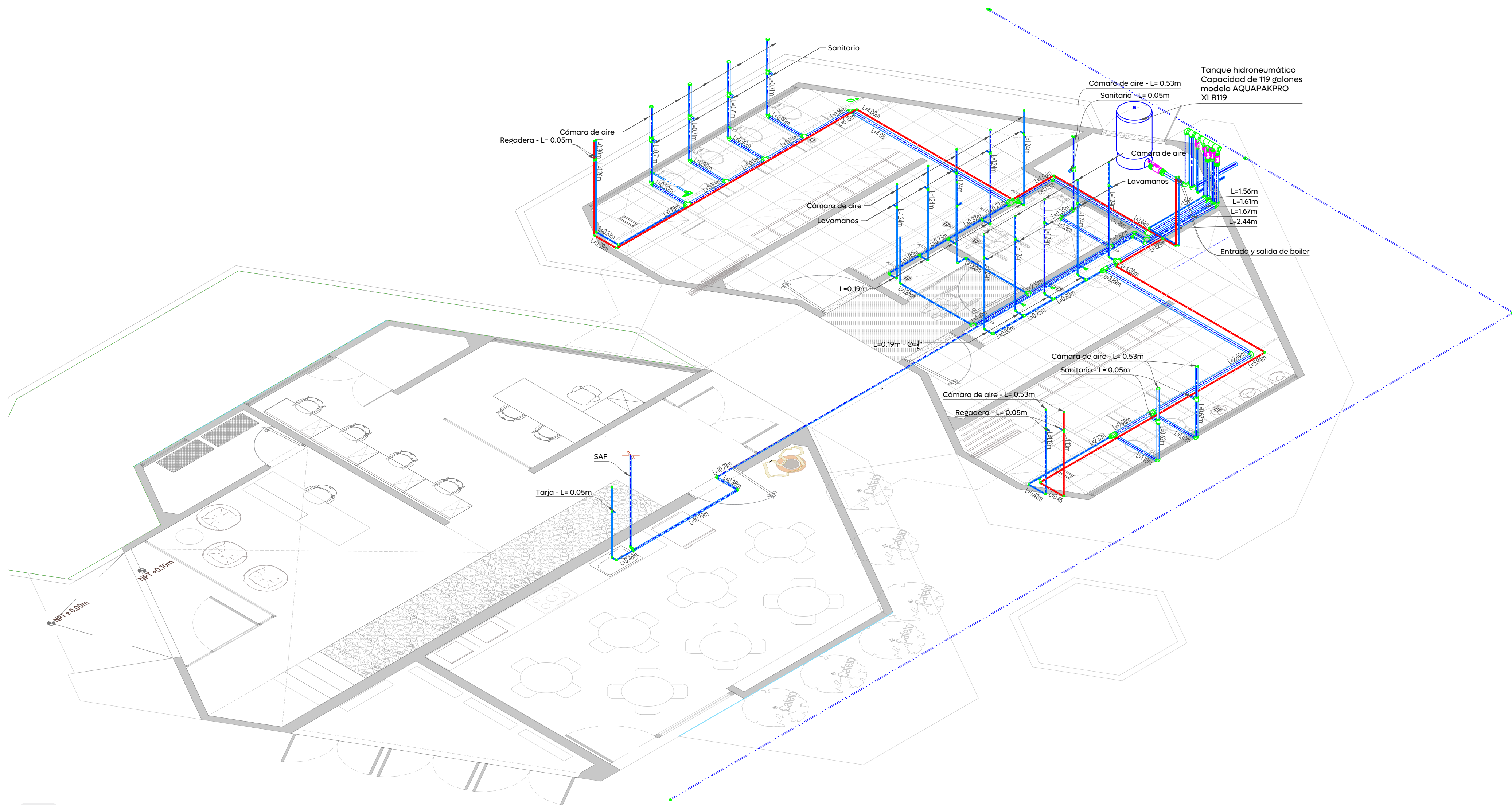
05 Isométrico planta baja APO.03
