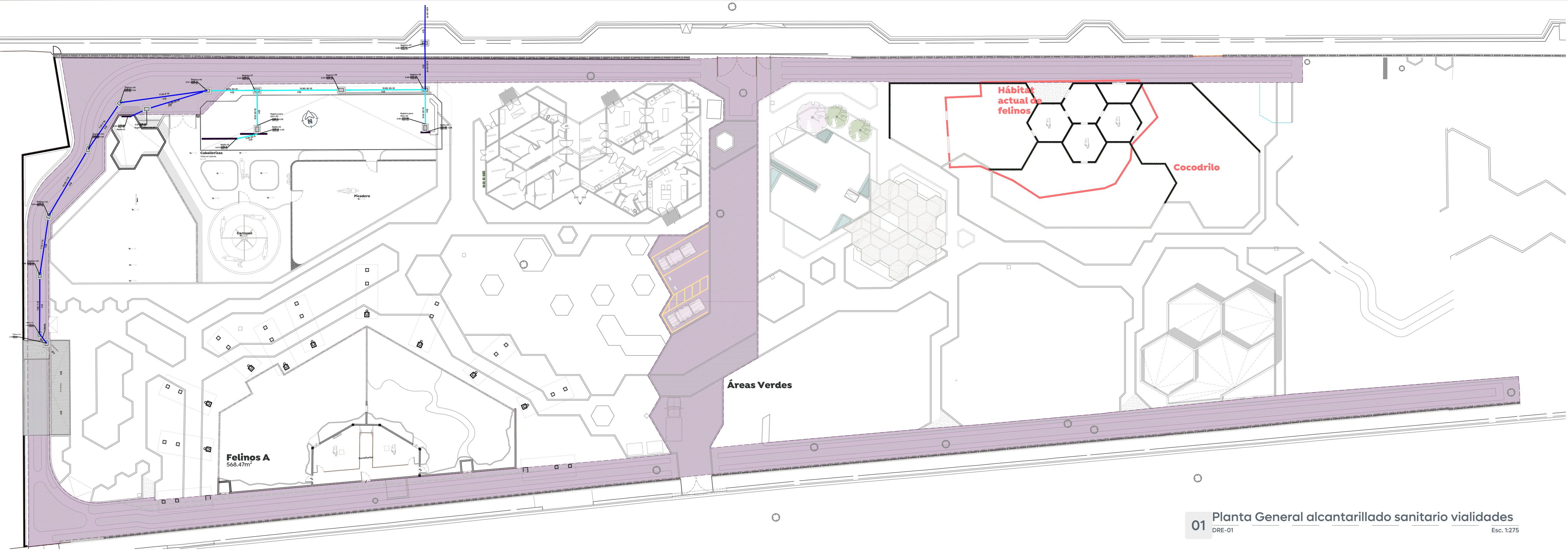
01 Planta de drenaje sanitario vialidades DRE-01 Esc. 1:125
