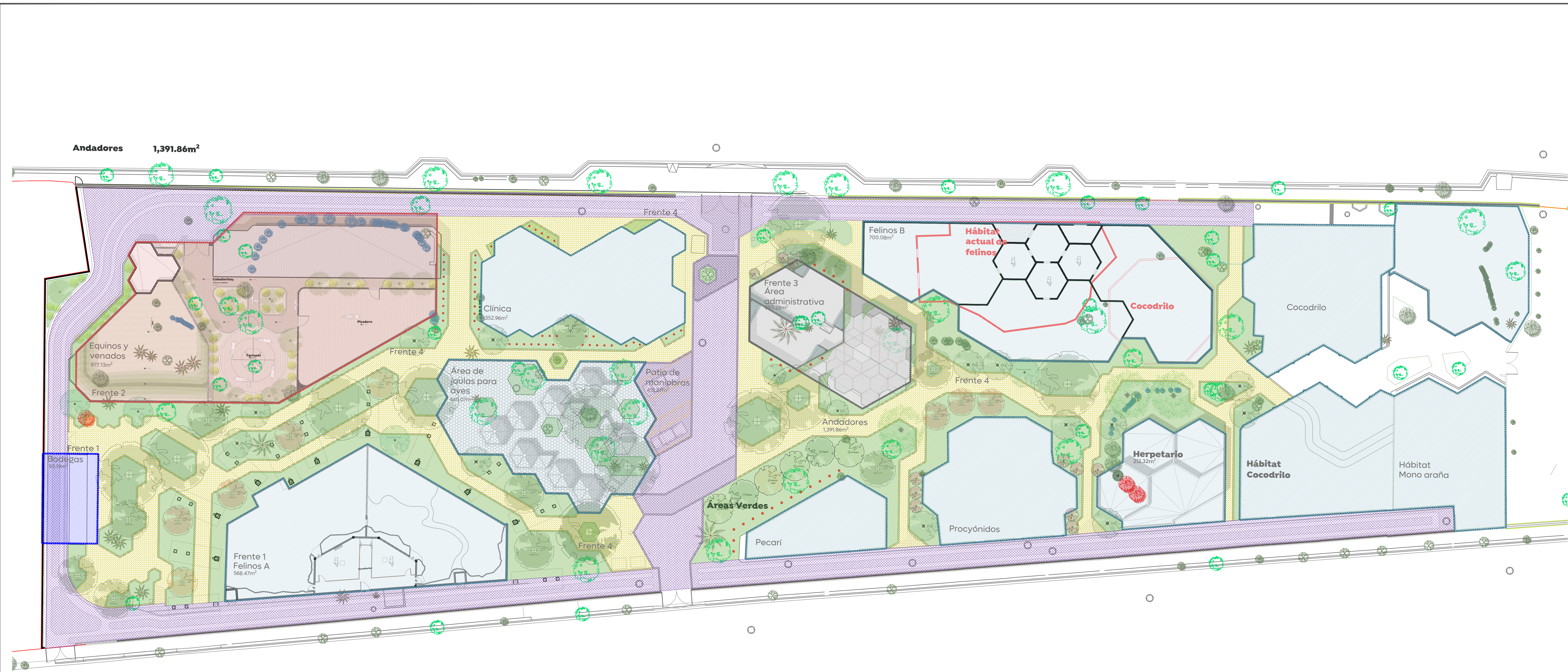
01 Planta frentes IE-00 Esc. 1:275
