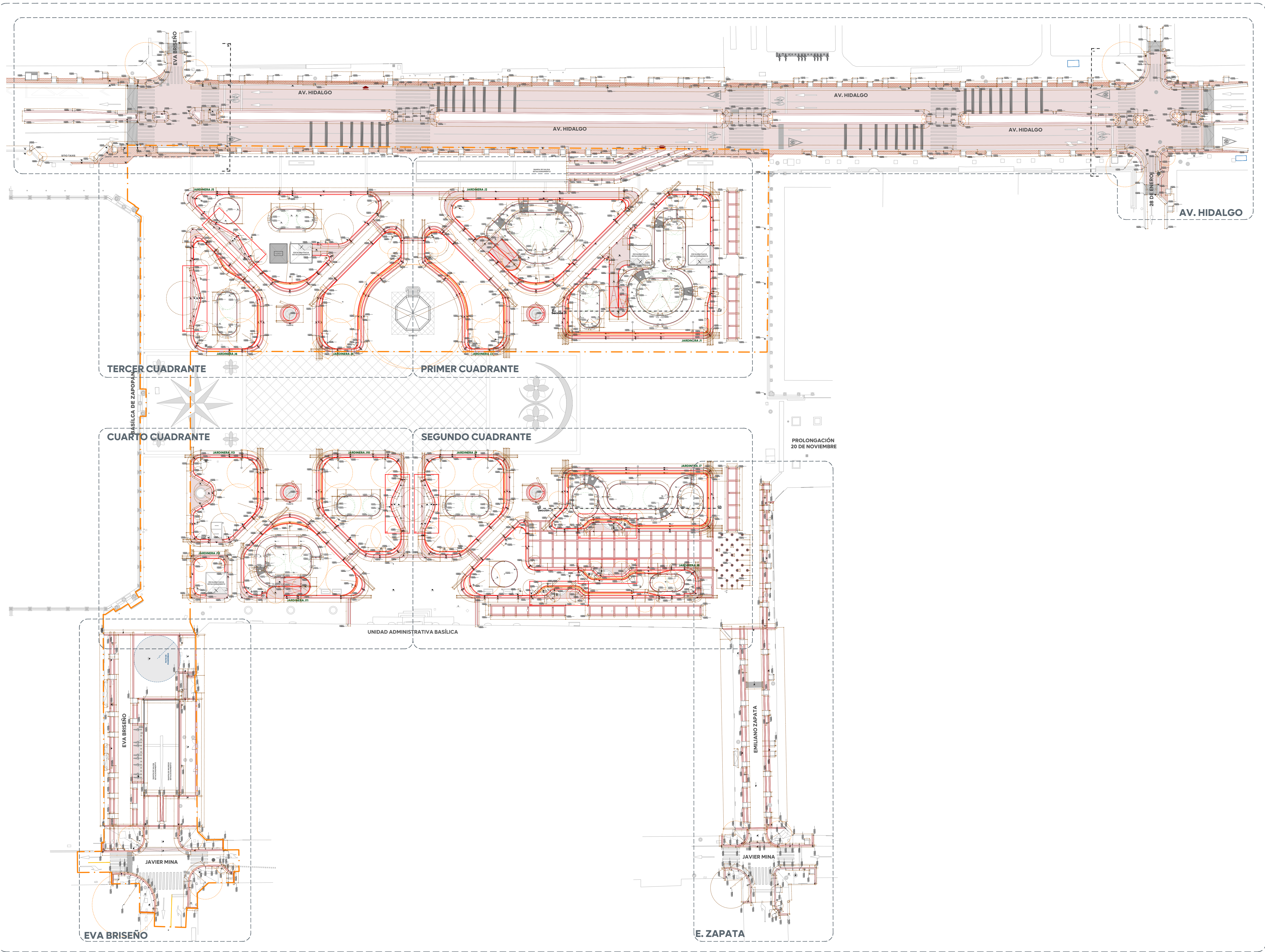
01 Plano Llave de Albañilerías 1:400
