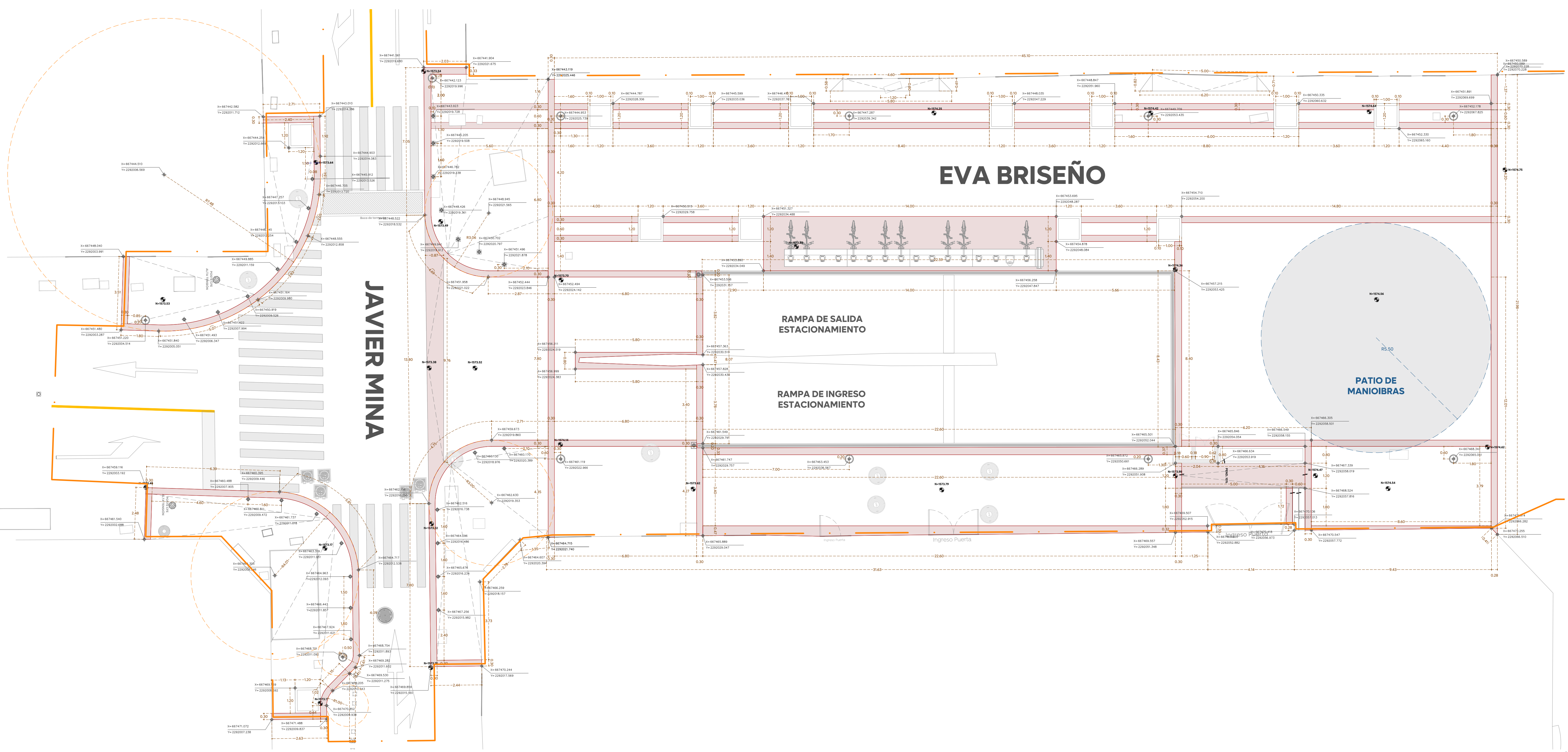
01 Plano de Albañilerías Andador Eva Briseño 1:100
